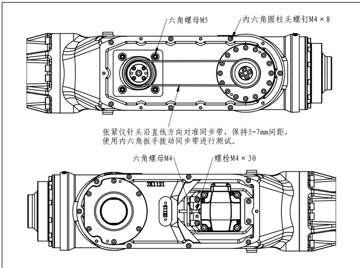
图 5.1 同步带张紧位置示意图
