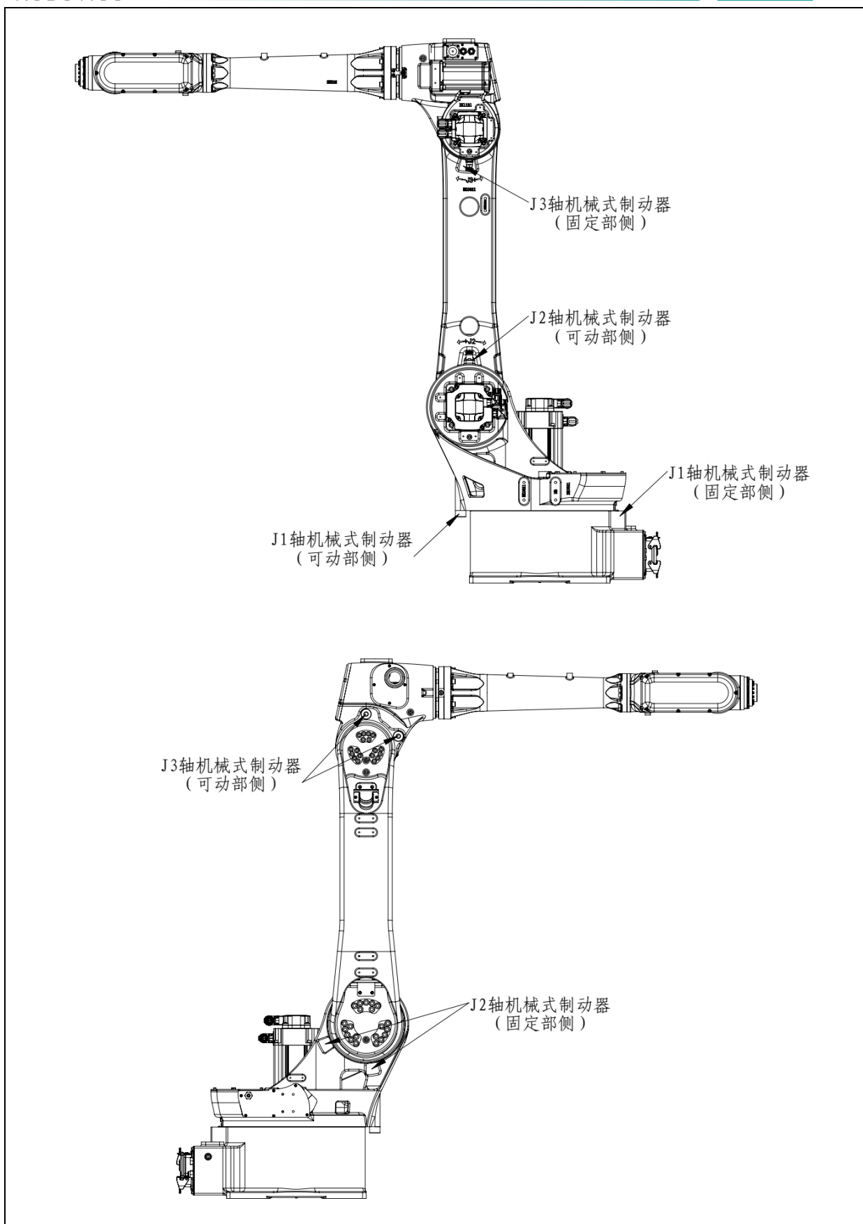
图 3.11 机械式制动器位置 (ER20B/10-2010-HI)
