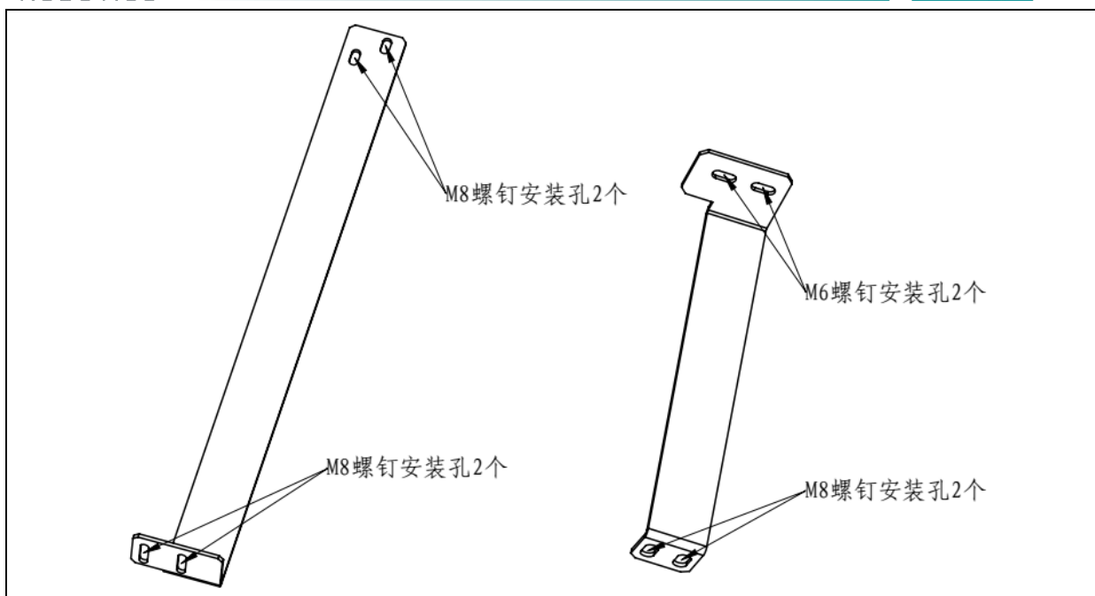
图 1.3 机器人固定支架示意图（ER20B-1760、ER20B-1760-HI）
