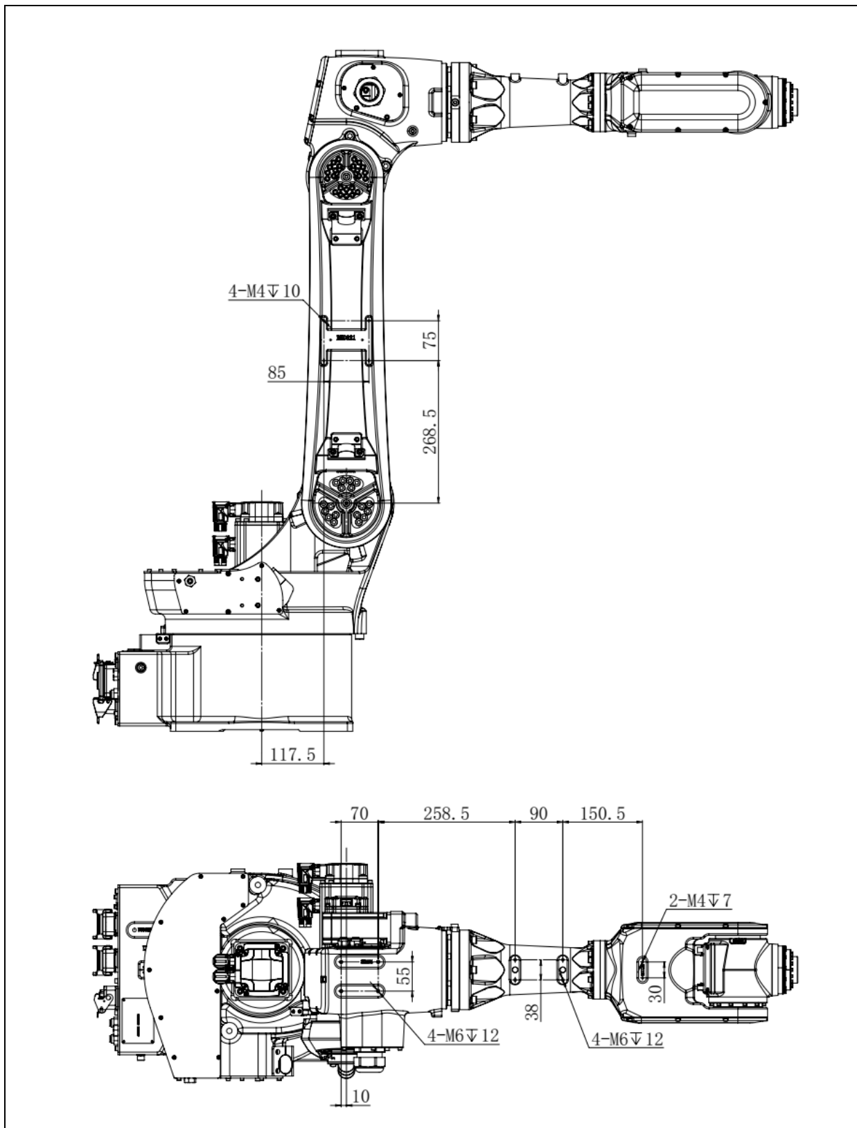
图 4.4 设备安装面尺寸 (ER12B-1510-LI、ER12B-1510)
