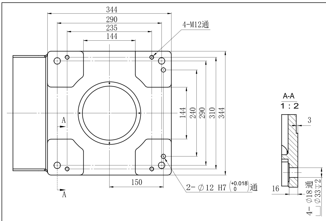
图 1.15 机器人底座安装尺寸 (ER12B-1510-LI、ER12B-1510)
