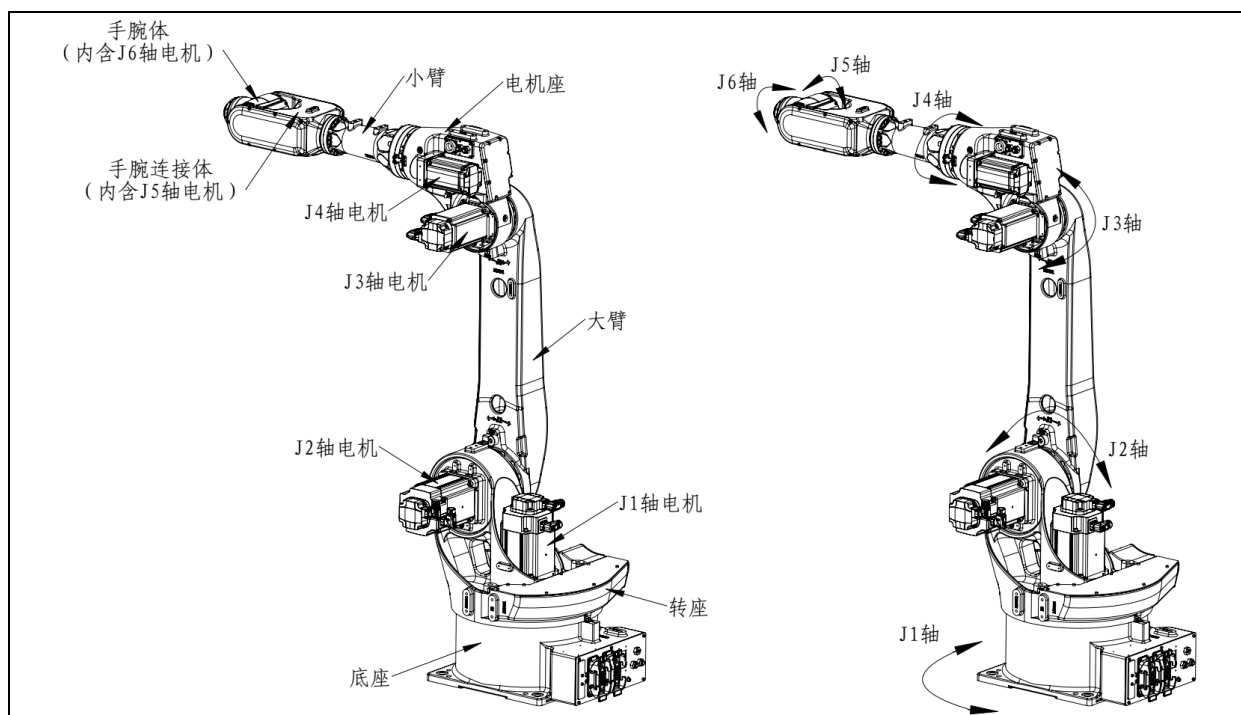
图 3.1 机器人的构成 (ER20B/10-2010-HI、ER20B-1760、ER20B-1760-HI、 ER35B-1810-LI、ER35B-1810)
