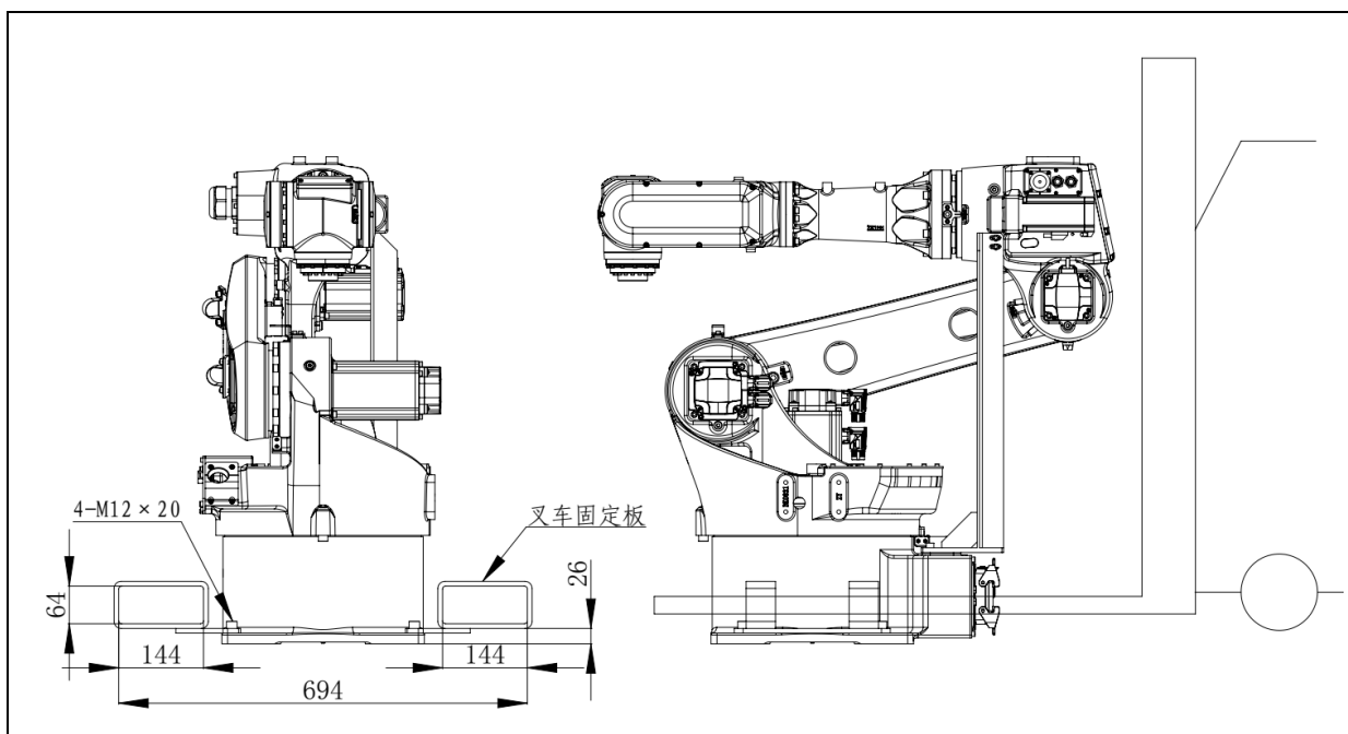
图 1.6 机器人叉车搬运示意图 (ER12B-1510-LI、ER12B-1510)
