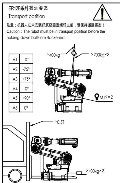
图 0.7 搬运标识 (ER12B-1510-LI、ER12B-1510)
