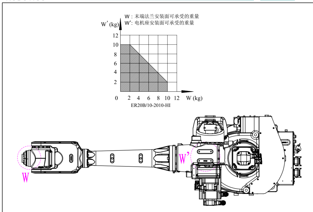
图 3.20 附加负载示意图(ER20B/10-2010-HI)
