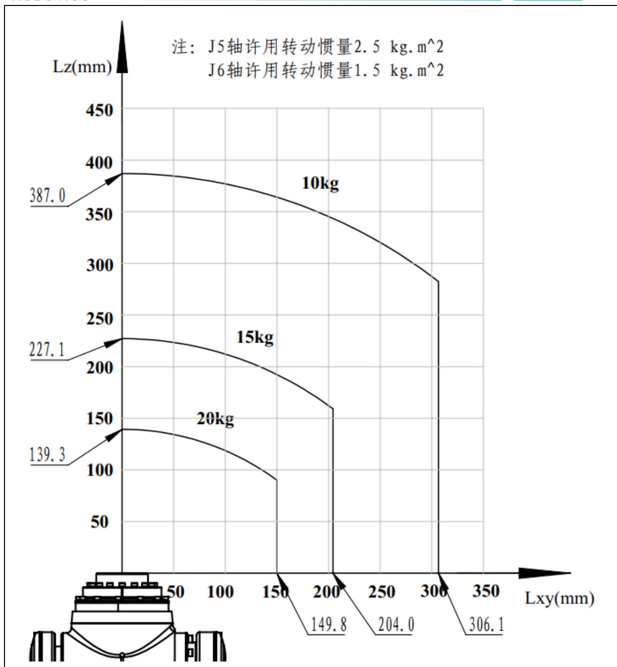
图 3.18 手腕部负载条件 (ER20B-1760-HI)
