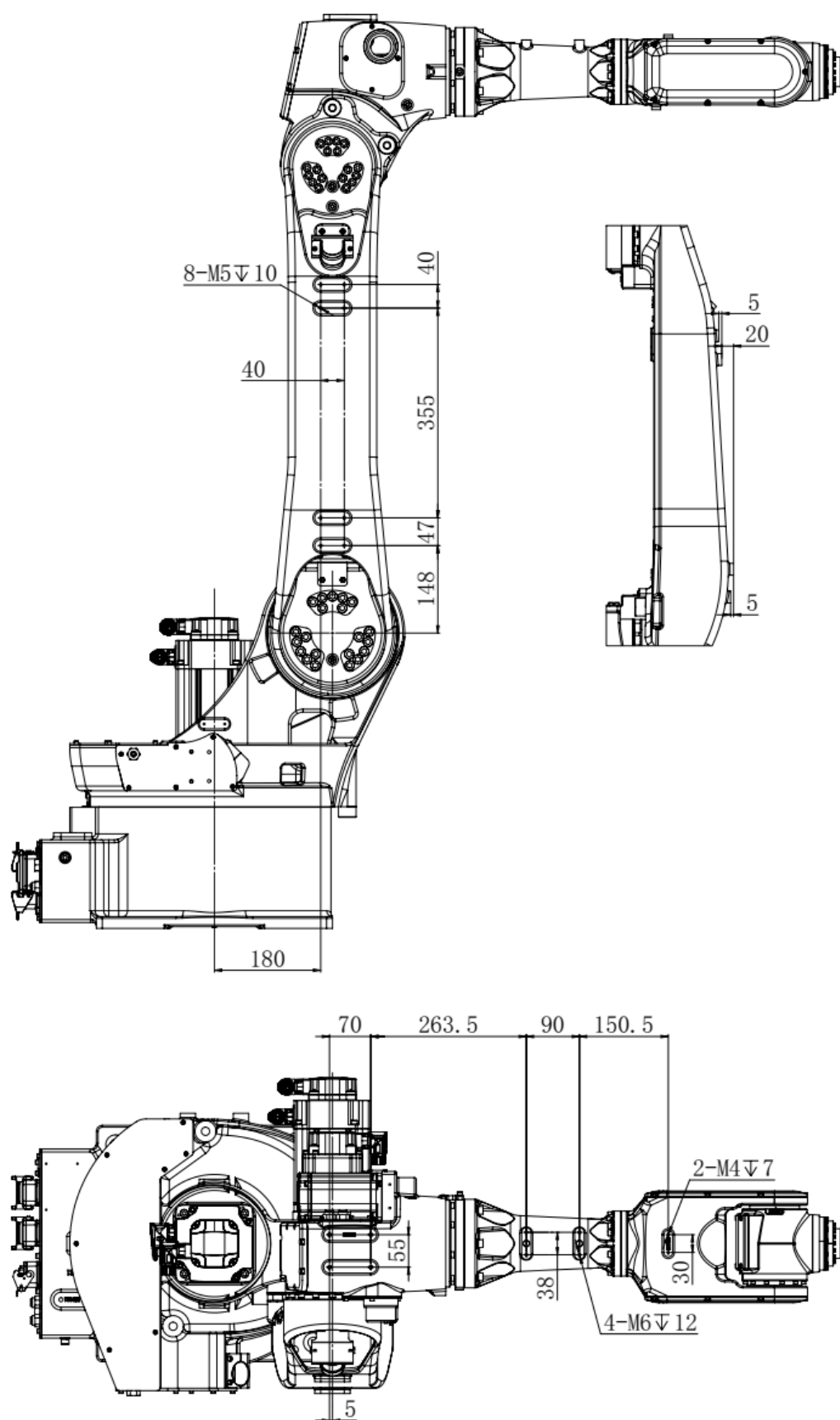
图 4.5 设备安装面尺寸 (ER20B-1760、ER20B-1760-HI)
