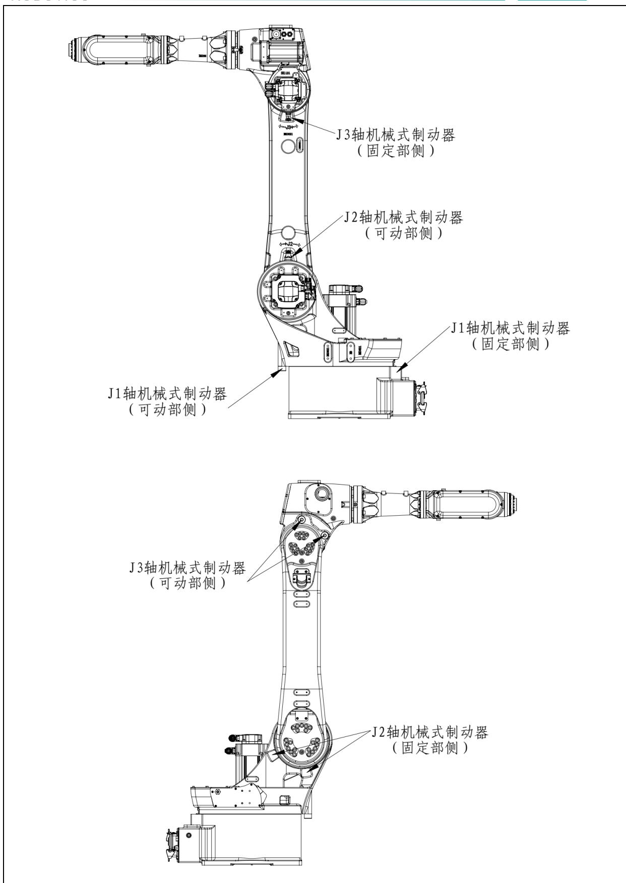
图 3.13 机械式制动器位置 (ER20B-1760、ER20B-1760-HI)
