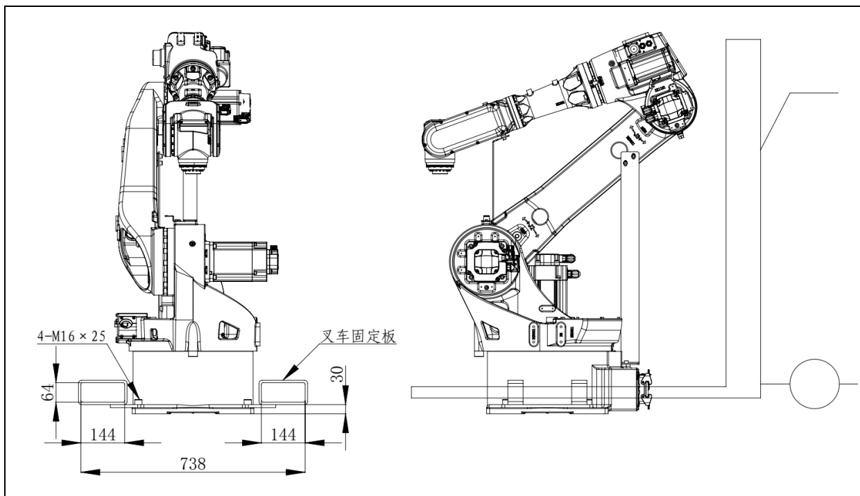
图 1.7 机器人叉车搬运示意图 (ER20B-1760、ER20B-1760-HI)
