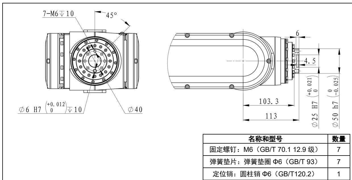
图 4.1 末端法兰安装接口 (ER20B/10-2010-HI、ER12B-1510-LI、ER12B-1510、ER20B-1760、ER20B-1760-HI)
