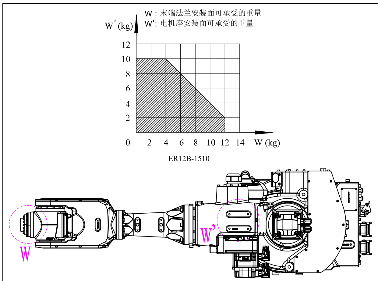
图 3.19 附加负载示意图(ER12B-1510-LI、ER12B-1510)
