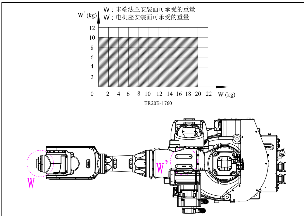
图 3.20 附加负载示意图(ER20B-1760)
