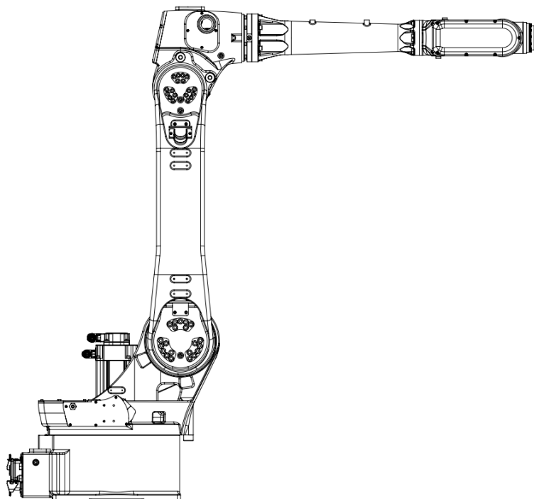
图 3.7 机器人的原点位置姿态 (ER20B/10-2010-HI)
