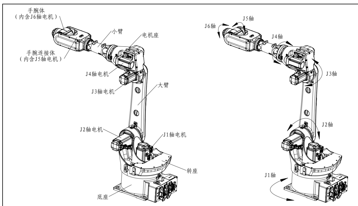
图 3.2 机器人的构成 (ER12B-1510-LI、ER12B-1510)
