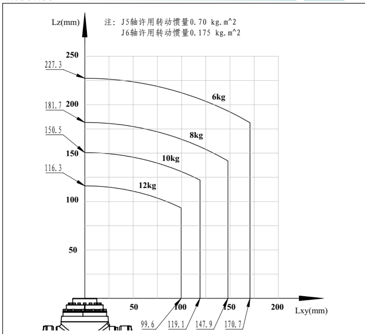
图 3.16 手腕部负载条件 (ER12B-1510-LI、ER12B-1510)
