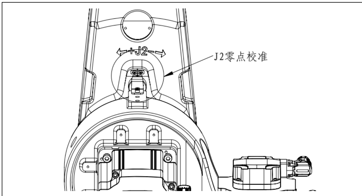
图 6.3 J2 轴校准示意图
