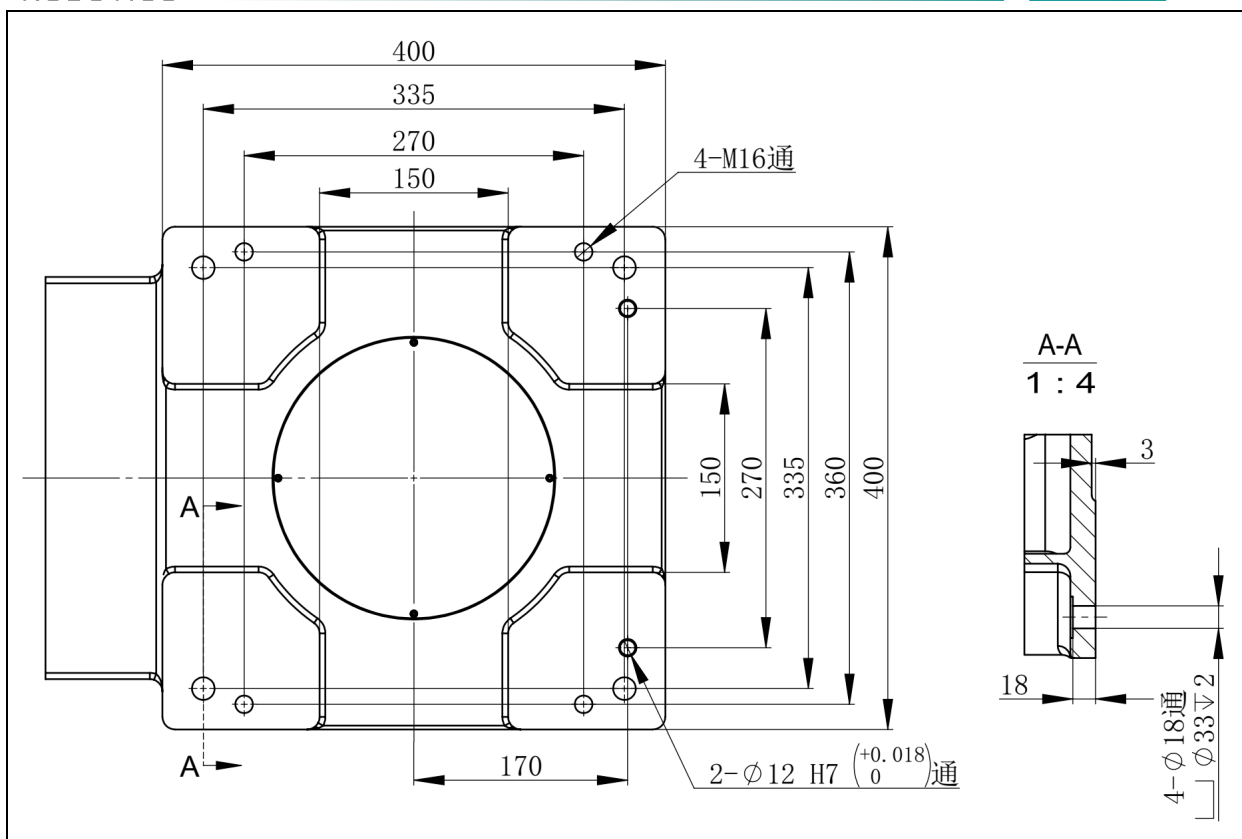
图 1.14 机器人底座安装尺寸 (ER20B/10-2010-HI、ER20B-1760、ER20B-1760-HI、 ER35B-1810-LI、ER35B-1810)
