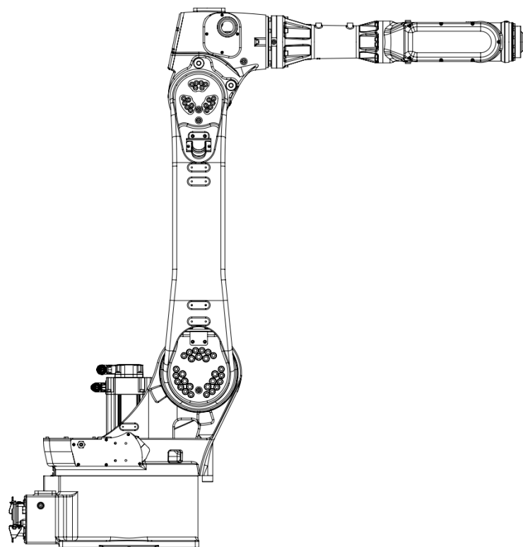
图 3.10 机器人的原点位置姿态 (ER35B-1810-LI、ER35B-1810)
