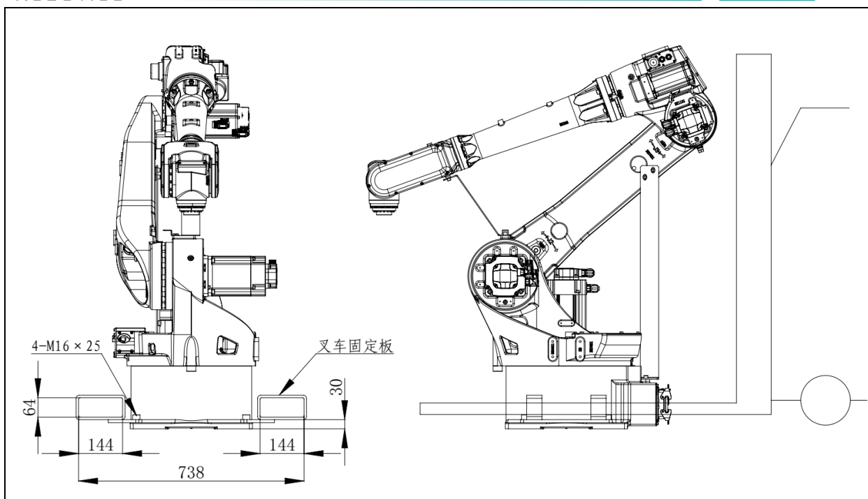
图 1.5 机器人叉车搬运示意图 (ER20B/10-2010-HI)
