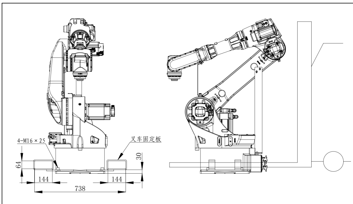
图 1.8 机器人叉车搬运示意图 (ER35B-1810-LI、ER35B-1810)
