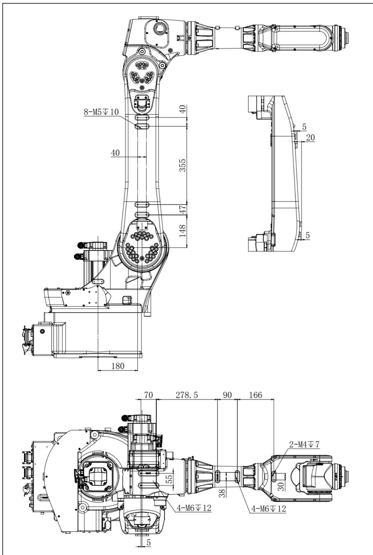
图 4.6 设备安装面尺寸 (ER35B-1810-LI、ER35B-1810)
