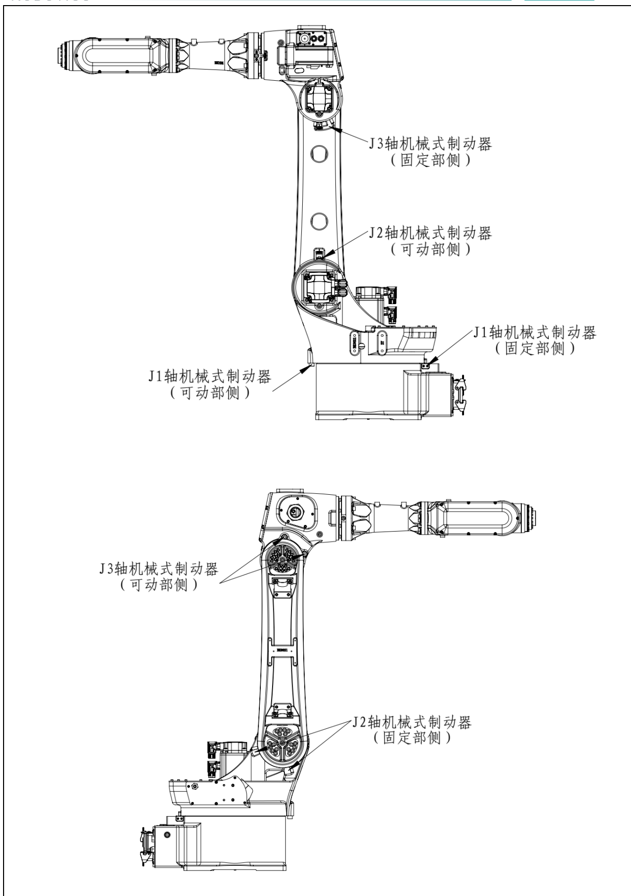
图 3.12 机械式制动器位置 (ER12B-1510-LI、ER12B-1510)
