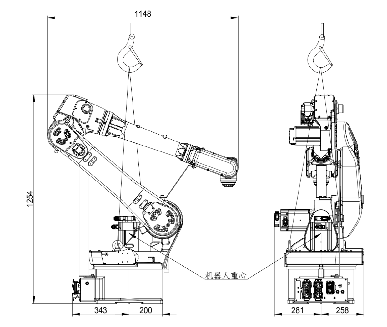
图 1.9 机器人起重机搬运示意图 (ER20B/10-2010-HI)
