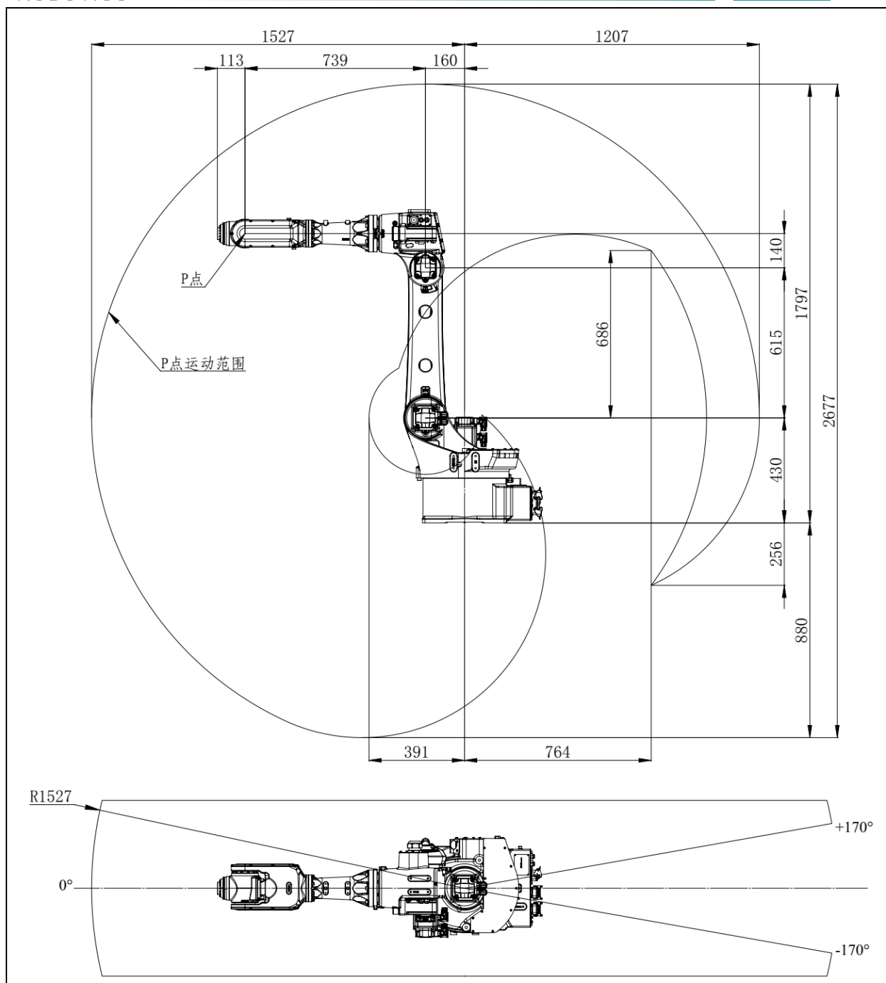
图 3.4 动作范围图 (ER12B-1510-LI、ER12B-1510)
