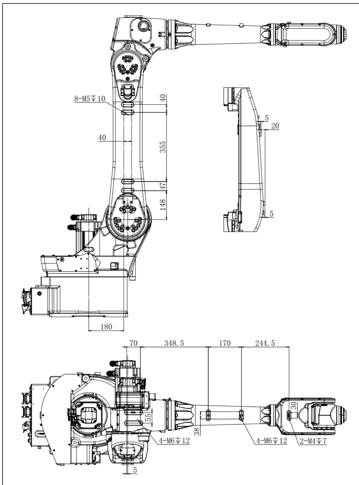
图 4.3 设备安装面尺寸 (ER20B/10-2010-HI)
