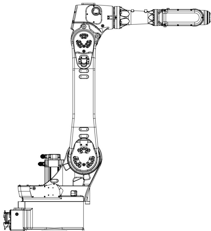
图 3.9 机器人的原点位置姿态 (ER20B-1760、ER20B-1760-HI)
