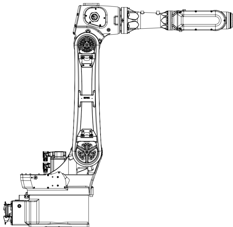
图 3.8 机器人的原点位置姿态 (ER12B-1510-LI、ER12B-1510)
