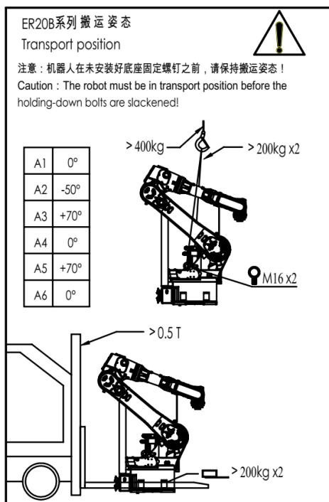
图 0.6 搬运标识（ER20B/10-2010-HI、ER20B-1760、ER20B-1760-HI、ER35B-1810-LI、 ER35B-1810）
