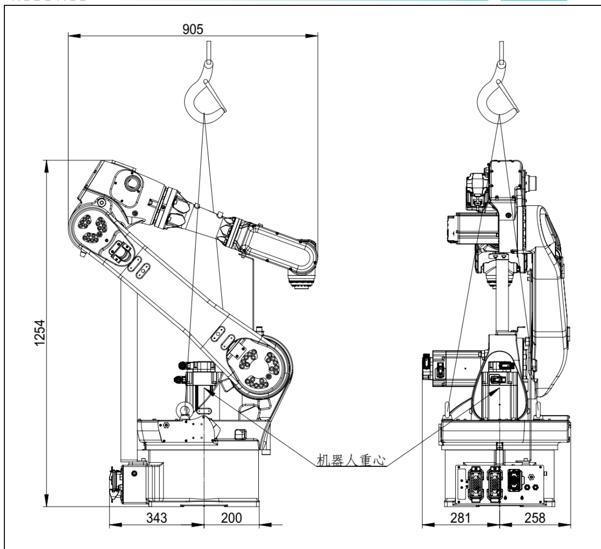
图 1.11 机器人起重机搬运示意图 (ER20B-1760、ER20B-1760-HI)
