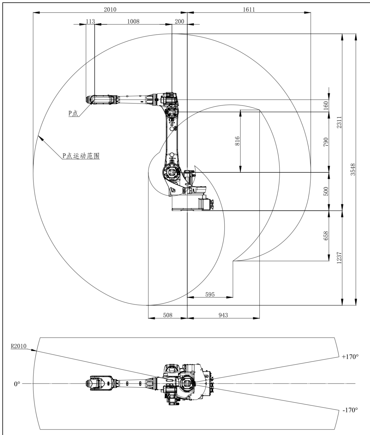
图 3.3 动作范围图 (ER20B/10-2010-HI)
