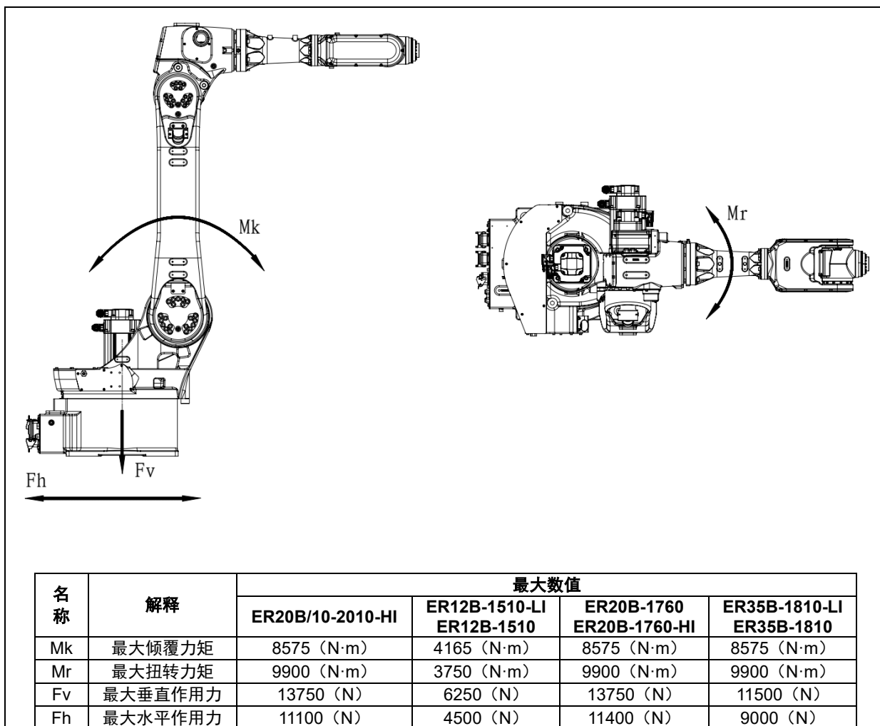
图 1.13 机器人底座受力数据
