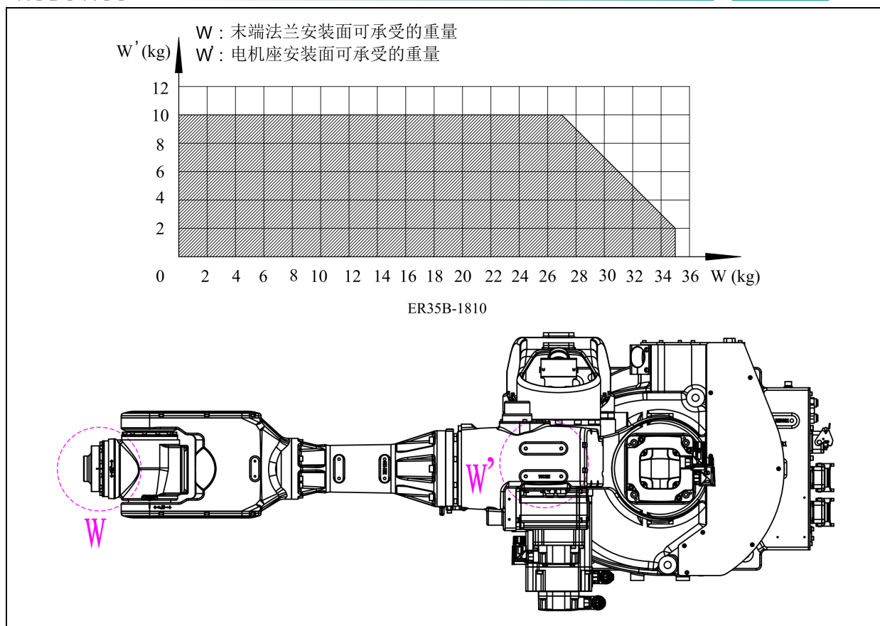
图 3.21 附加负载示意图(ER35B-1810-LI、ER35B-1810)
