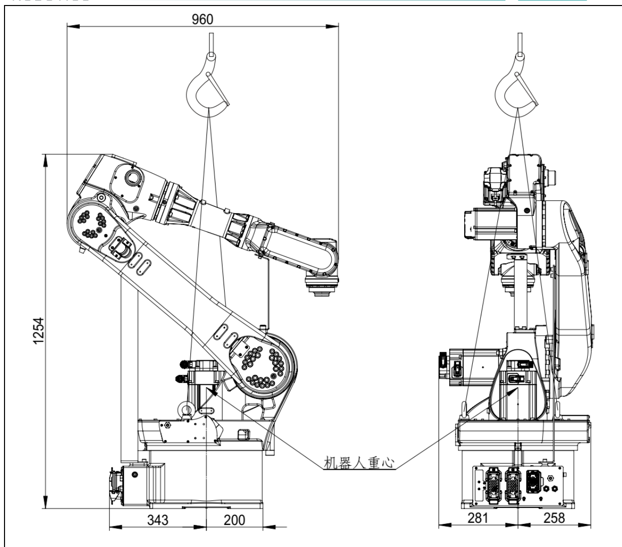
图 1.12 机器人起重机搬运示意图 (ER35B-1810-LI、ER35B-1810)
