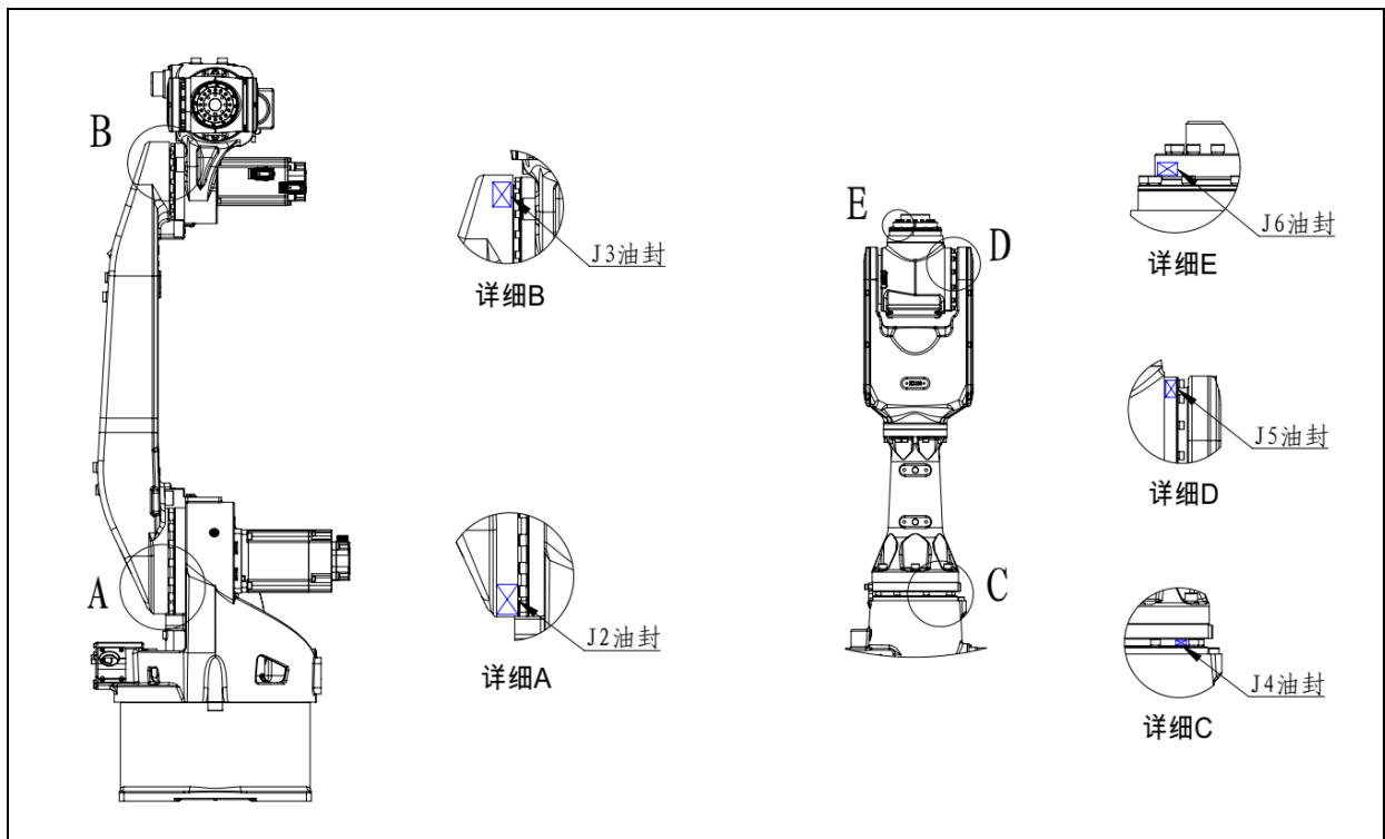
图 5.7 油封的检查部位
