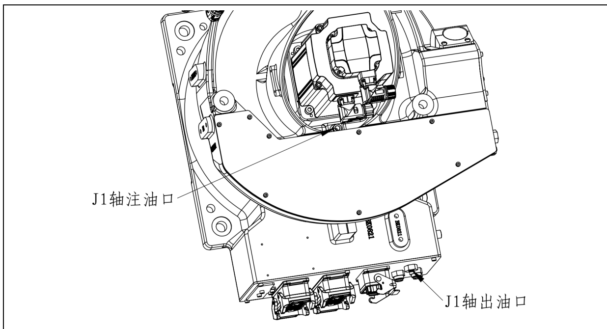
图 5.3 J1 轴注油、出油口
