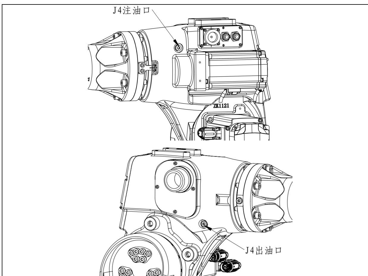
图 5.6 J4 轴注油、出油口
