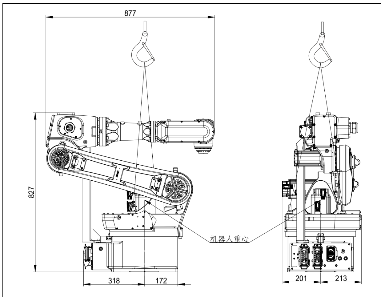
图 1.10 机器人起重机搬运示意图 (ER12B-1510-LI、ER12B-1510)
