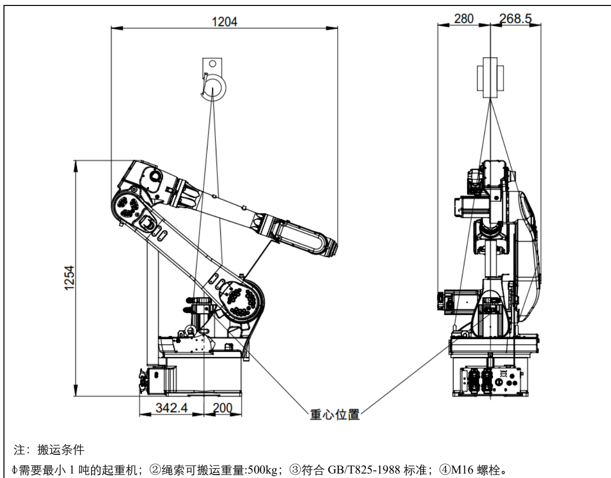
图 1-7 机器人起重机搬运示意图 (ER8-2000-CW)
