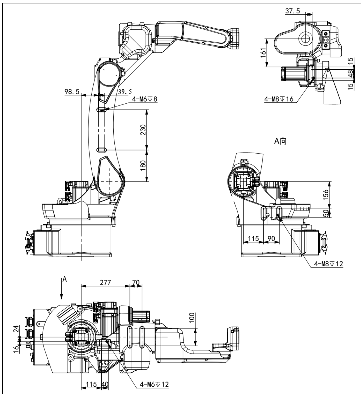
图 4-5 设备安装面尺寸 (ER8-1450-HW)
