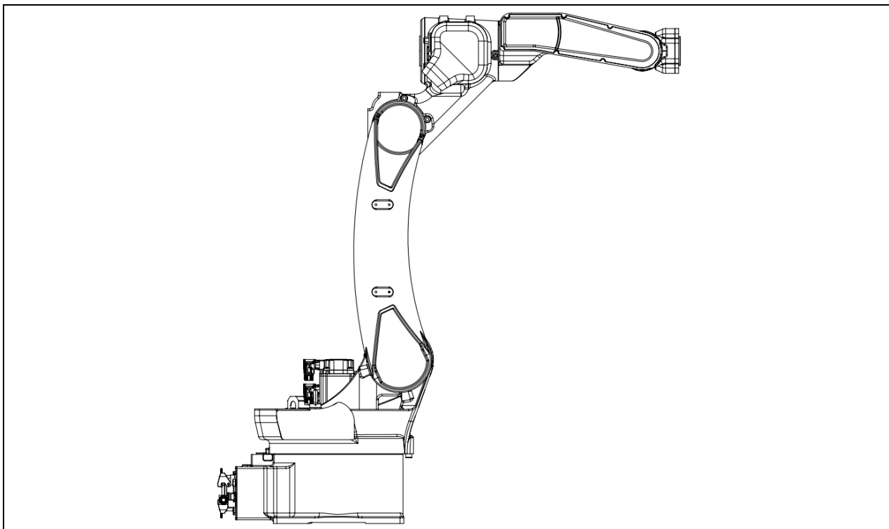
图 3-9 机器人的原点位置姿态（ER8-1450-HW）
