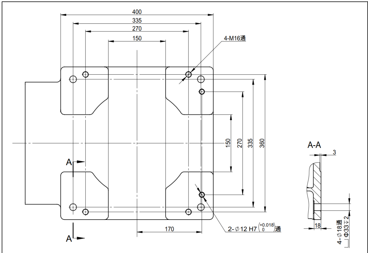
图 1-14 机器人底座安装尺寸 (ER8-2000-CW、ER8-2000-HW)
