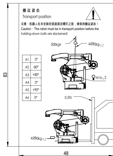
图 0-9 ER8-2000-HW 搬运标识
