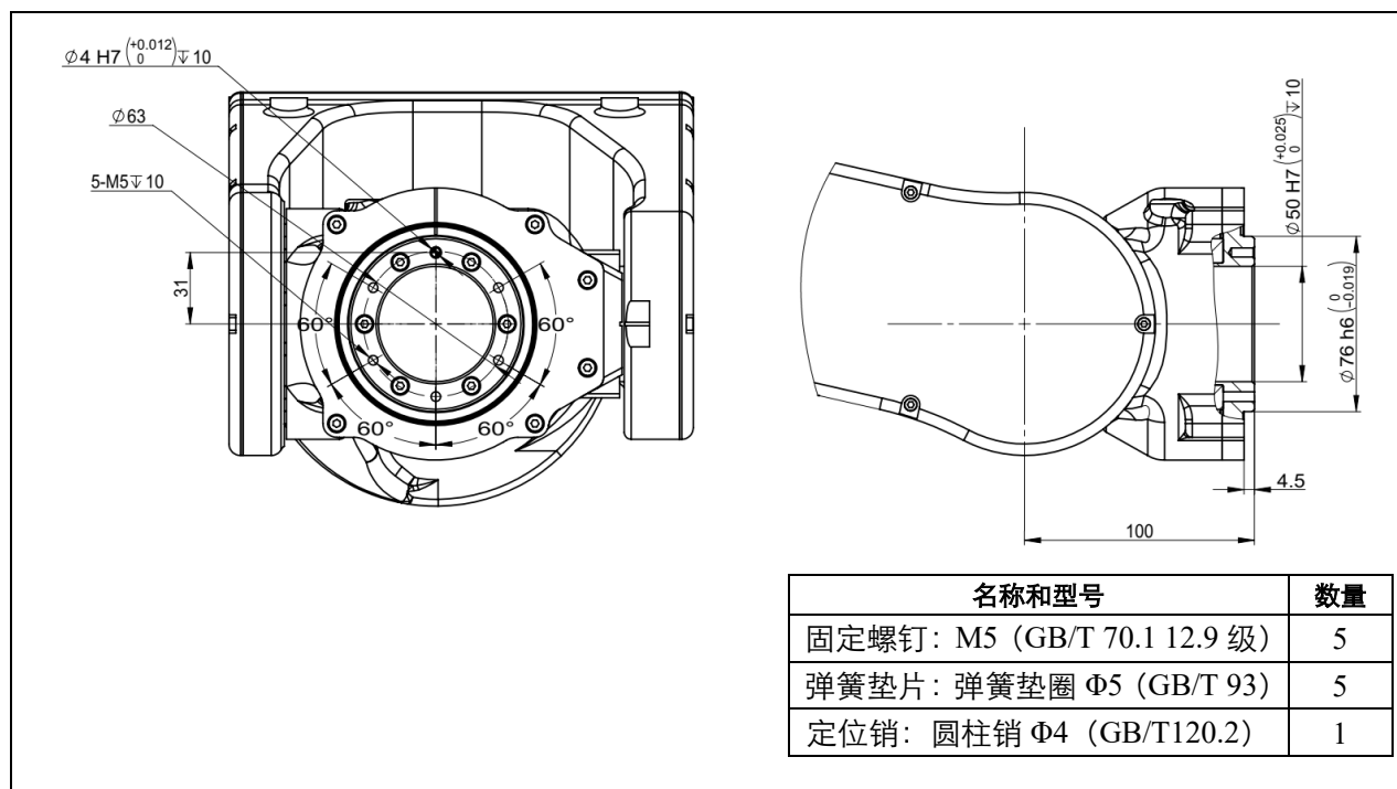
图 4-4 末端法兰安装接口 (ER8-2000-HW)
