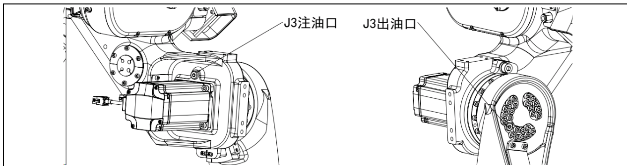
图 5-11J3 轴注油、出油口 (ER8-1450-HW)
