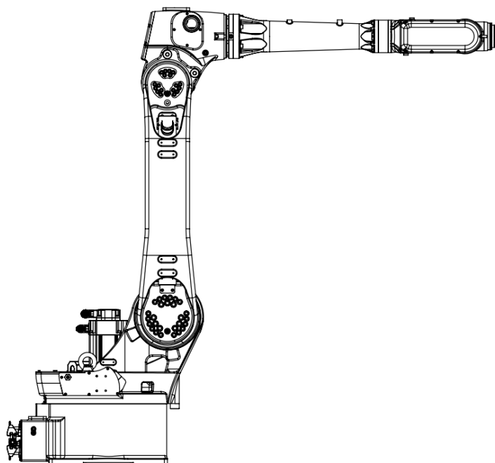
图 3-11 机器人的原点位置姿态 (ER8-2000-CW)
