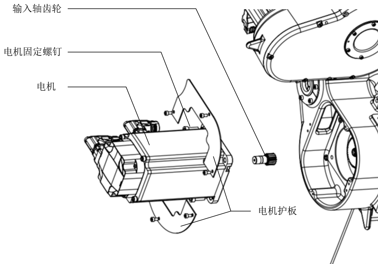
ER8-2000-HW 电机安装爆炸图
