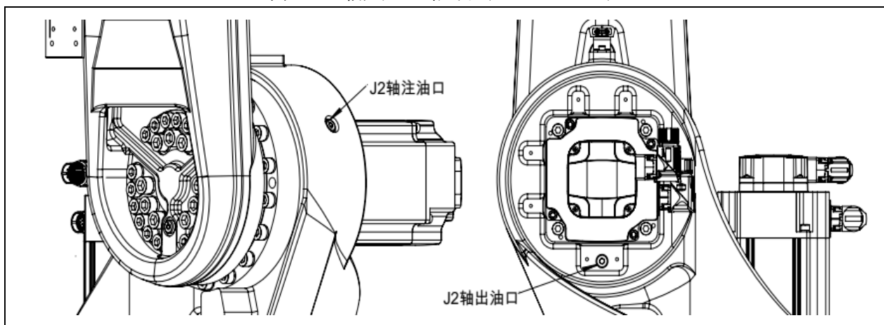
图 5-9J2 轴注油、出油口 (ER8-2000-HW)
