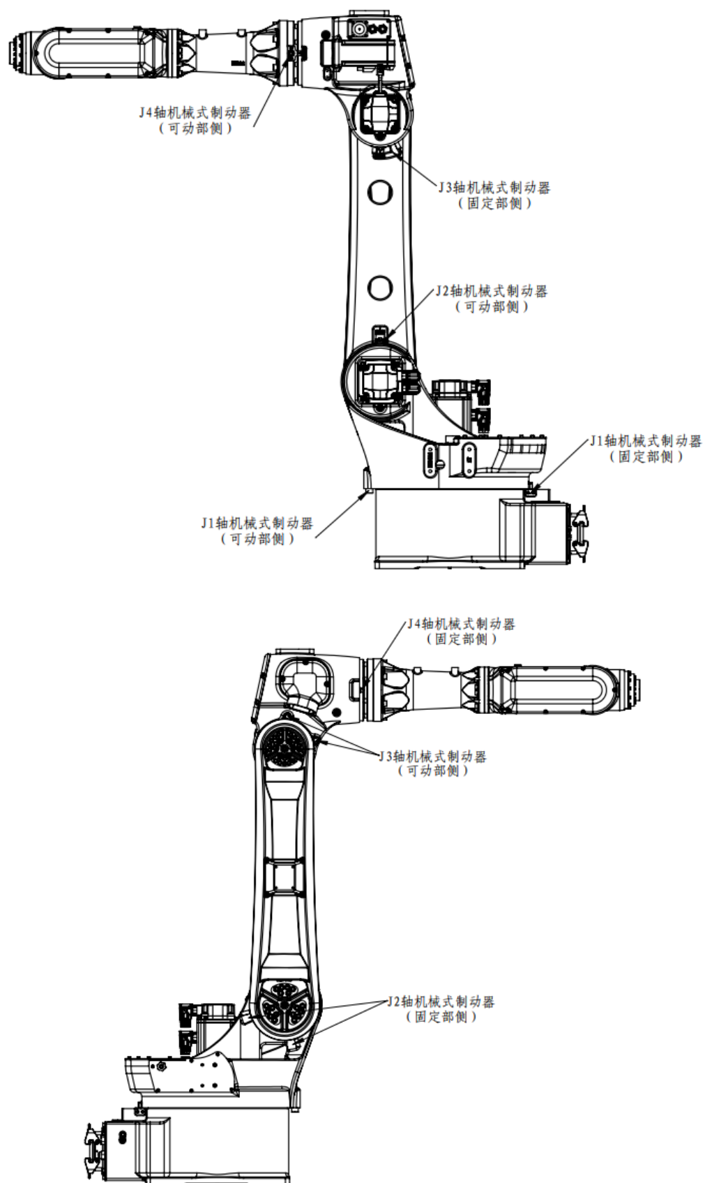
图 3-14 机械式制动器位置 (ER8-1500-CW)
