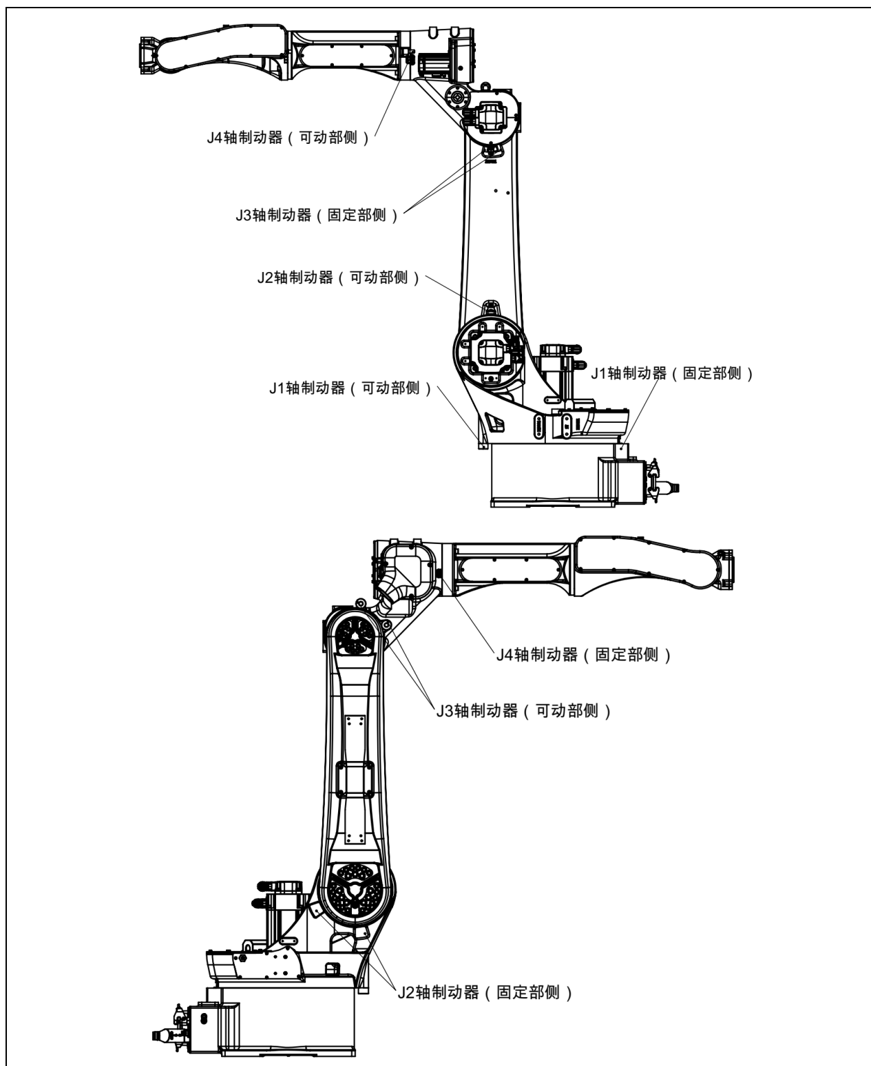
图 3-16 机械式制动器位置 (ER8-2000-HW)
