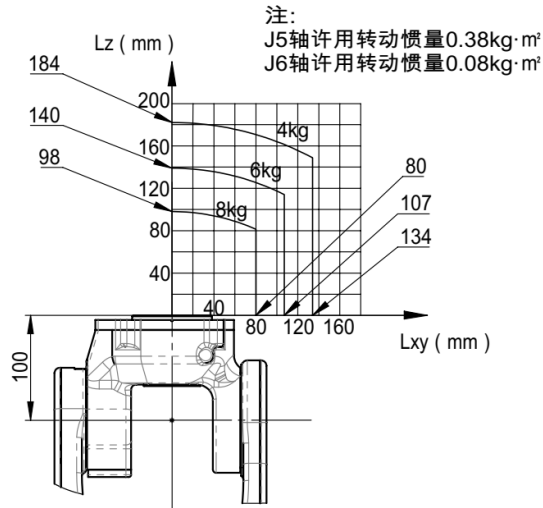
图 3-20 手腕部负载条件 (ER8-2000-HW)
