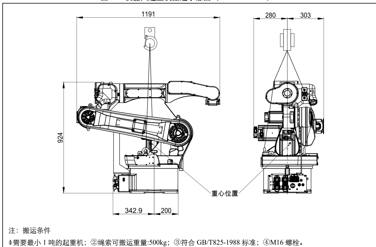
图 1-8 机器人起重机搬运示意图 (ER8-2000-HW)
