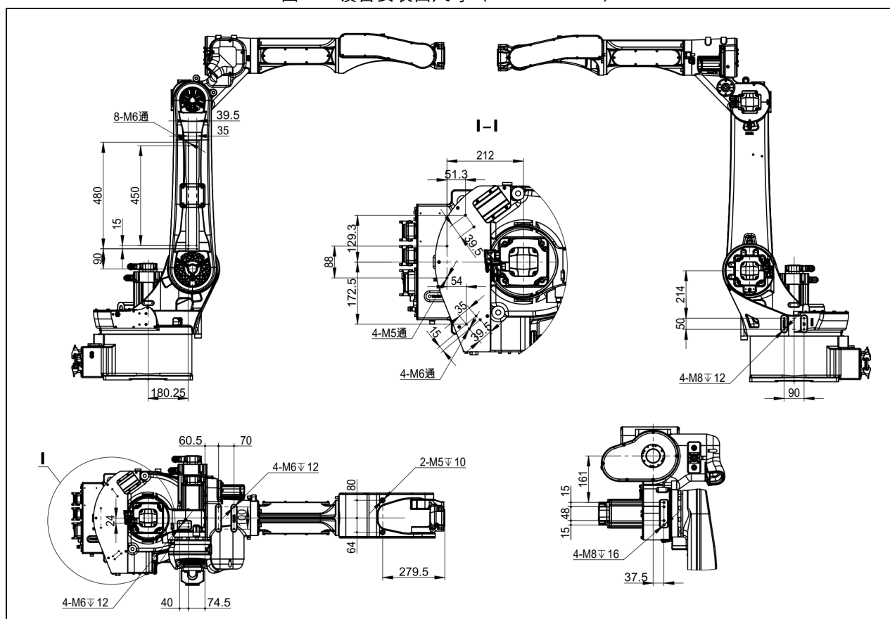
图 4-8 设备安装面尺寸 (ER8-2000-HW)
