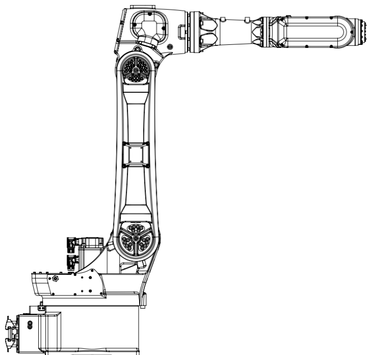
图 3-10 机器人的原点位置姿态 (ER8-1500-CW)
