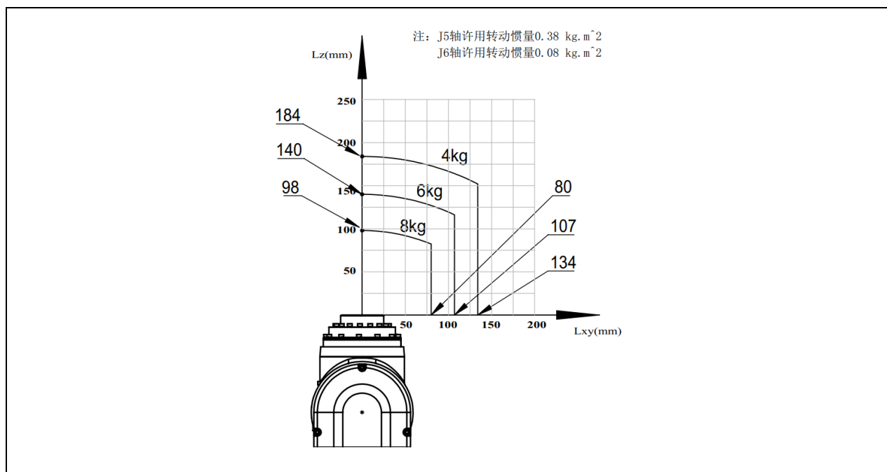
图 3-18 手腕部负载条件 (ER8-1500-CW)
