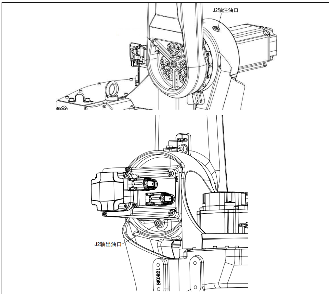
图 5-8J2 轴注油、出油口 (ER8-1500-CW)
