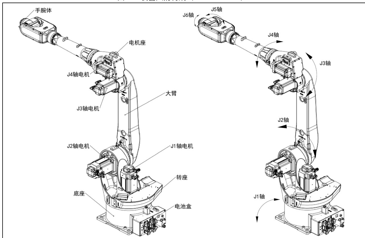
图 3-4 机器人的构成 (ER8-2000-CW)
