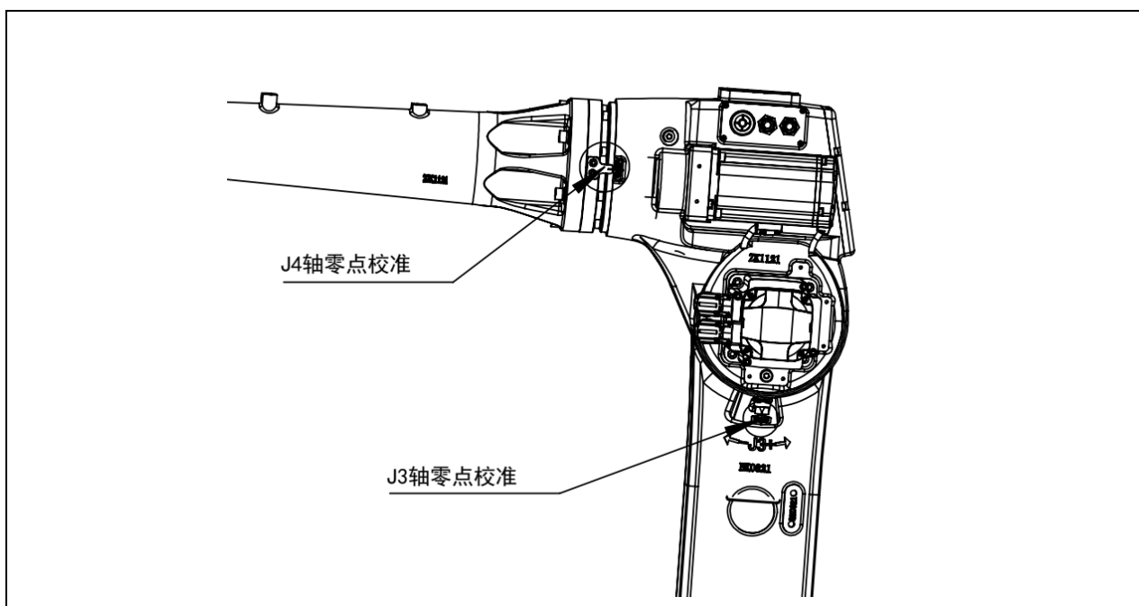
图 6-9 J3、J4 轴校准示意图 (ER8-2000-CW)
