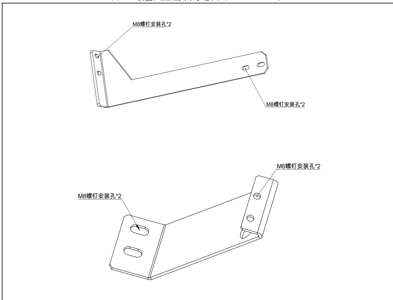
图 1-4 机器人固定支架示意图 (ER8-2000-HW)
