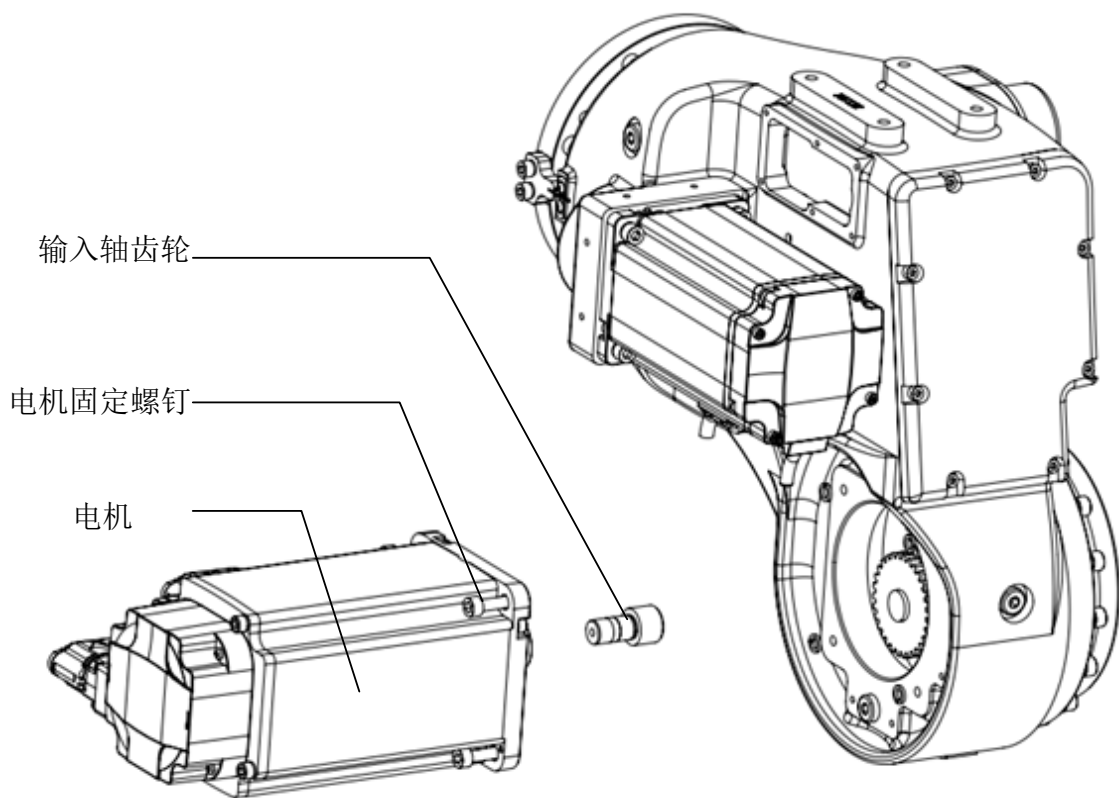
ER8-2000-CW 电机安装爆炸图
