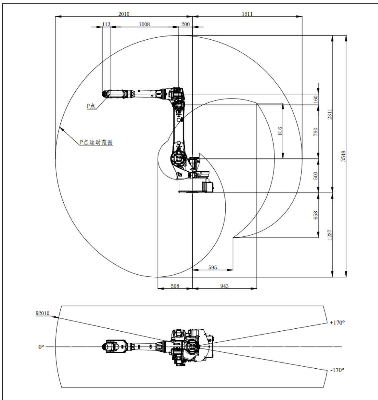
图 3-7 动作范围图 (ER8-2000-CW)
