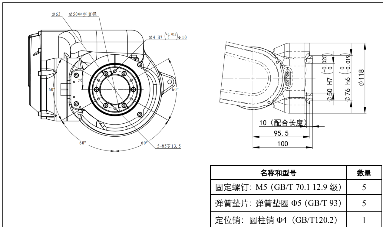
图 4-1 末端法兰安装接口 (ER8-1450-HW)
