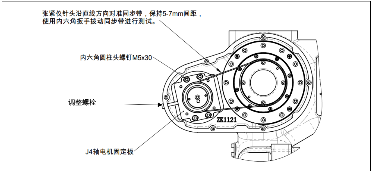
图 5-1J4 轴同步带张紧位置示意图 (ER8-1450-HW、ER8-2000-HW)
