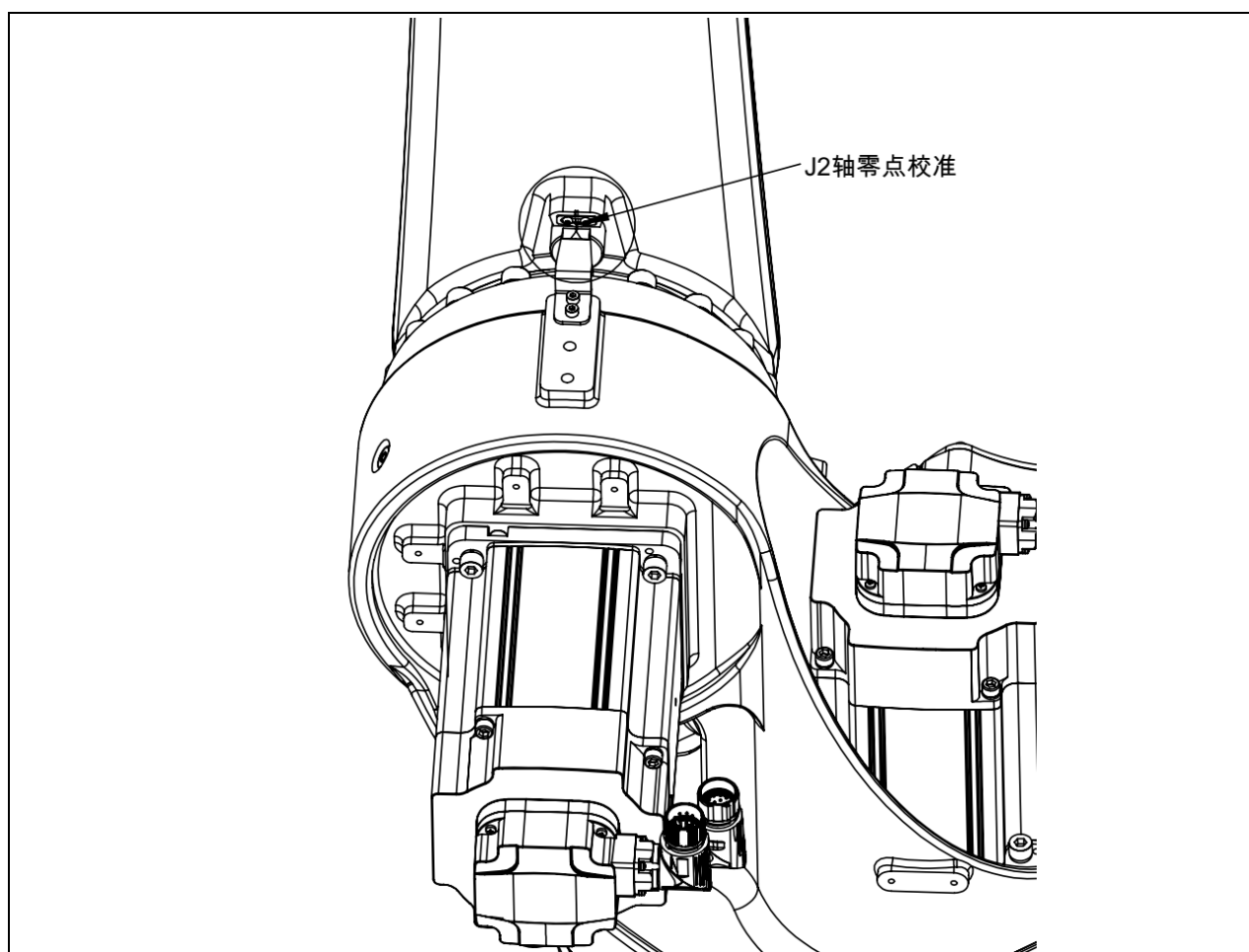
图 6-4 J2 轴校准示意图 (ER8-1500-CW、ER8-2000-CW、ER8-2000-HW)
