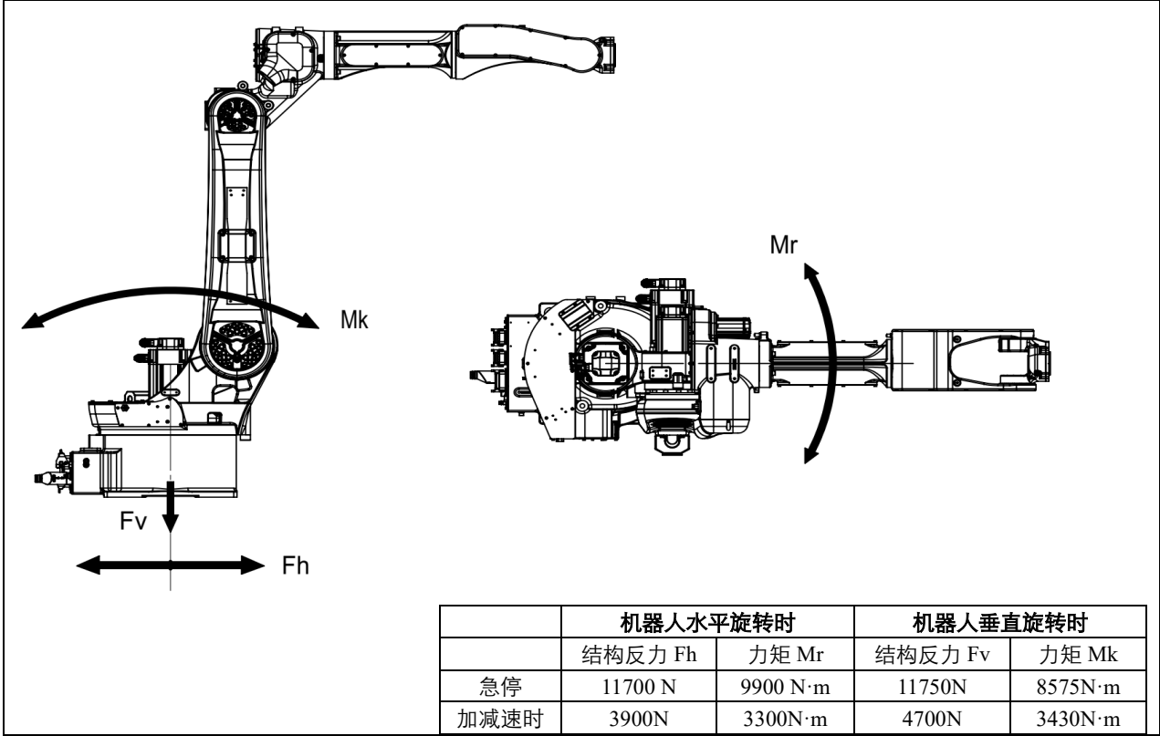
图 1-12 机器人底座受力数据 (ER8-2000-HW)
