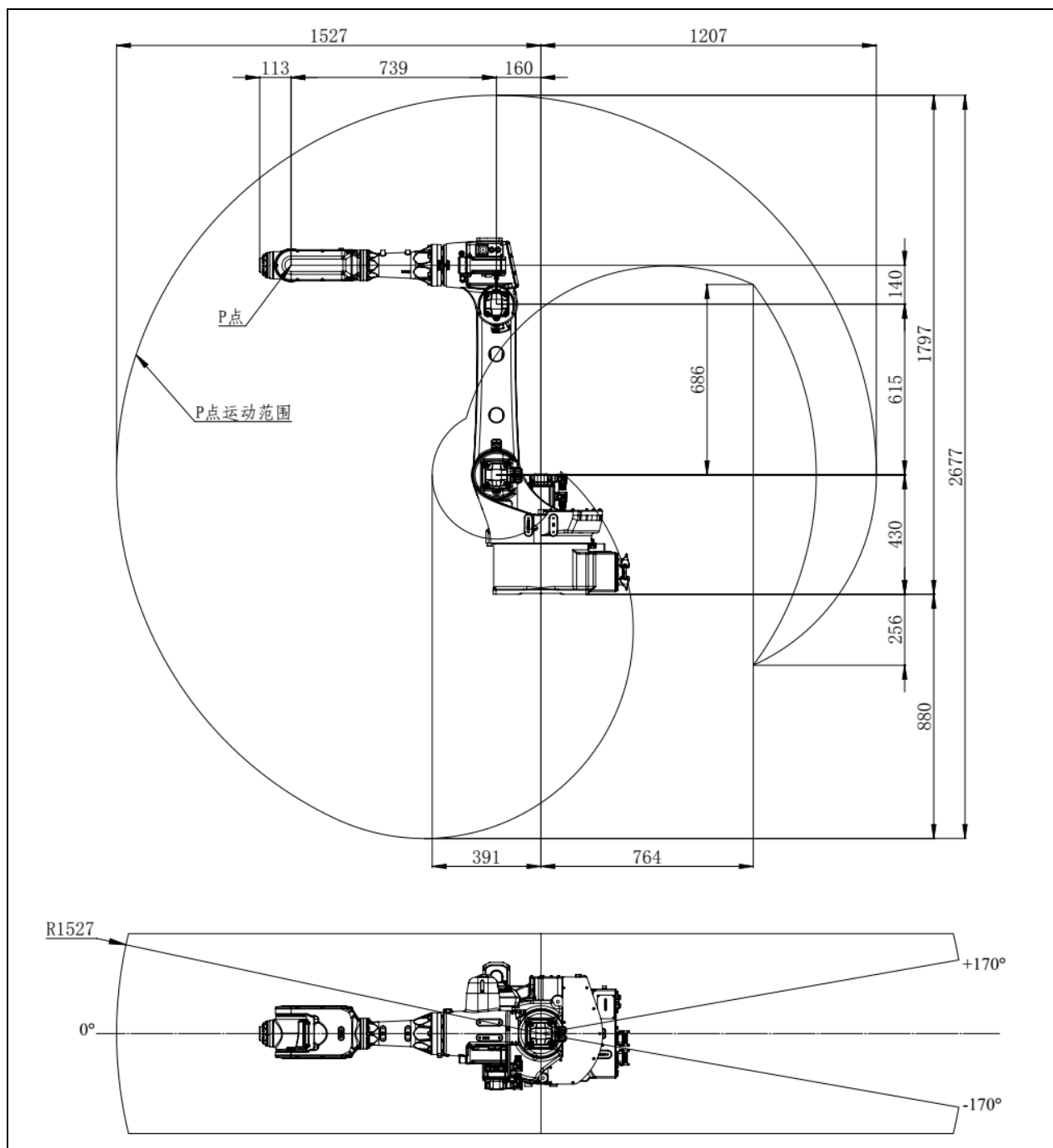
图 3-6 动作范围图 (ER8-1500-CW)
