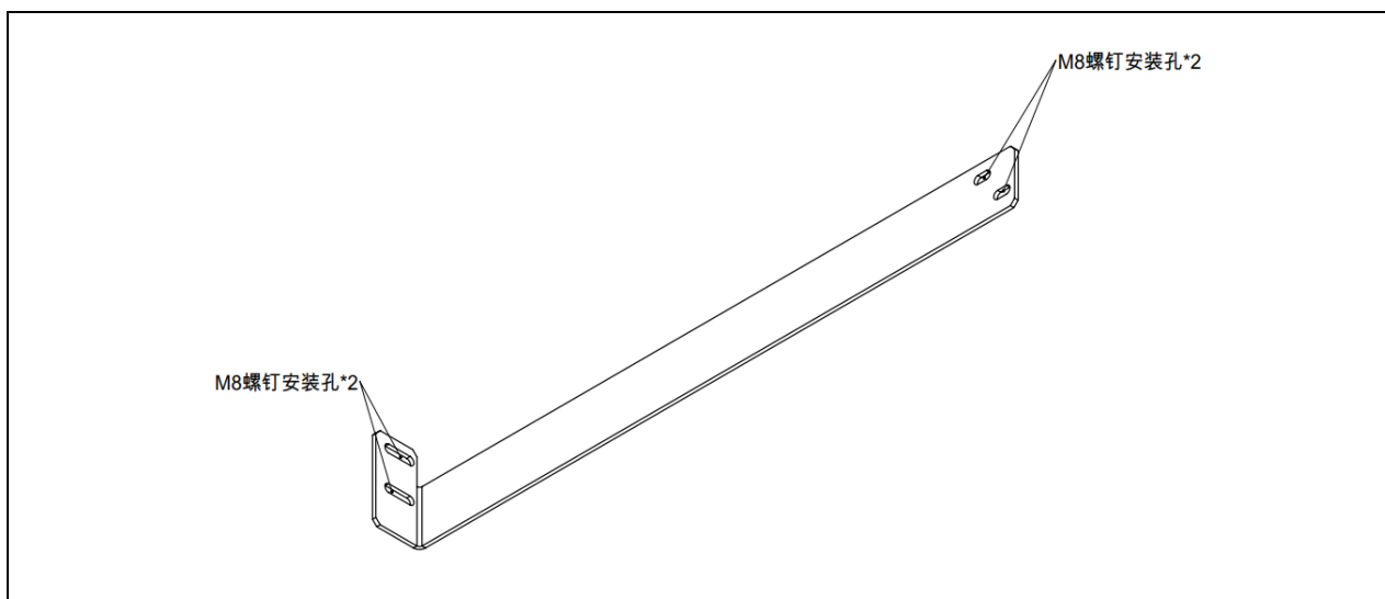
图 1-2 机器人固定支架示意图 (ER8-1500-CW)
