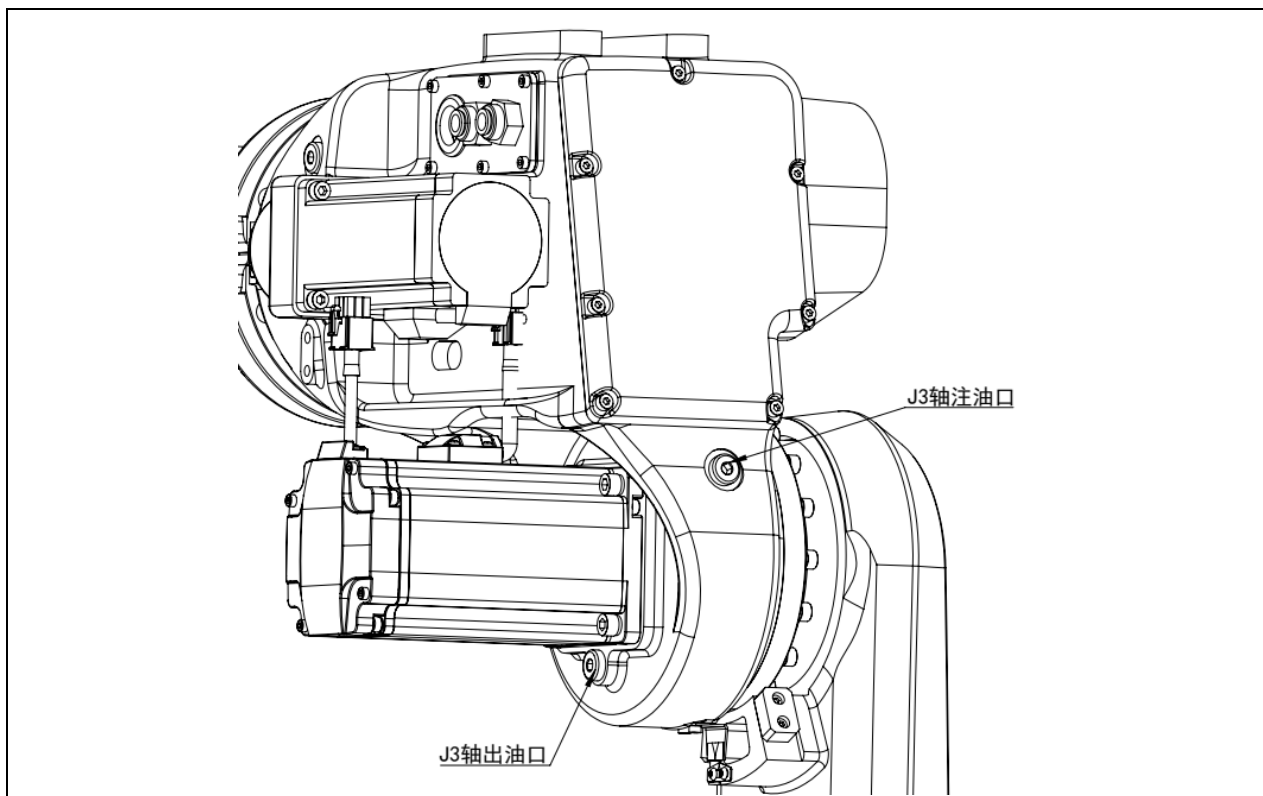
图 5-14J3 轴注油、出油口 (ER8-2000-CW)
