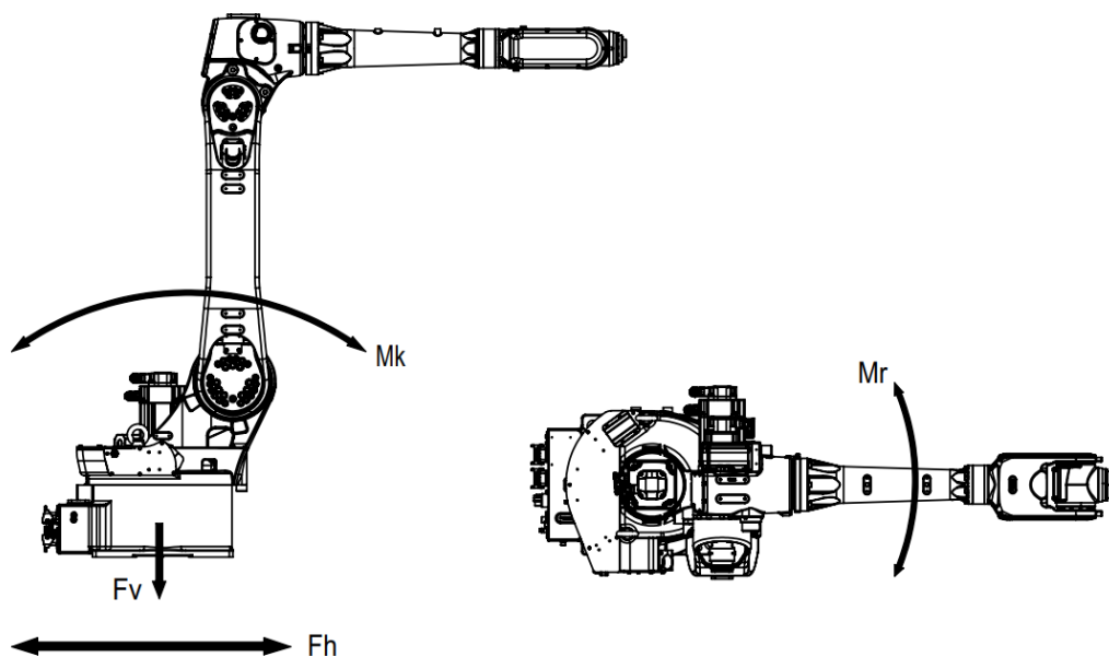
图 1-10 机器人底座受力数据 (ER8-1500-CW)
