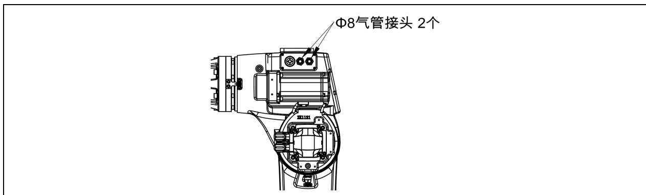
图 4-11 外部管线示意图 (ER8-2000-CW)
