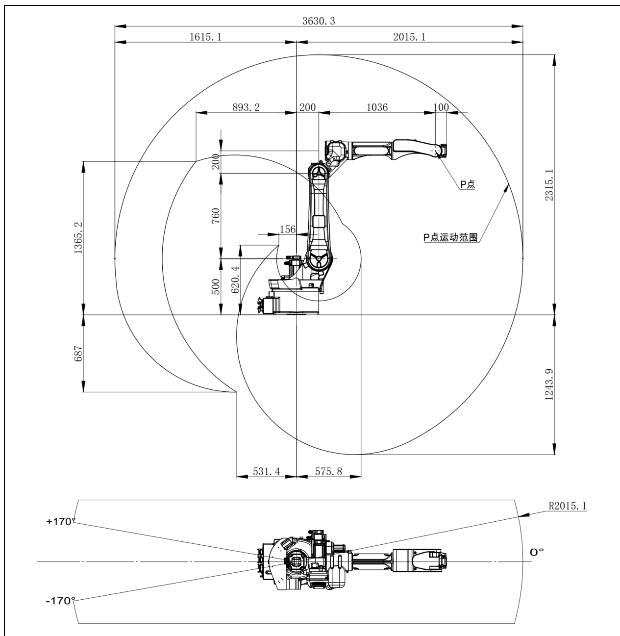
图 3-8 动作范围图 (ER8-2000-HW)
