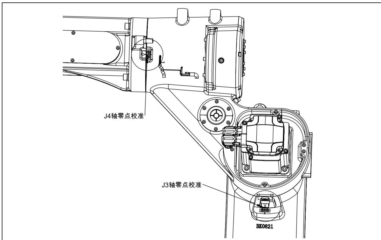
图 6-8 J3、J4 轴校准示意图 (ER8-2000-HW)
