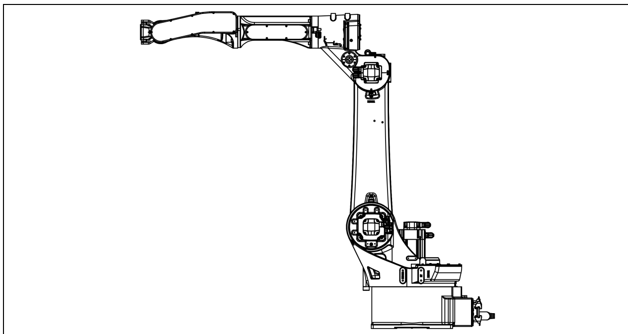
图 3-12 机器人的原点位置姿态 (ER8-2000-HW)
