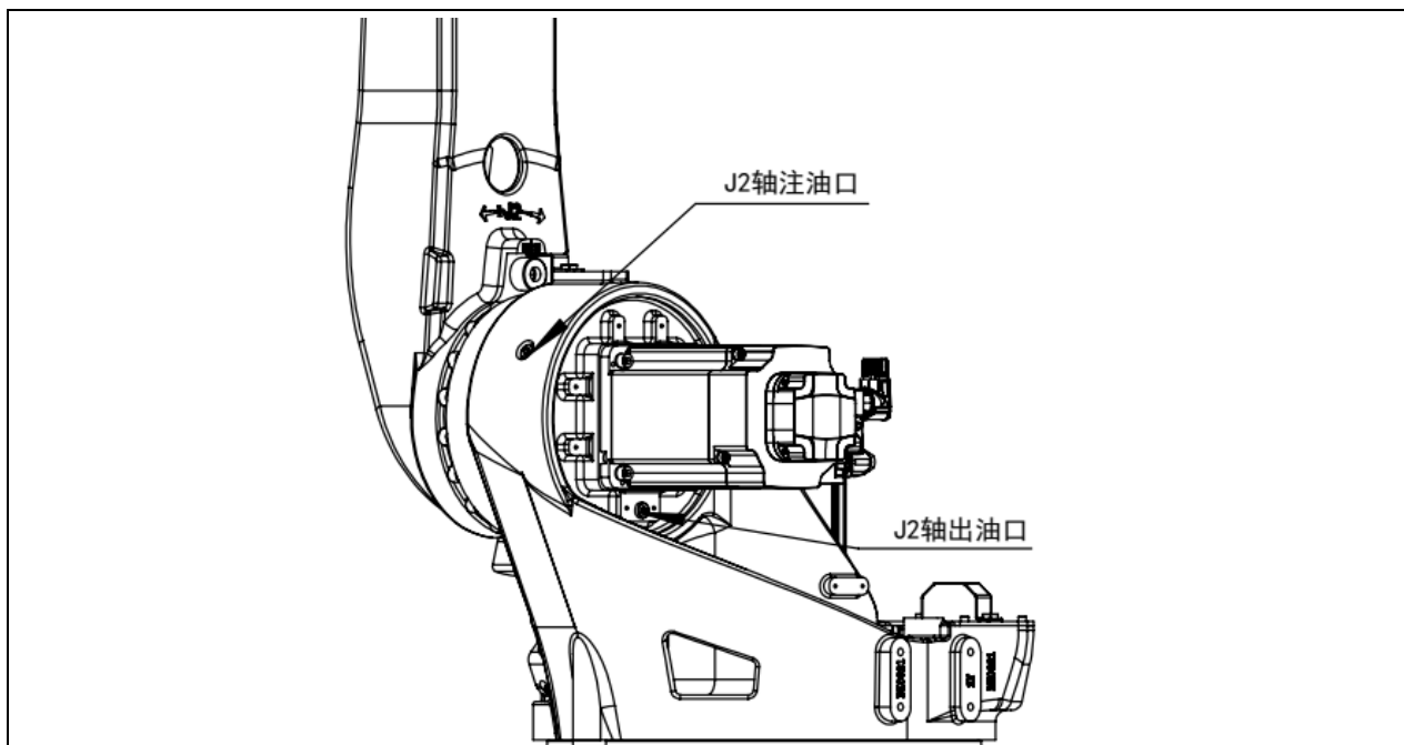
图 5-10J2 轴注油、出油口 (ER8-2000-CW)
