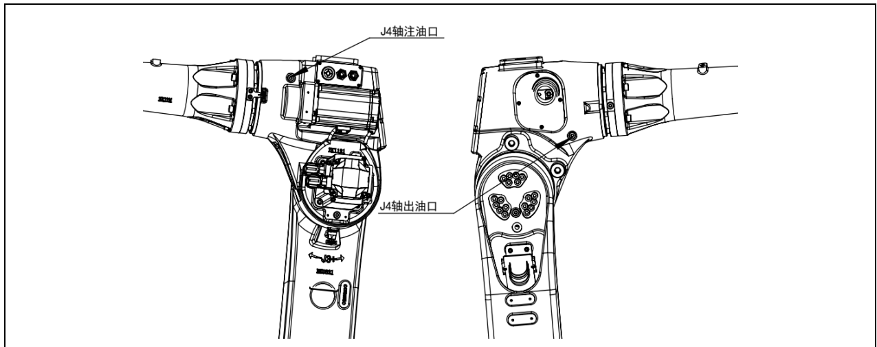
图 5-16J4 轴注油、出油口 (ER8-2000-CW)
