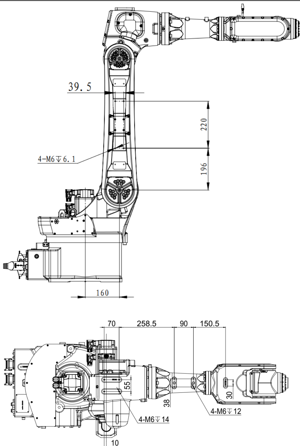
图 4-6 设备安装面尺寸 (ER8-1500-CW)
