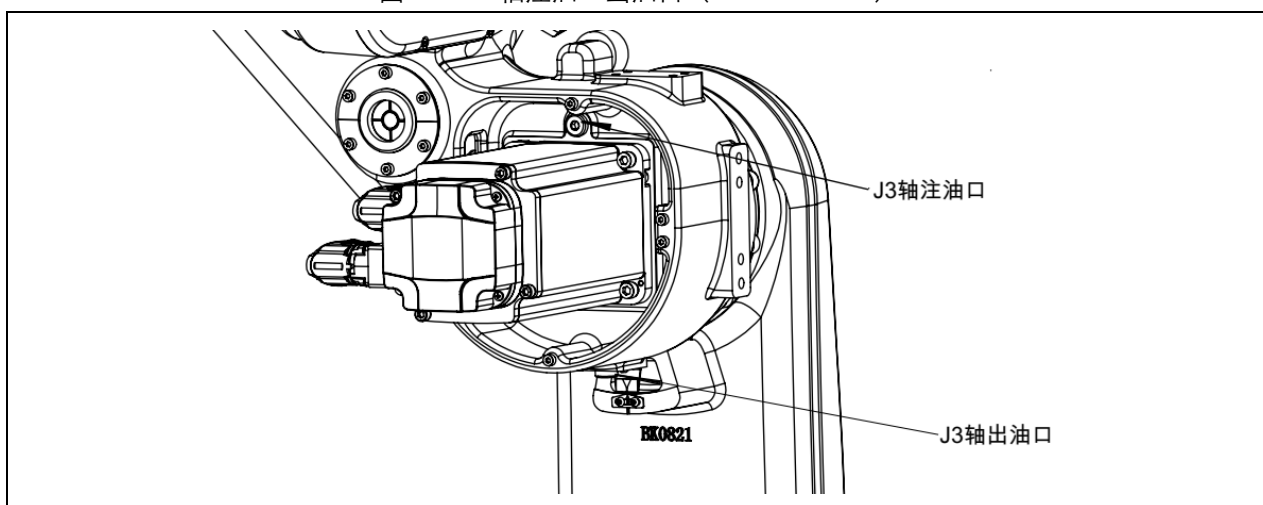
图 5-13J3 轴注油、出油口 (ER8-2000-HW)
