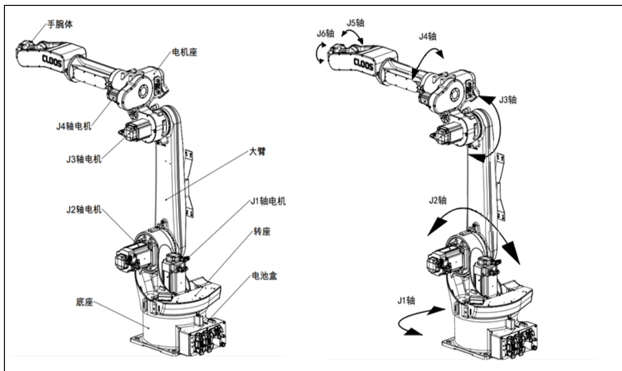
图 3-3 机器人的构成 (ER8-2000-HW)
