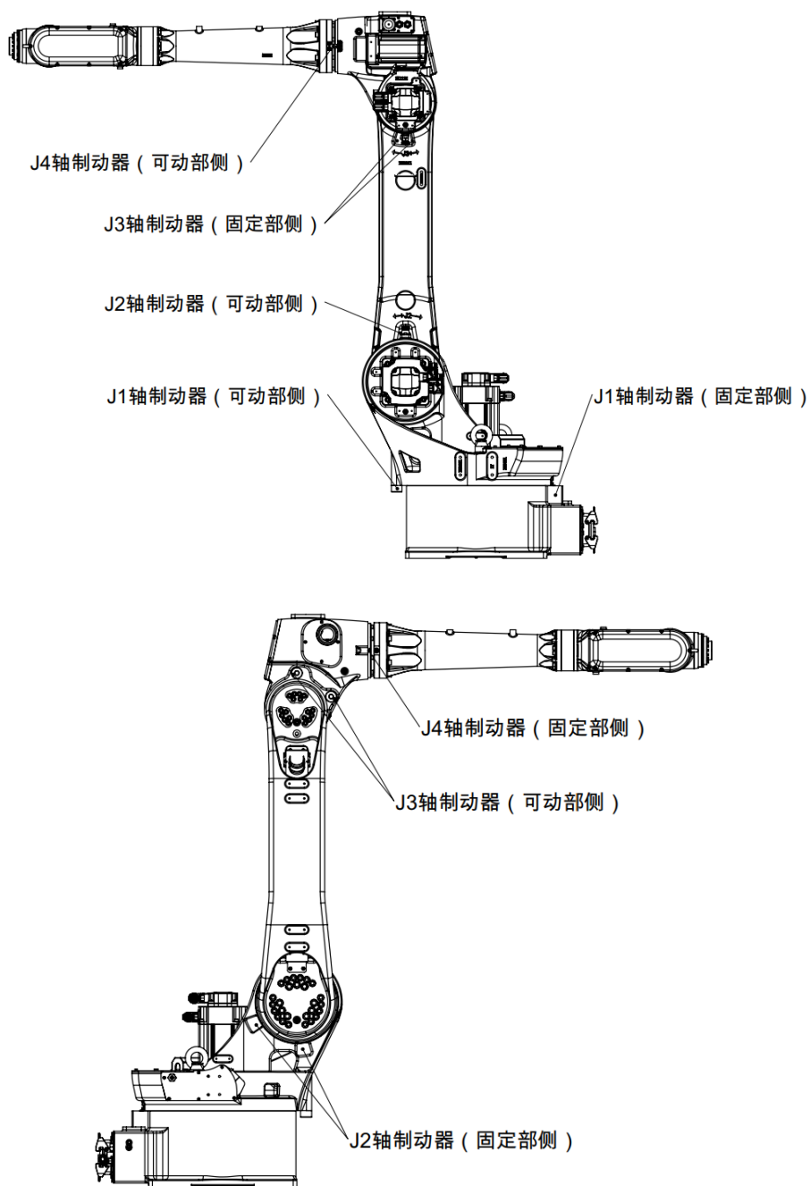
图 3-15 机械式制动器位置 (ER8-2000-CW)
