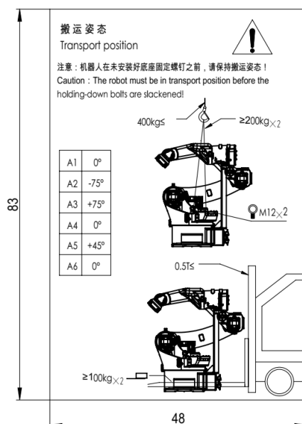
图 0-6 ER8-1450-HW 搬运标识
