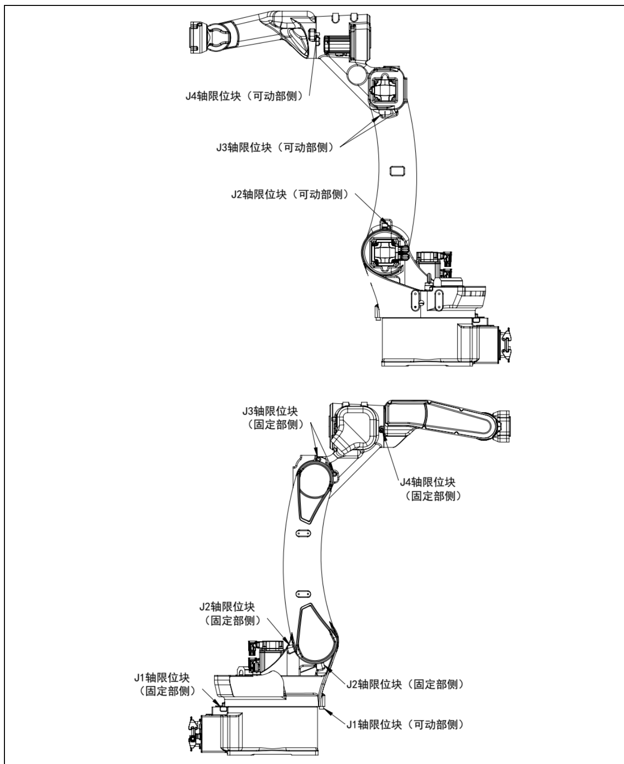
图 3-13 机械式制动器位置（ER8-1450-HW）
