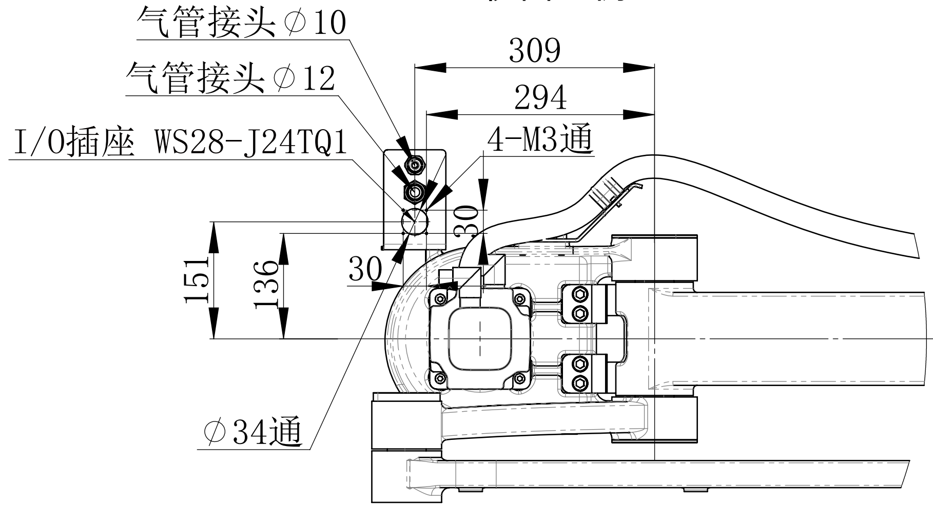
视图比例1:5
