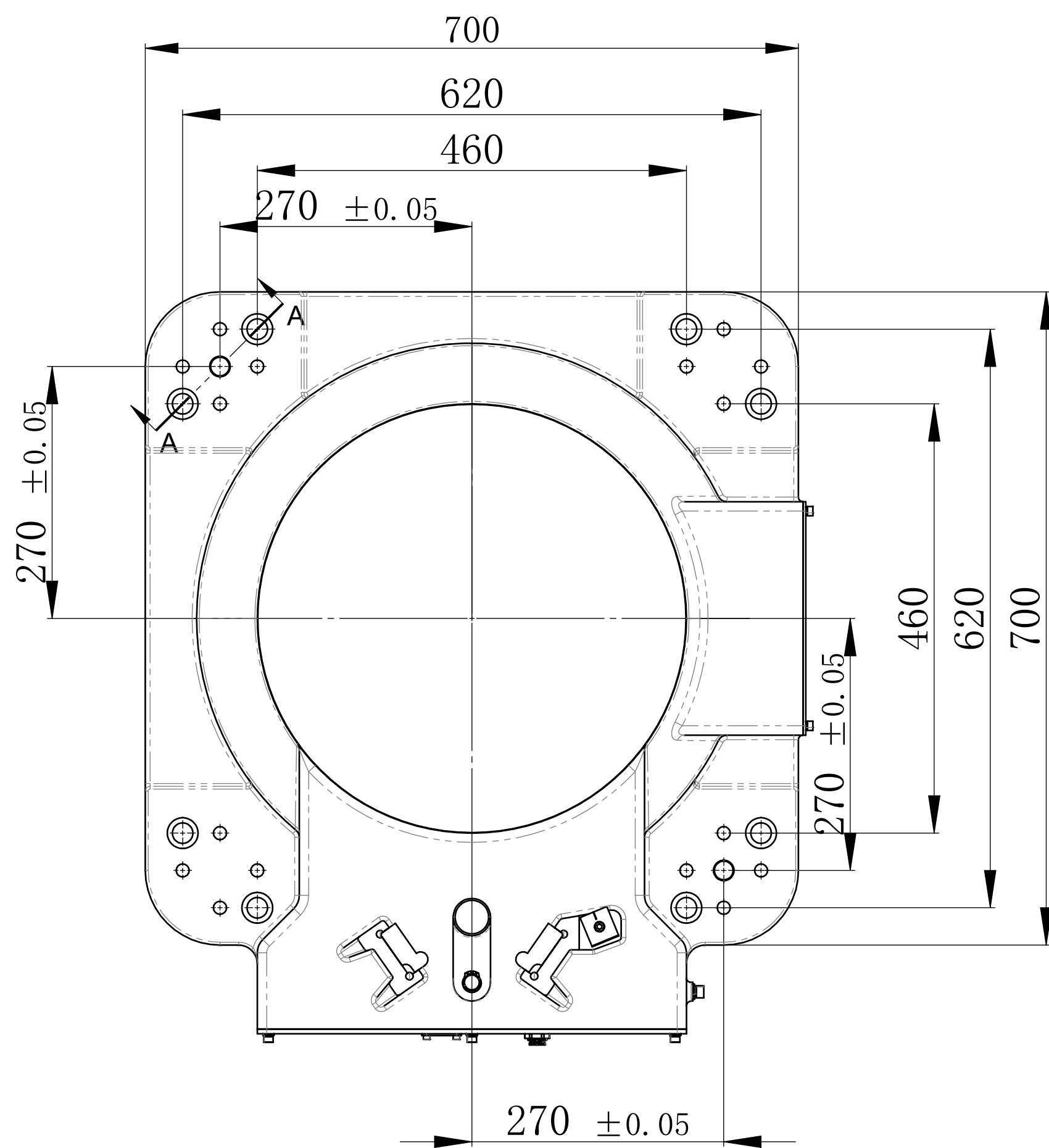
底座安装接口 视图比例1:5
