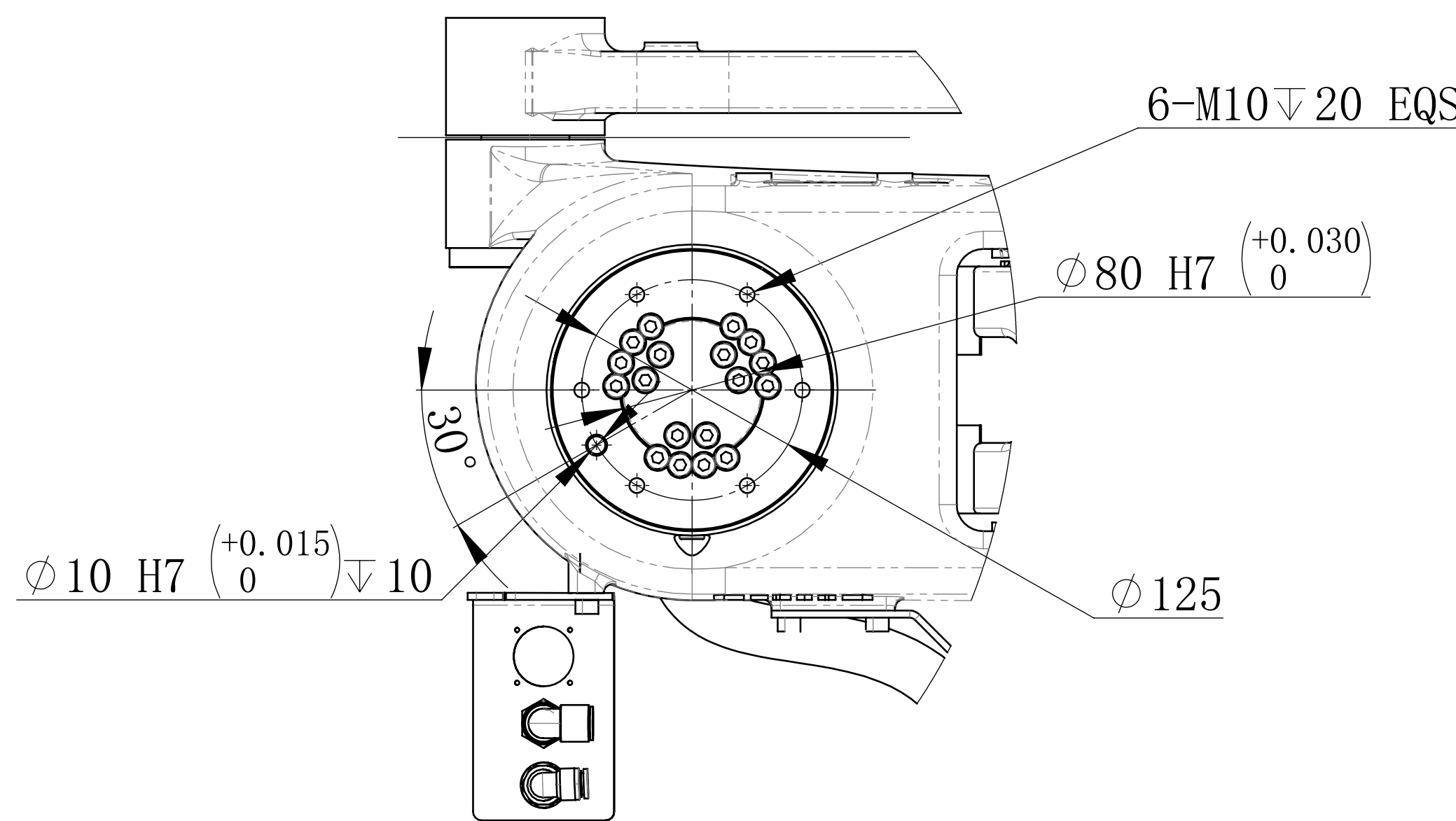
末端法兰安装接口 视图比例1:3
