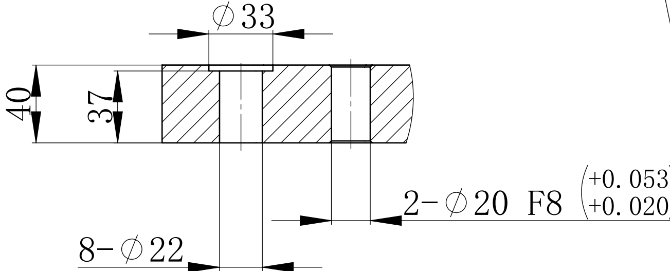
A-A 1 : 2
