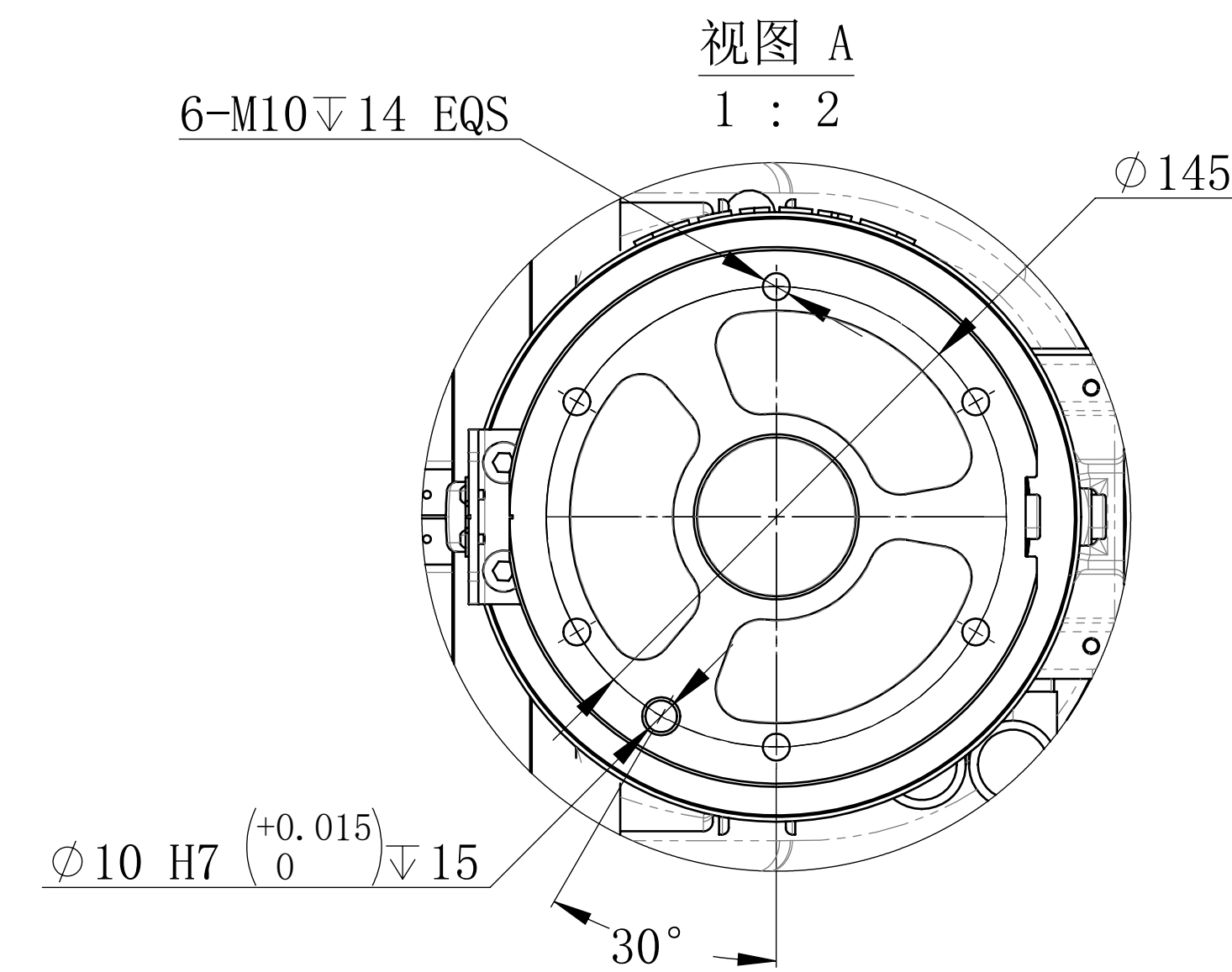
末端法兰安装接口 视图比例1:2
