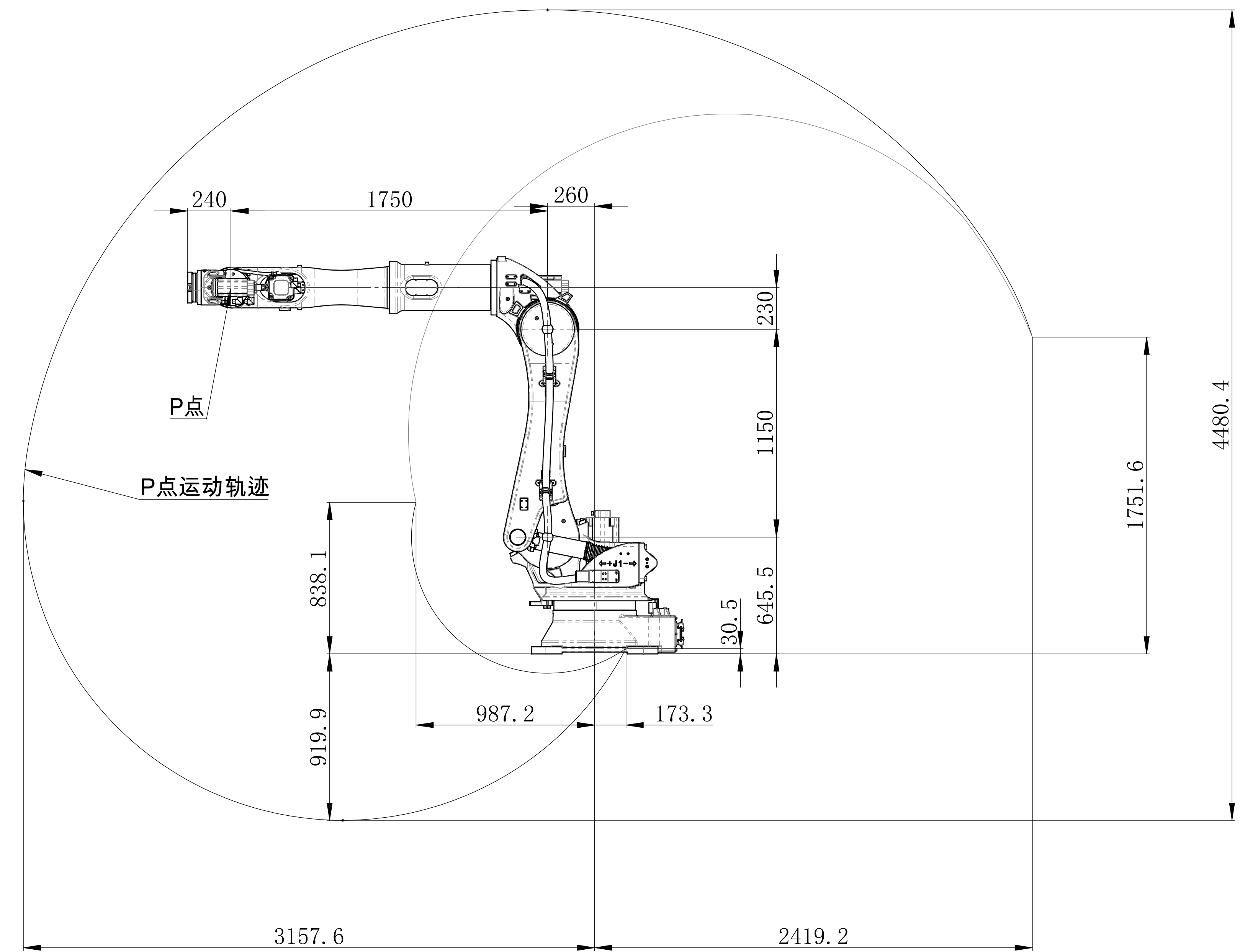
动作范围图 视图比例1:16
