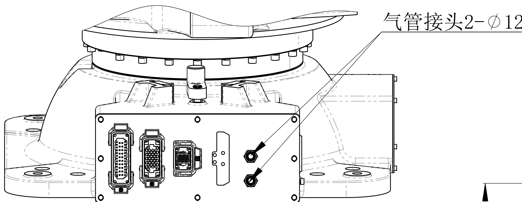
视图C
