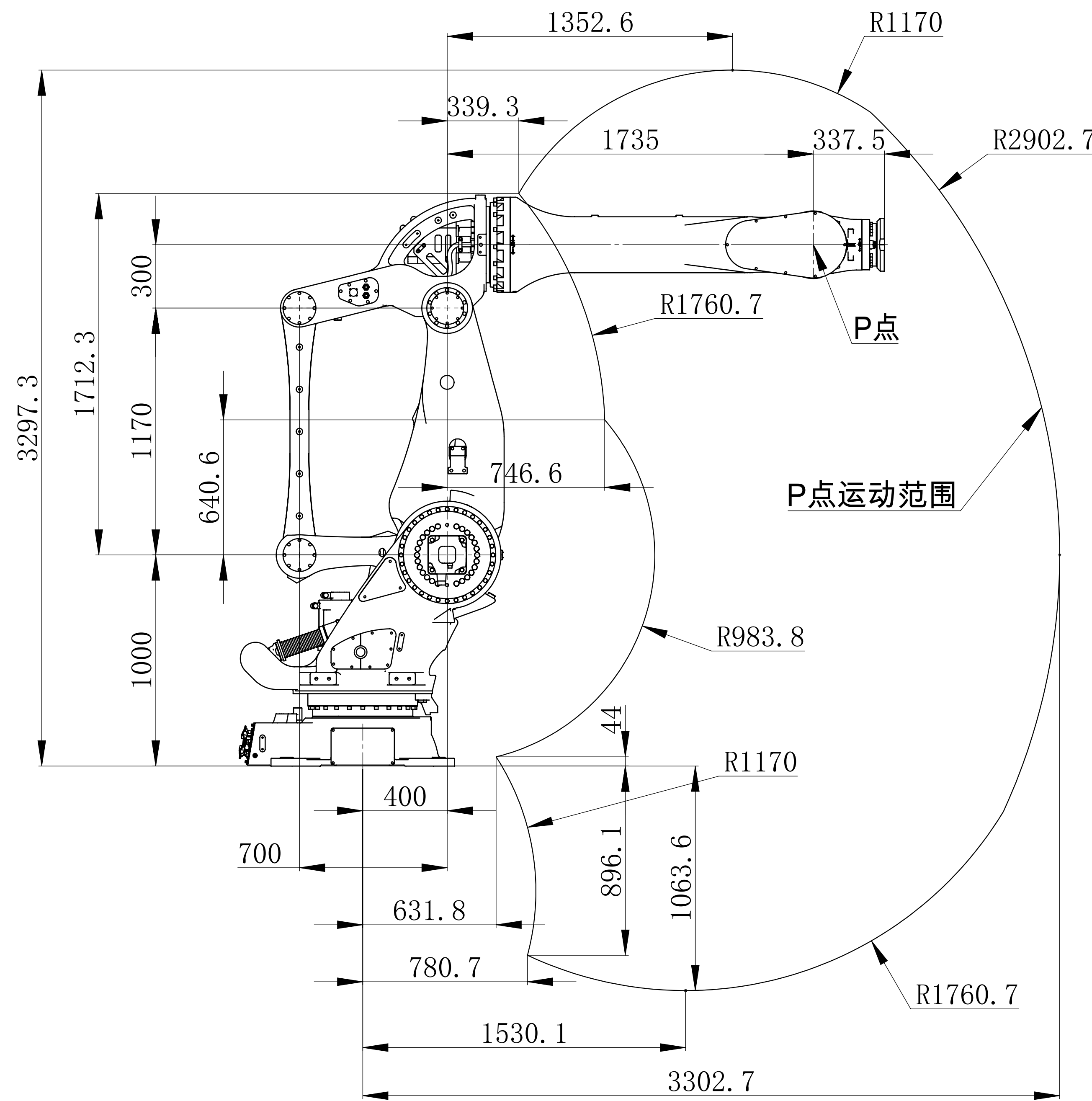
动作范围图
