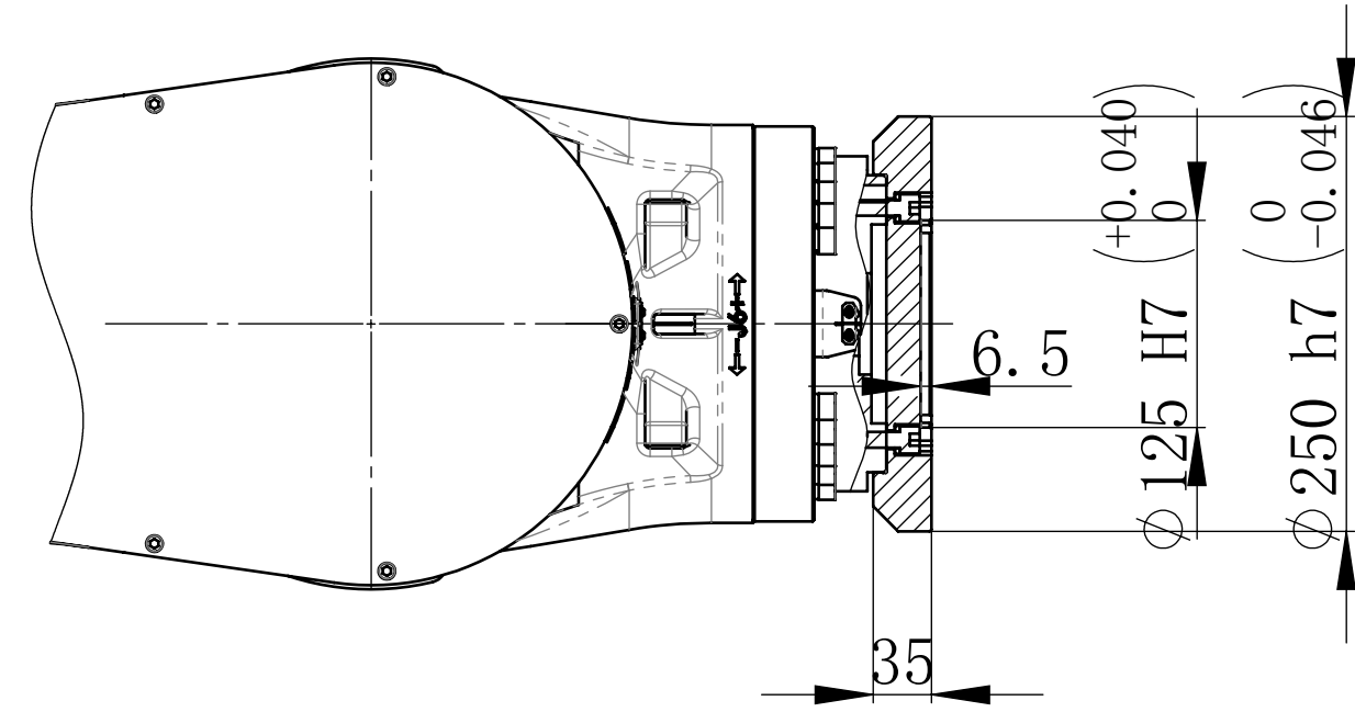
末端法兰安装接口
