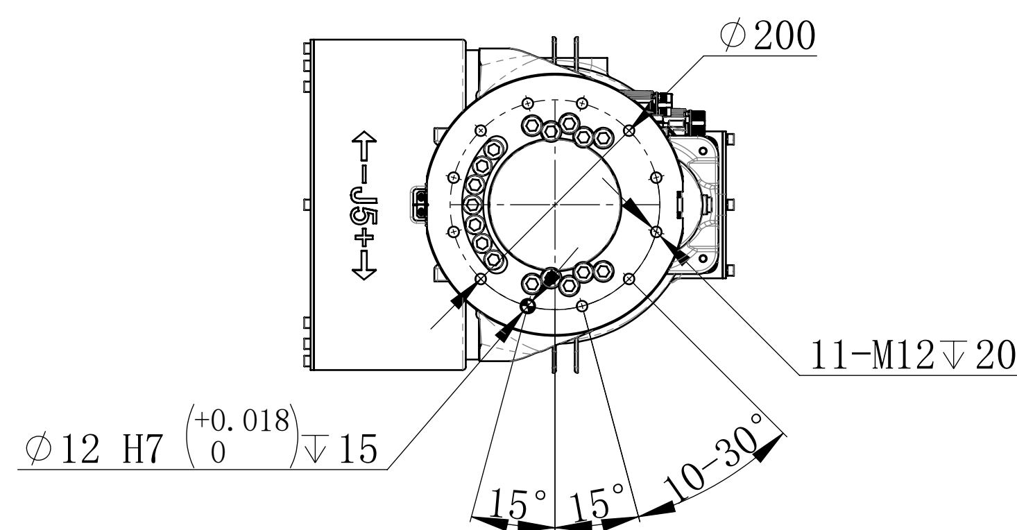
末端法兰安装接口
