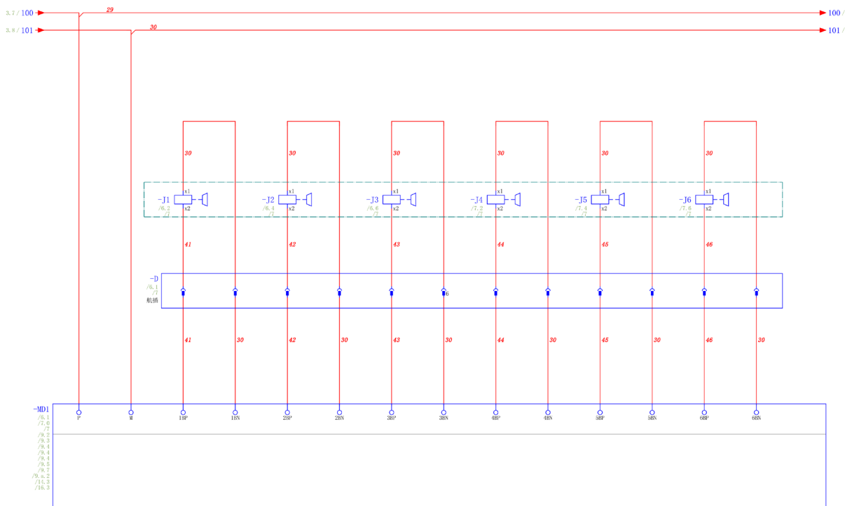
图 3.10 电机抱闸
