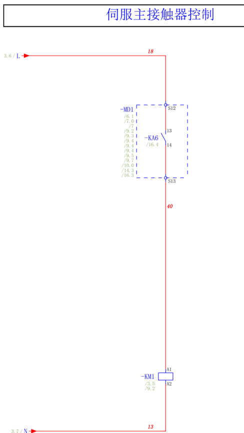
图 3.9 AC 220V 控制回路
