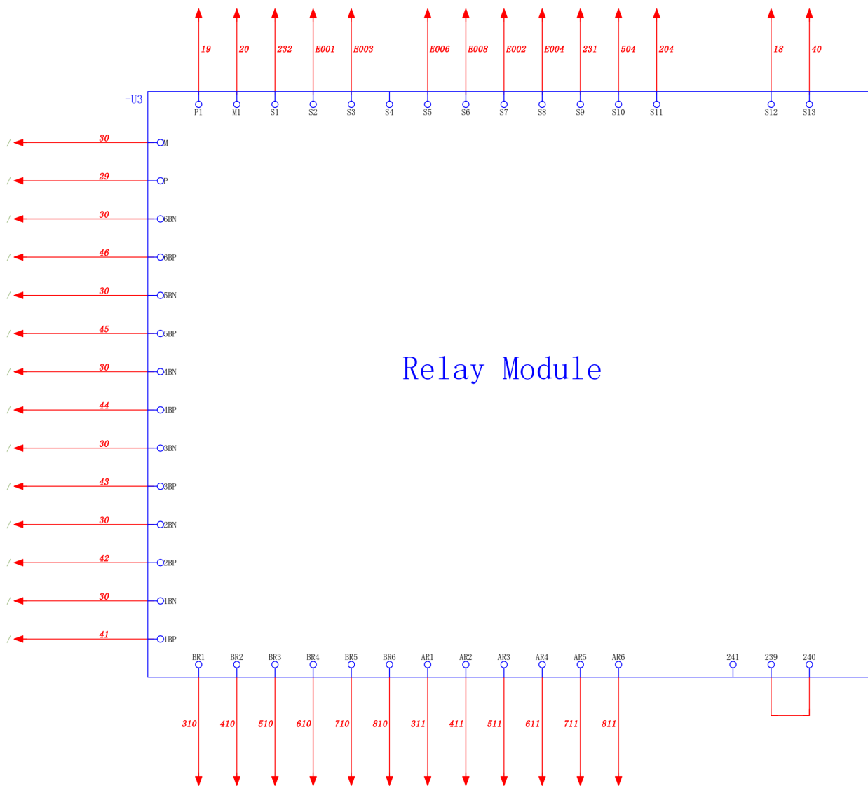
图 3.23 继电器模组
