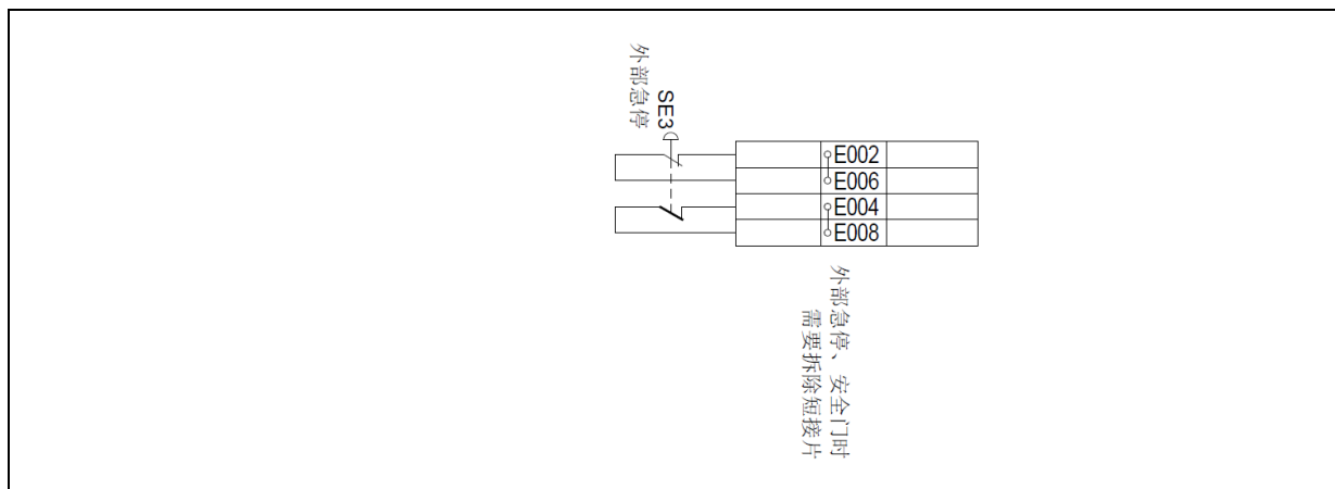
图 3.18 急停接线图
