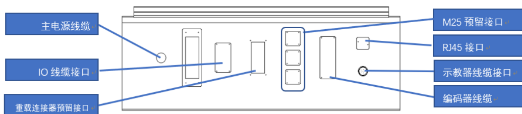
图 3.1 对外接口
