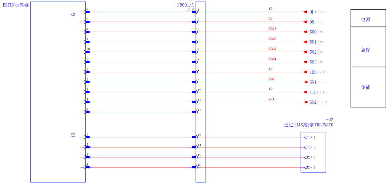
图 3.11 示教器接线
