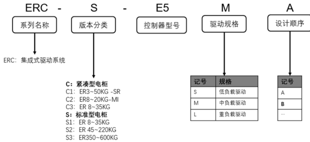
图 1.3 型号说明
