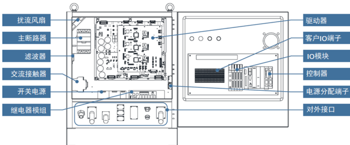
图 1.5 内部结构
