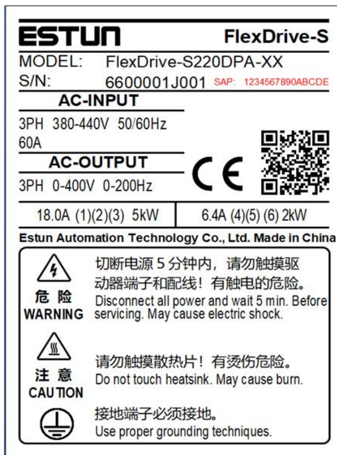
图 1.2 驱动铭牌示意图
