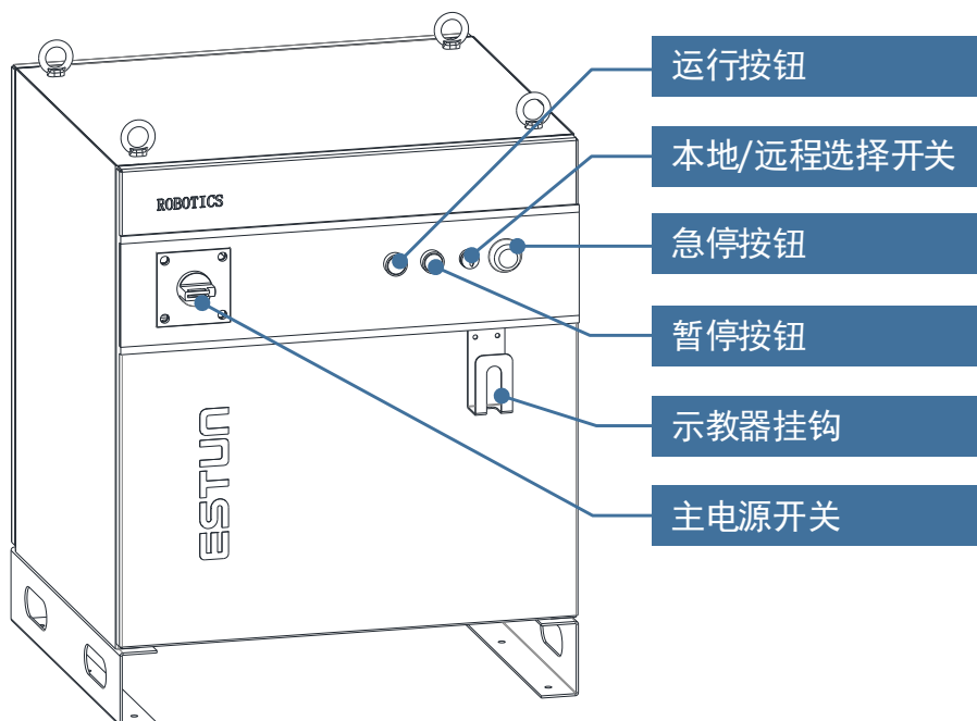
图 1.4 外观说明
