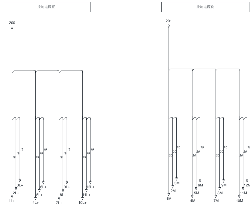
图 3.5 控制电源 24V
