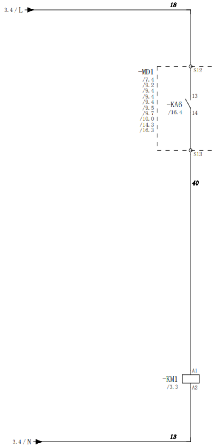
图 3.8 AC 220V 控制回路
