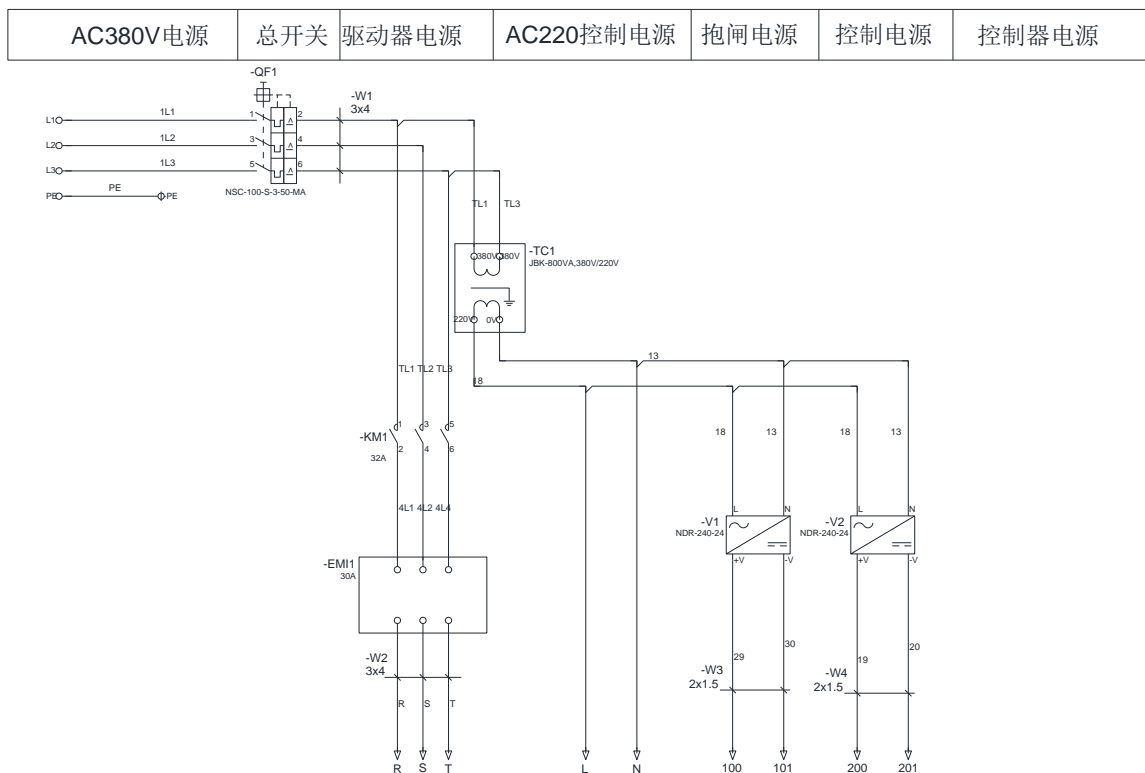
图 3.4 电源分配
