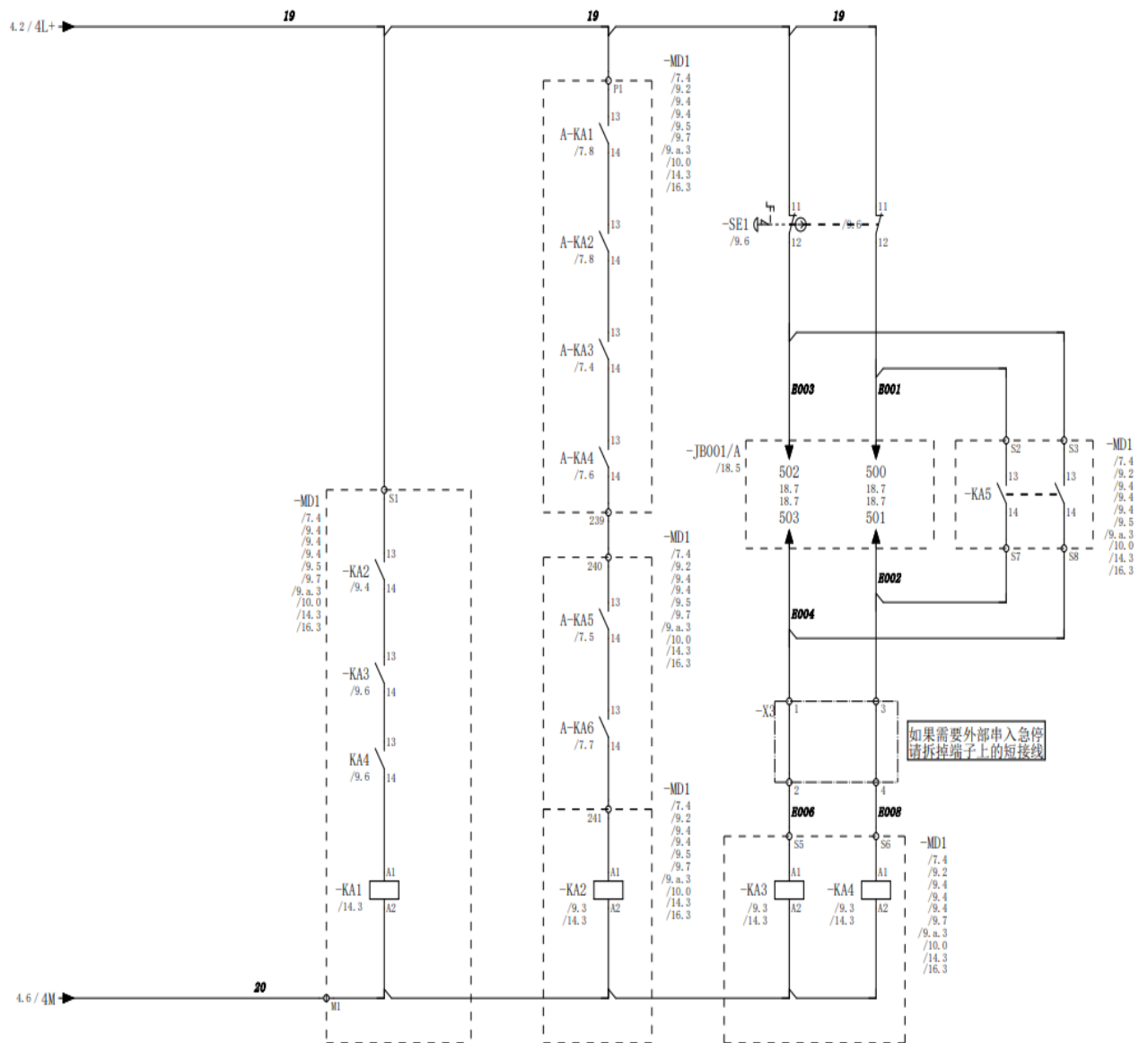
图 3.7 DC 24V 控制回路
