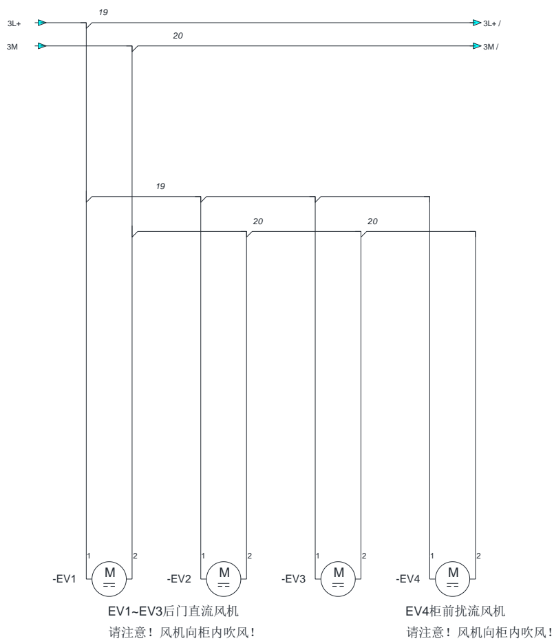
图 3.6 散热风机
