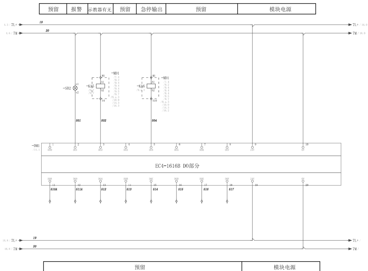
图 3.17 输出模块
