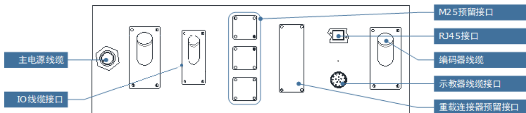
图 3.1 对外接口说明
