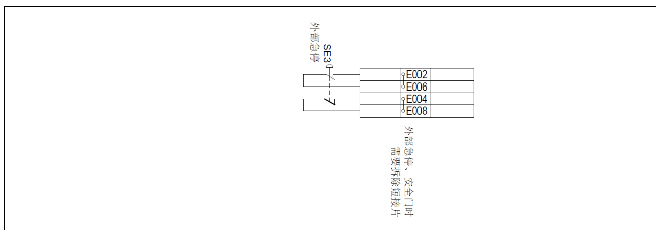
图 3.13 急停接线图
