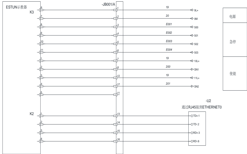
图 3.11 示教器接线
