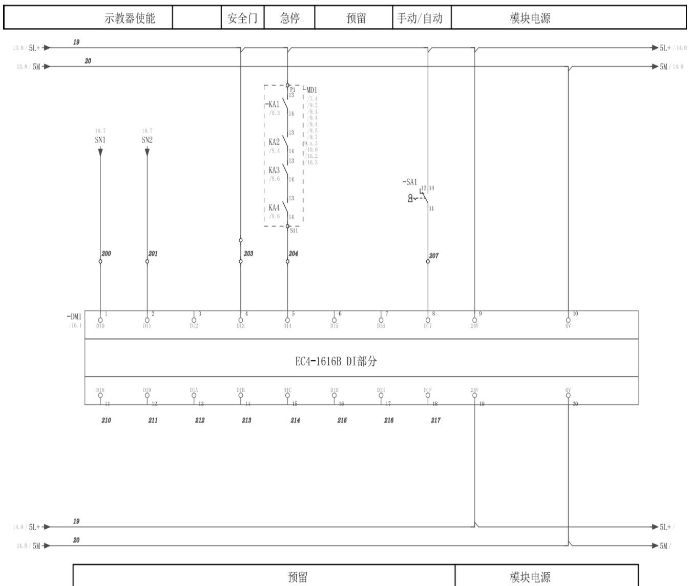
图 3.16 输入模块
