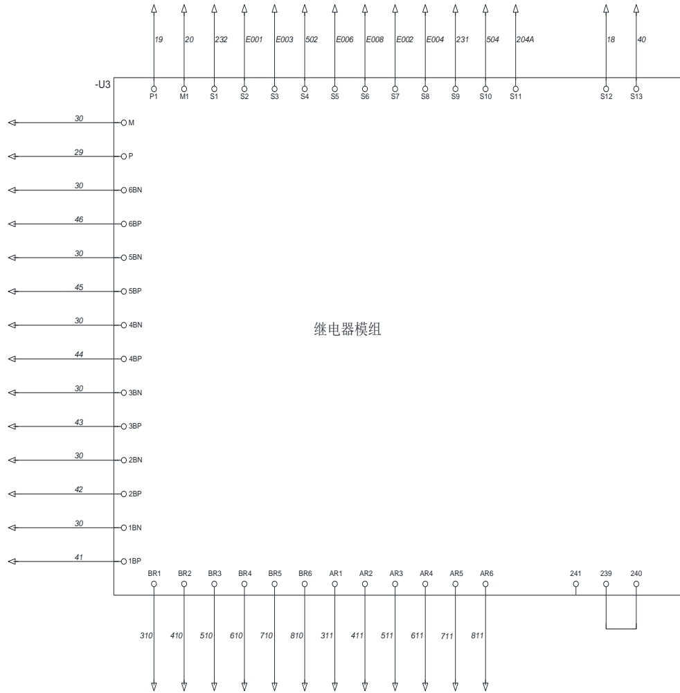
图 3.19 继电器模组
