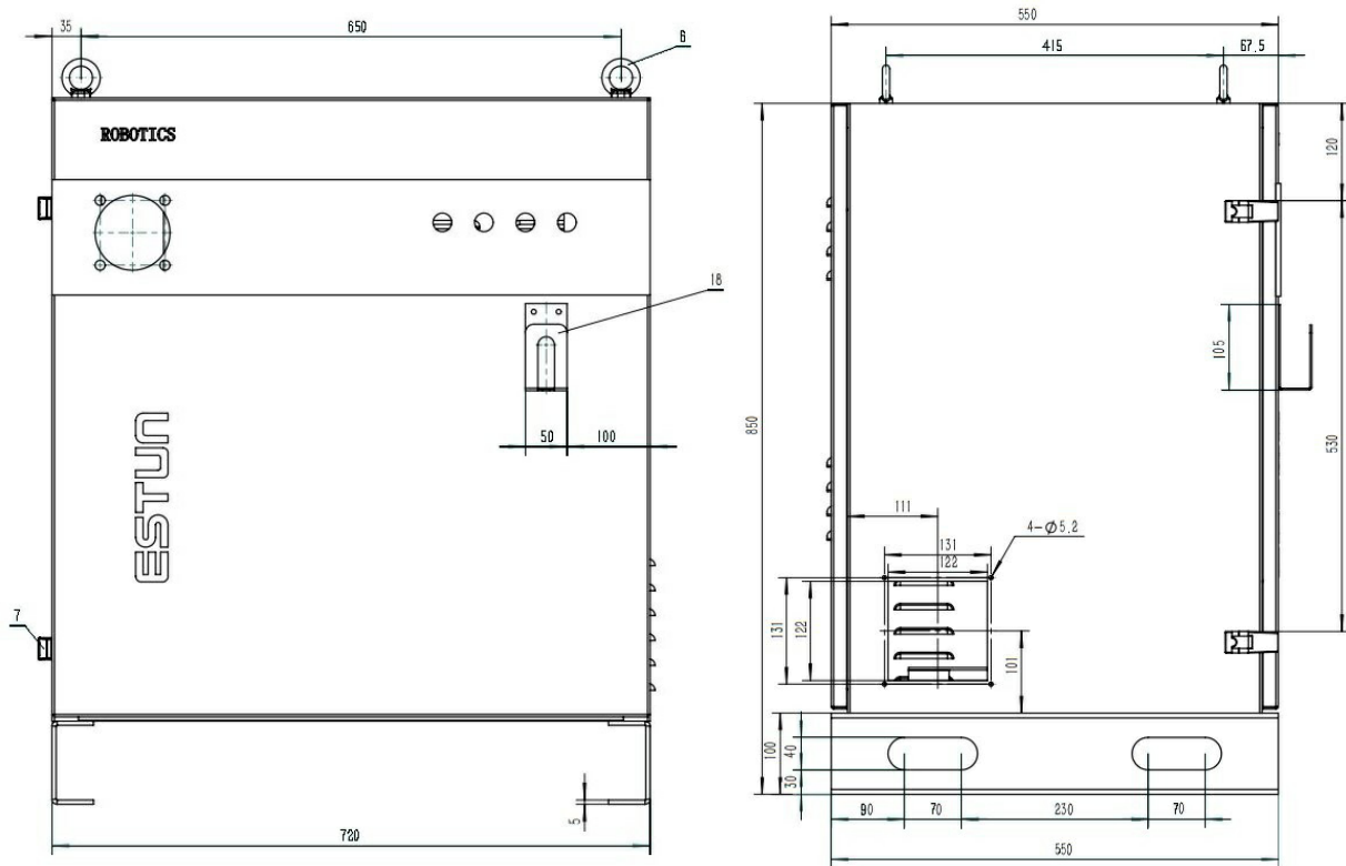
图 1.7 产品尺寸
