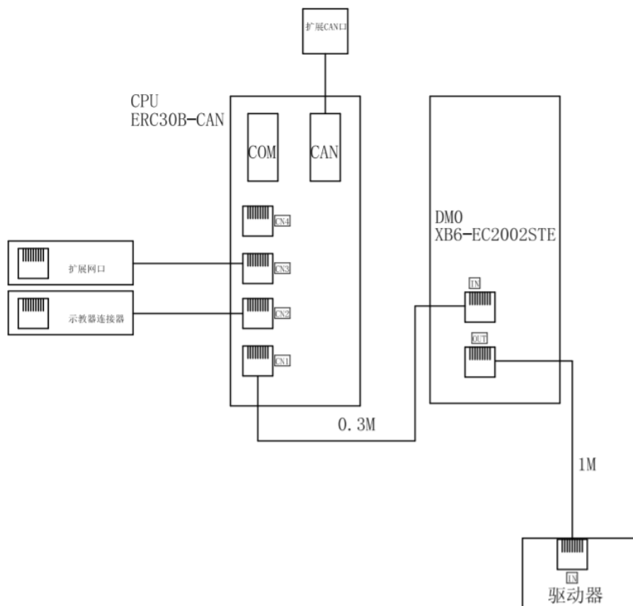
图 3.12 通讯连接图
