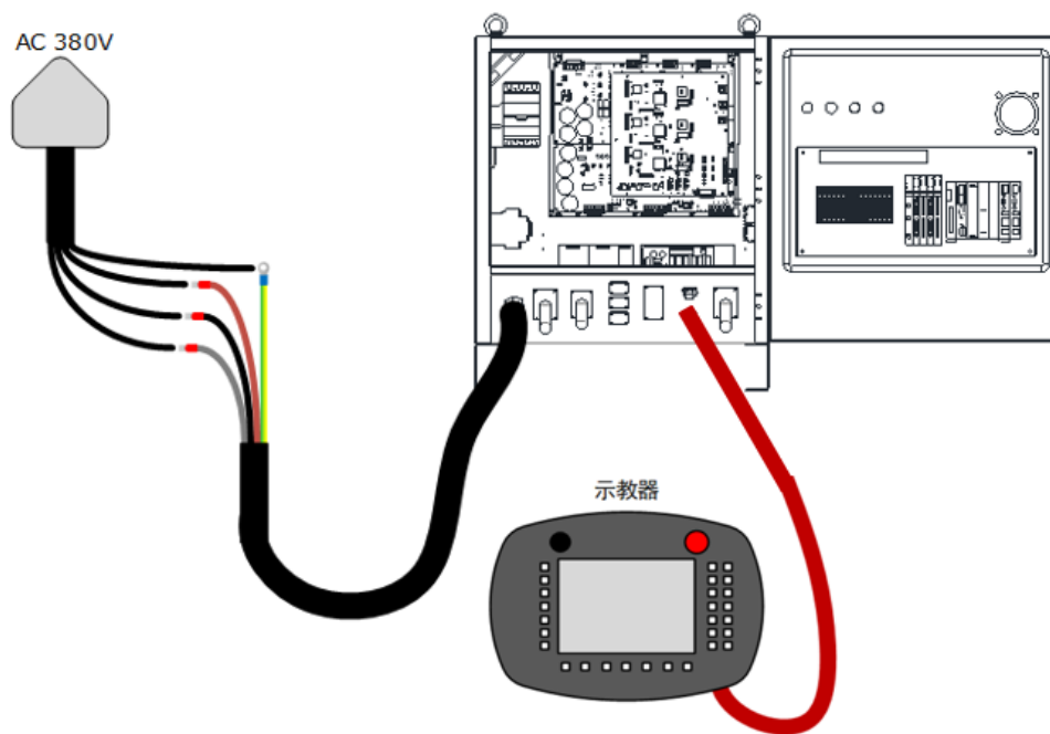
图 3.1 基本示意图
