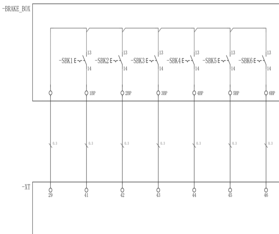
图 3.10 抱闸释放
