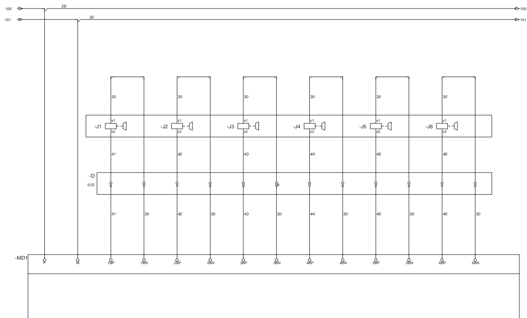
图 3.9 电机抱闸
