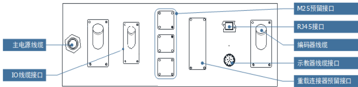
图 1.6 对外接口
