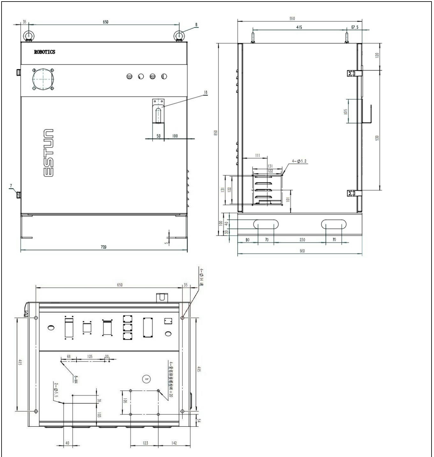
图 2.1 装配尺寸图
