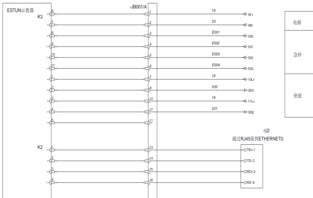
图 3.13 示教器接线
