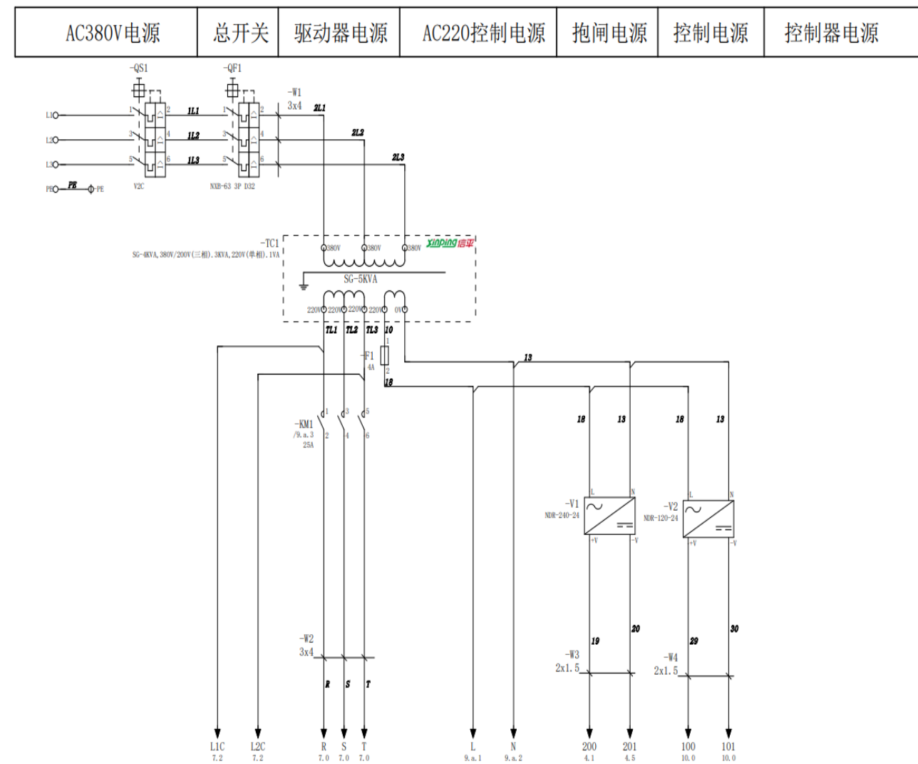
图 3.5 电源分配
