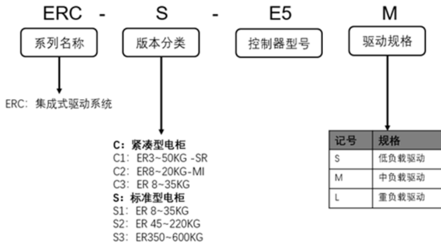
图 1.3 型号说明
