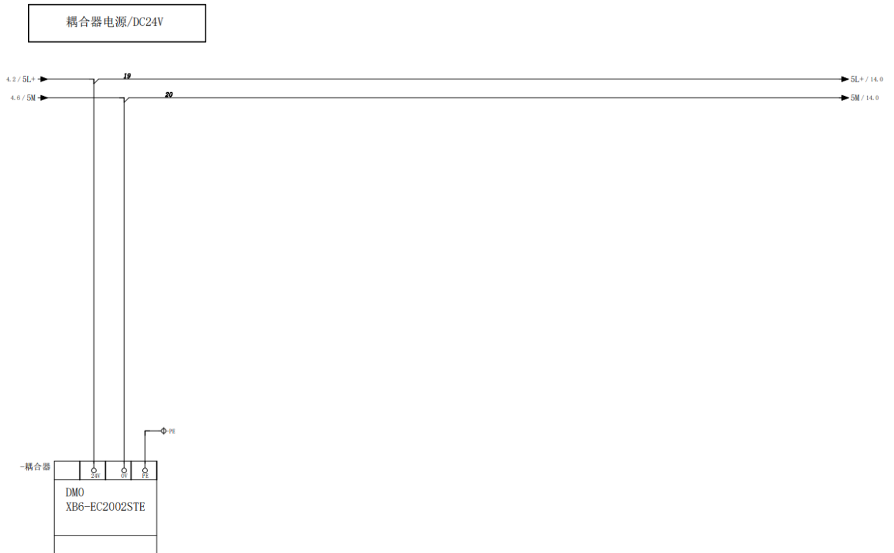
图 3.17 耦合器电源
