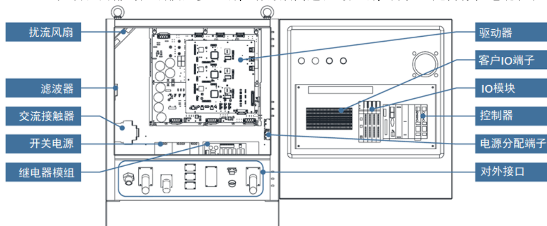
图 1.5 内部结构
