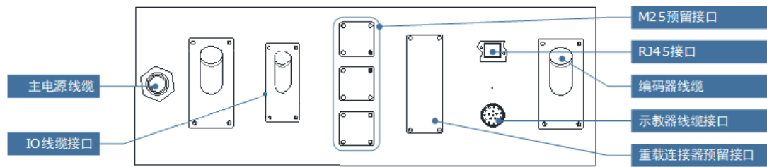
图 3.2 对外接口
