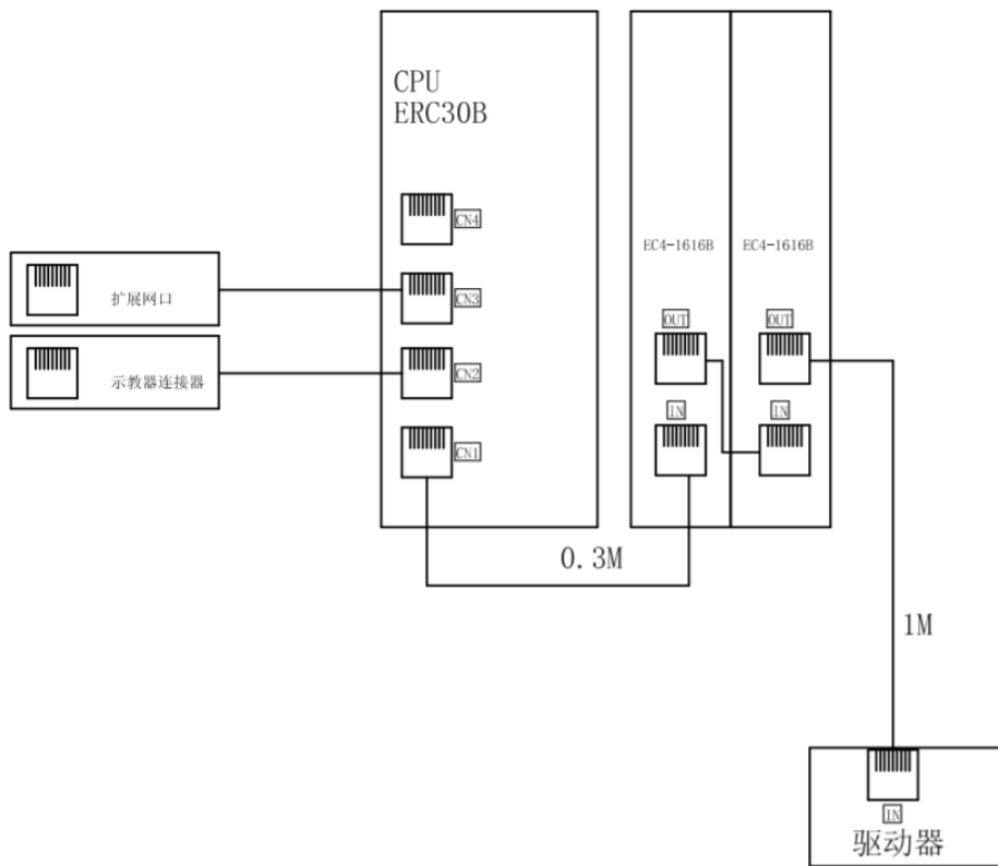
图 3.15 通讯连接图 (ERC-S1-E4SB)
