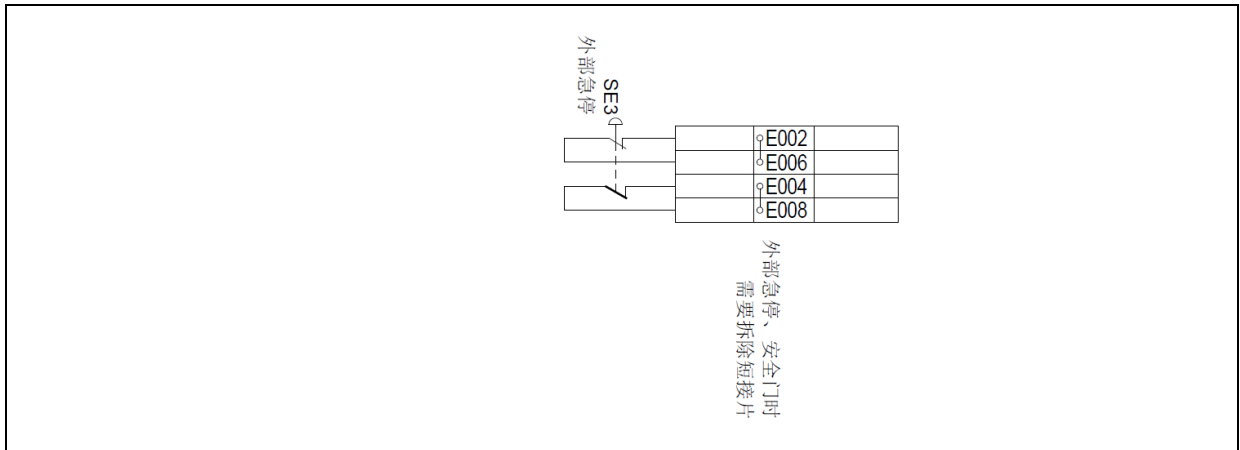
图 3.18 急停接线图
