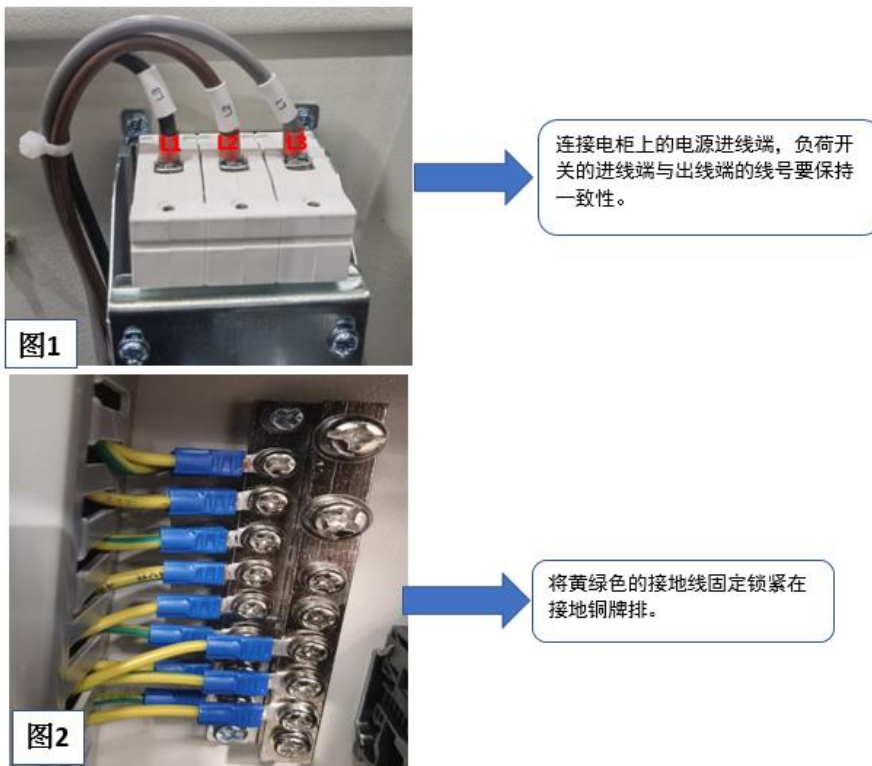
图 3.4 电源线束装配示意图（三相 2）
