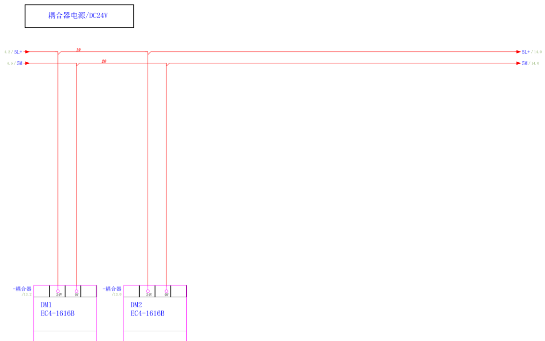
图 3.19 耦合器电源
