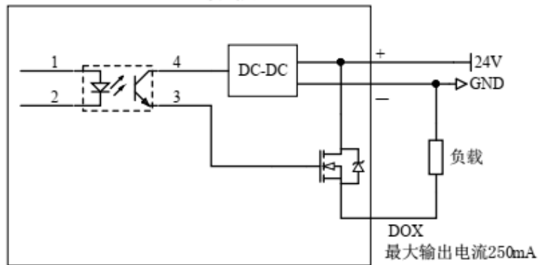
图 3.14 DO PNP 型接线图
