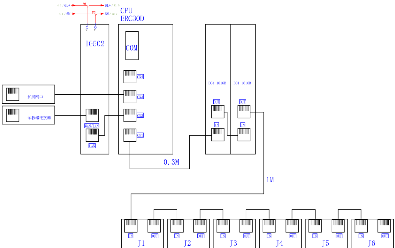
图 3.17 通讯连接图（选配运维精灵）
