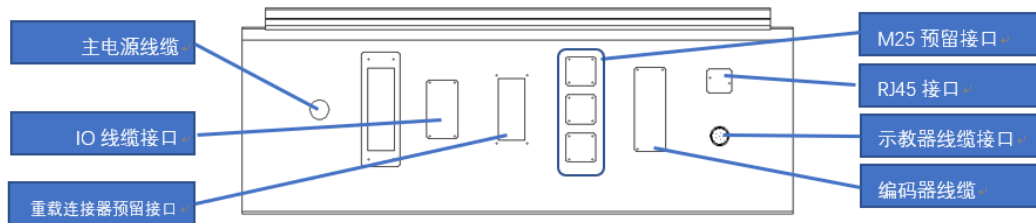
图 3.1 对外接口
