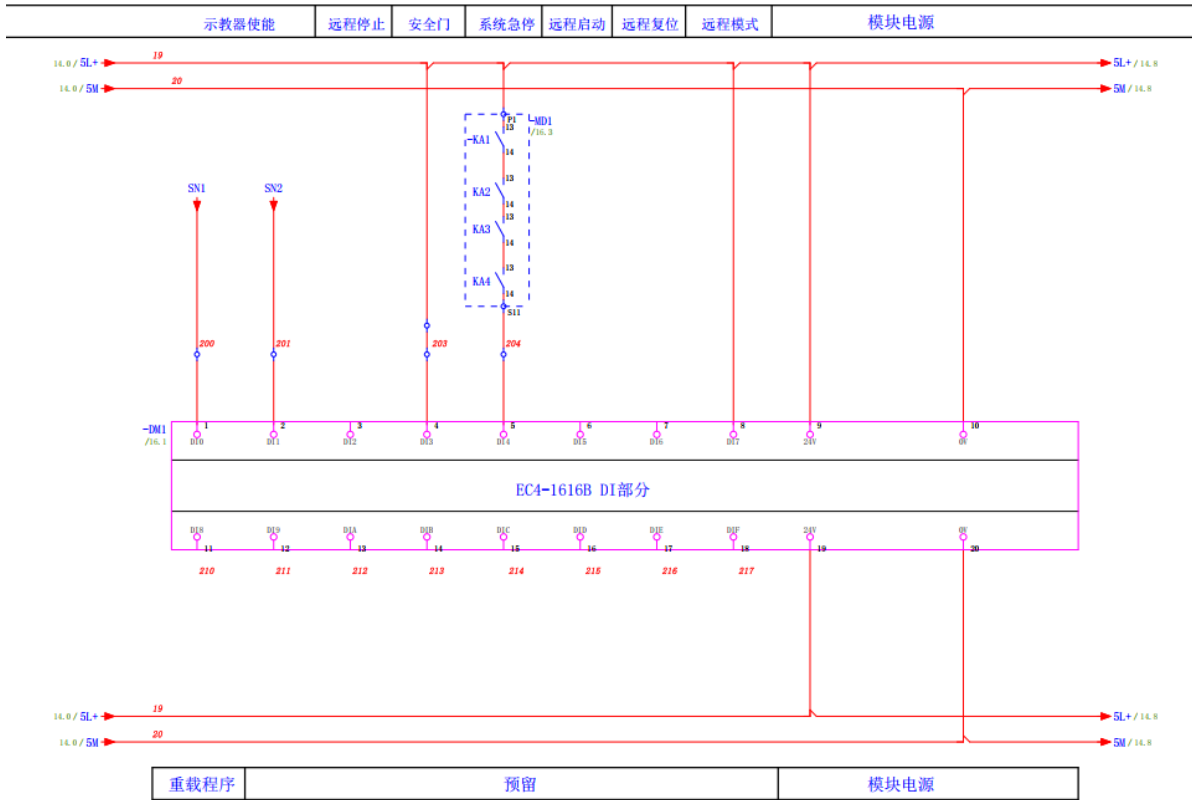
图 3.20 输入模块
