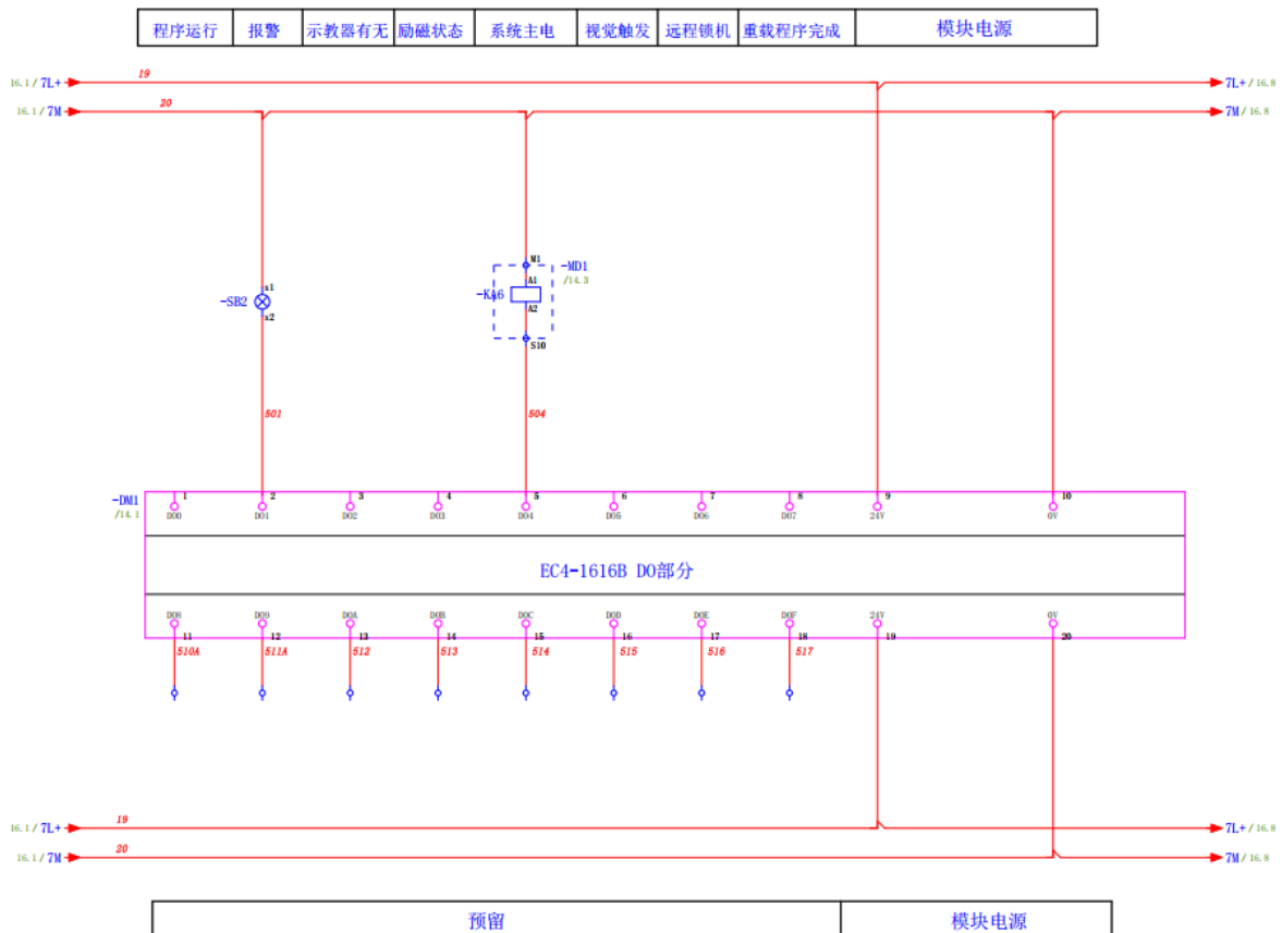
图 3.21 输出模块
