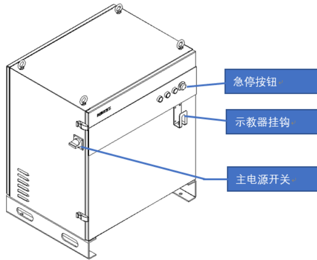
图 1.3 外观说明
