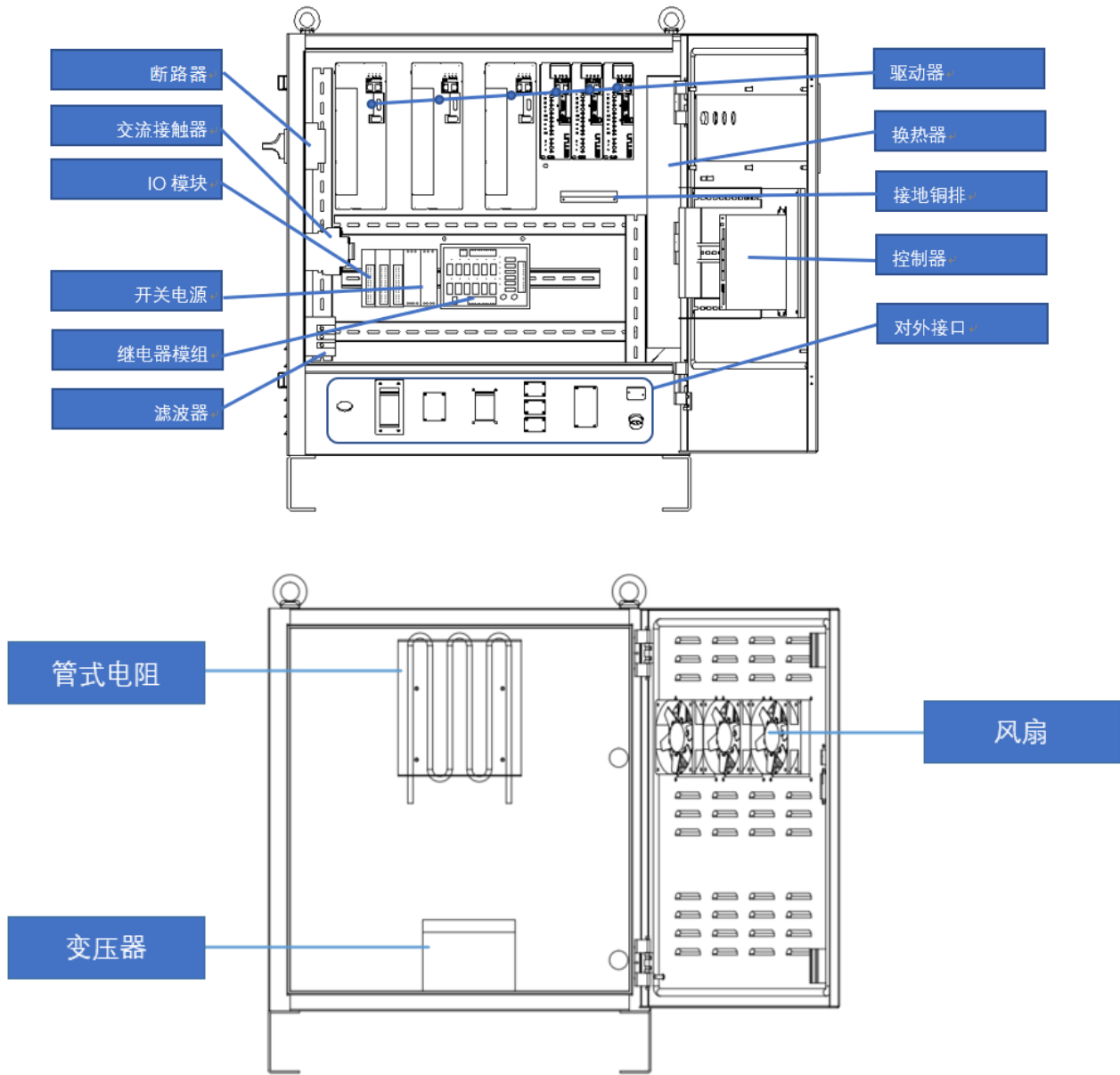
图 1.4 内部结构
