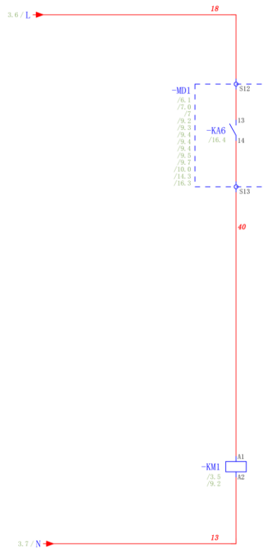
图 3.9 AC 220V 控制回路
