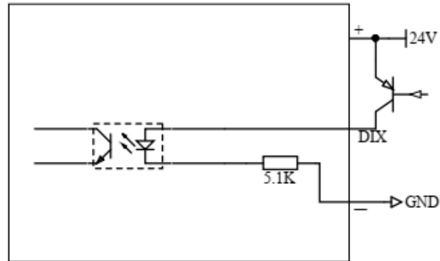
图 3.13 DI PNP 型接线图
