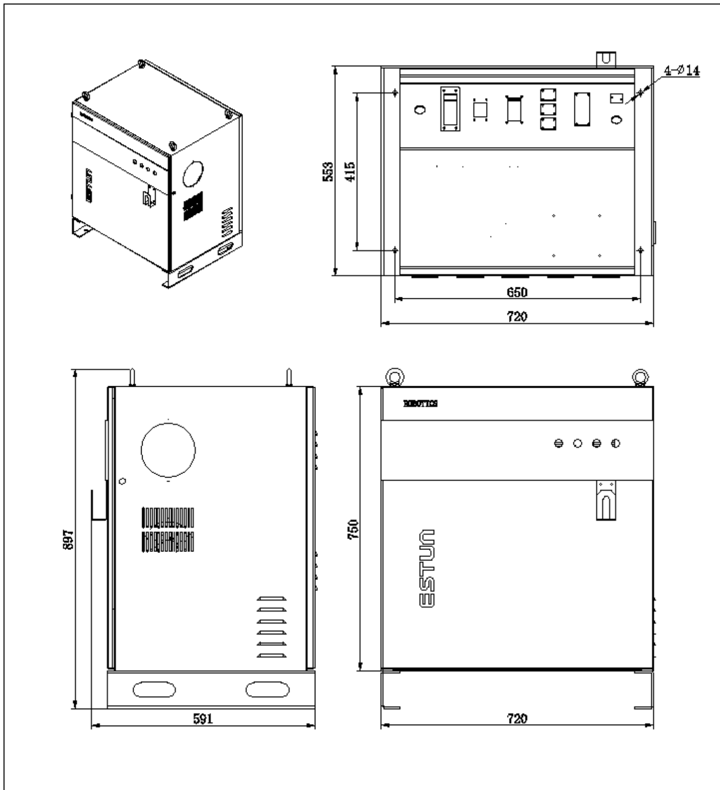
图 1.6 产品尺寸图
