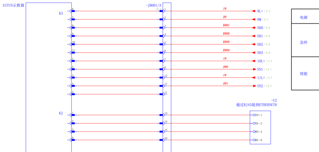
图 3.11 示教器接线
