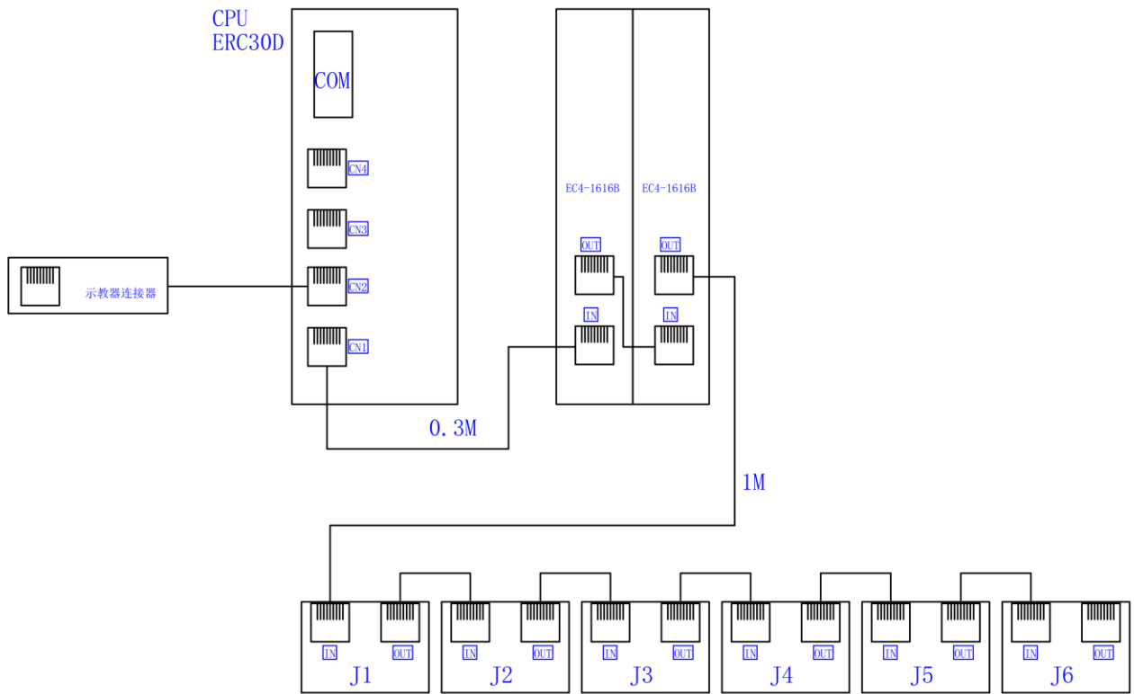
图 3.16 通讯连接图
