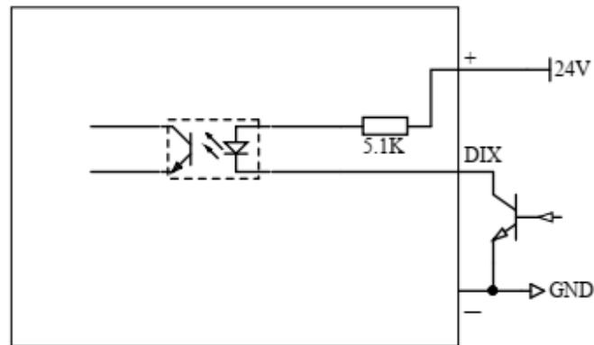
图 3.15 DI NPN 型接线图
