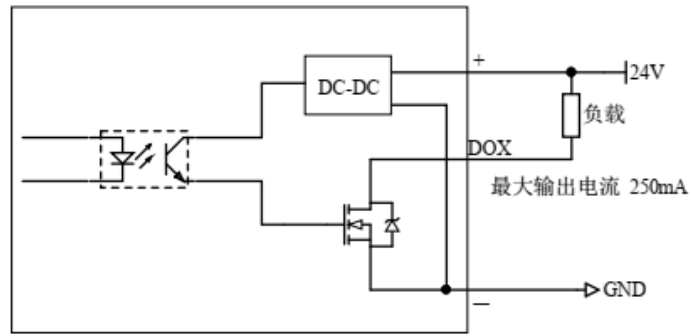
图 3.12 DO NPN 型接线图
