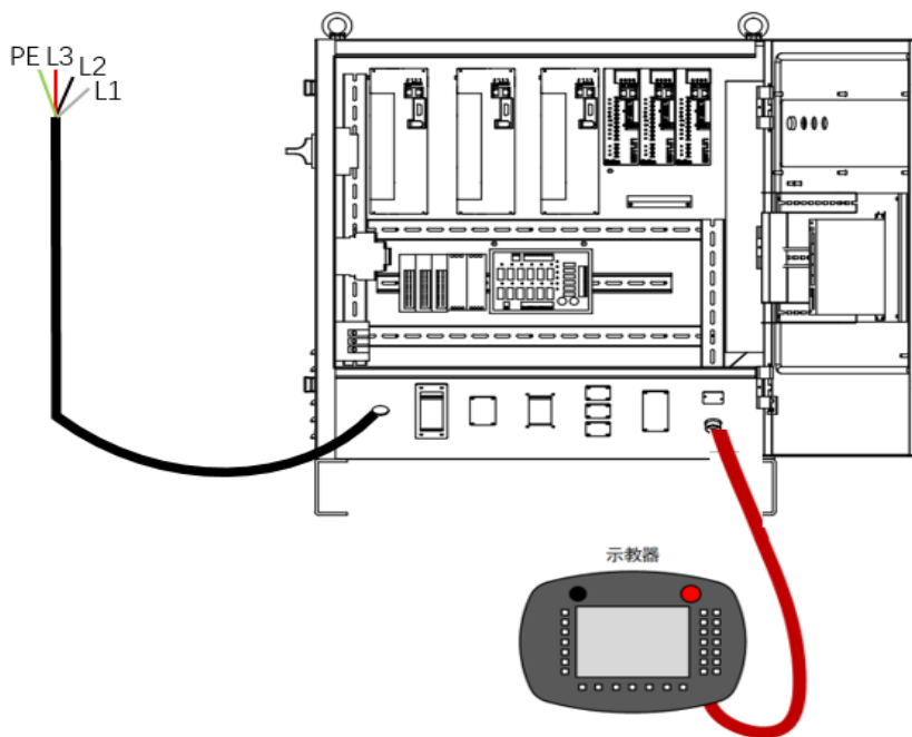
图 3.2 基本示意图
