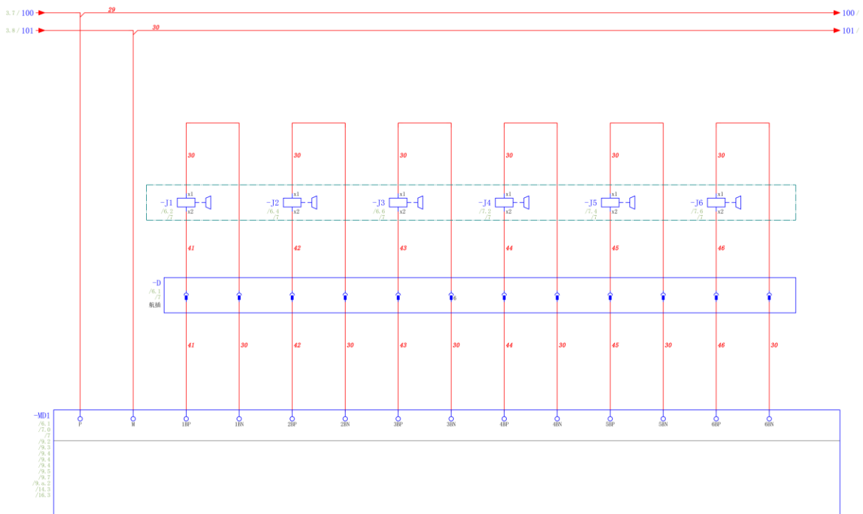
图 3.10 电机抱闸
