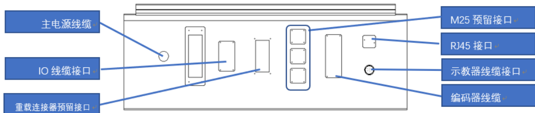
图 1.5 对外接口
