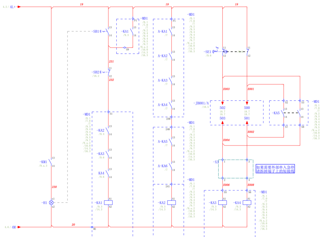
图 3.8 DC 24V 控制回路
