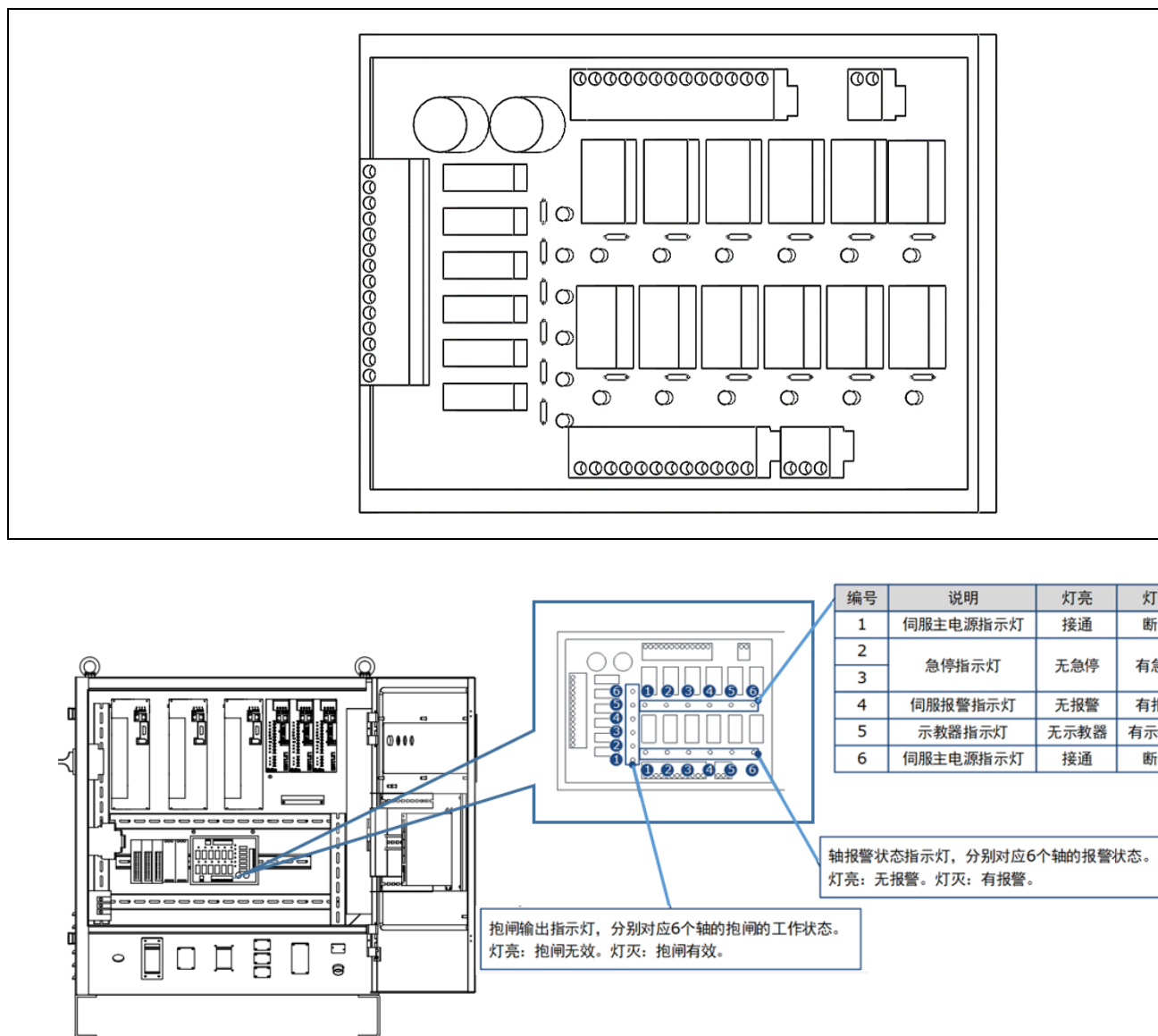
图 3.22 继电器模组指示灯
