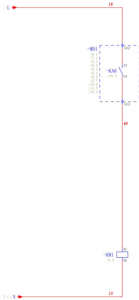
图 3.9 AC 220V 控制回路
