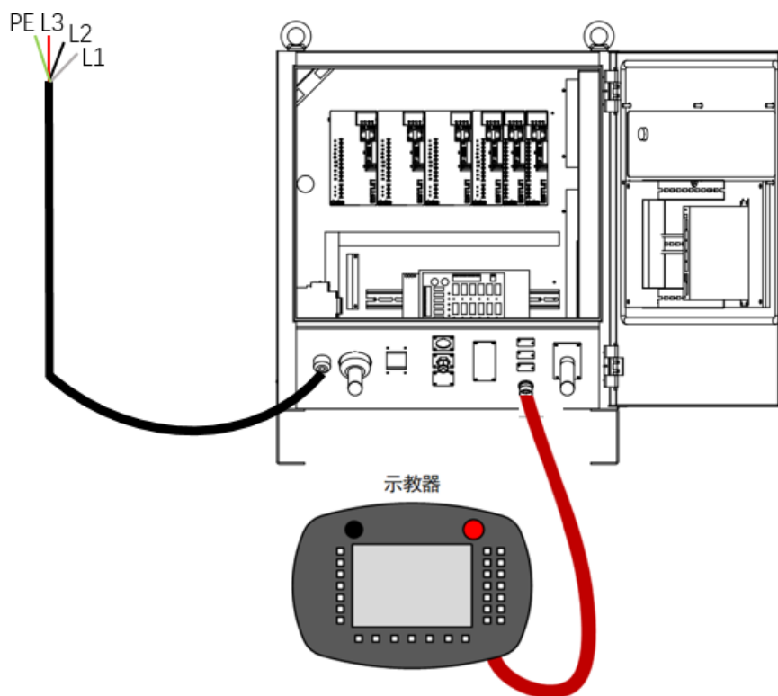
图 3.2 基本示意图
