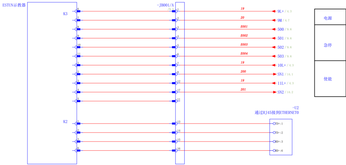
图 3.12 示教器接线
