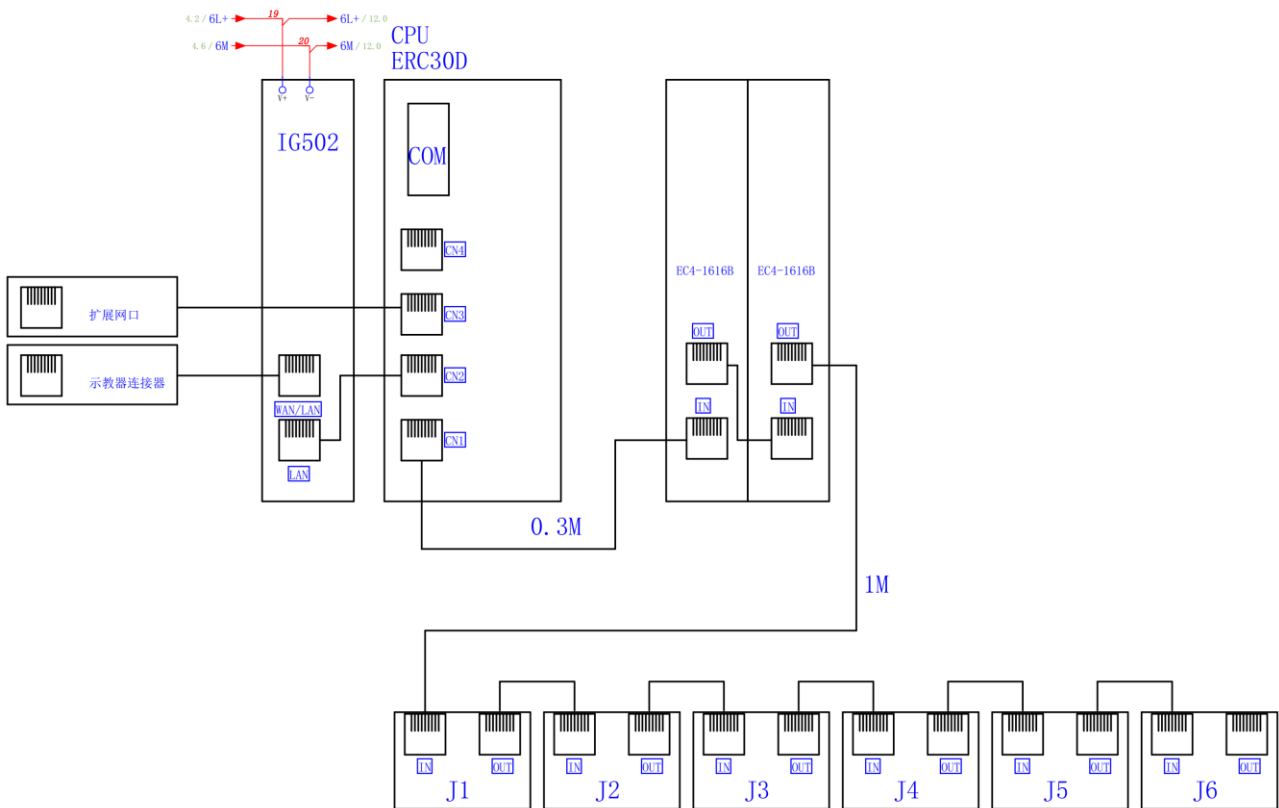
图 3.18 通讯连接图（选配运维精灵）
