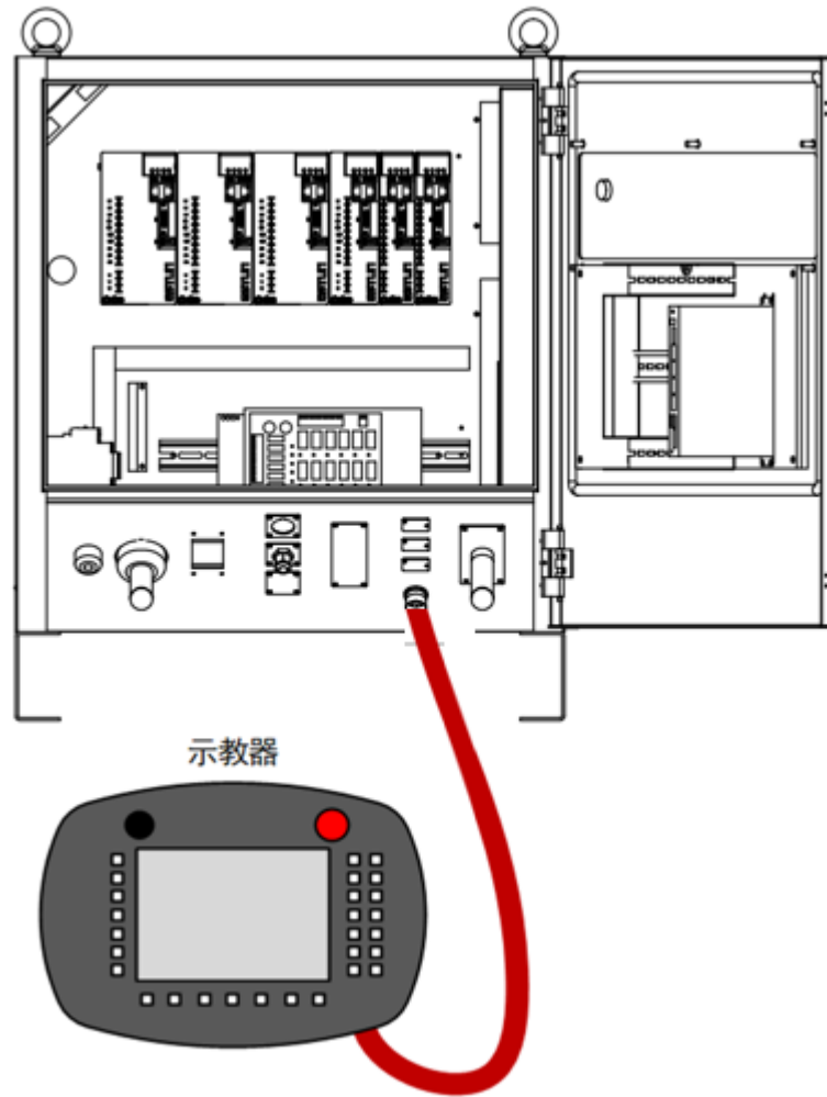
图 3.11 示教器接线
