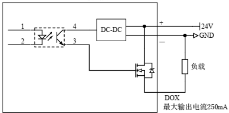
图 3.15 DO PNP 型接线图
