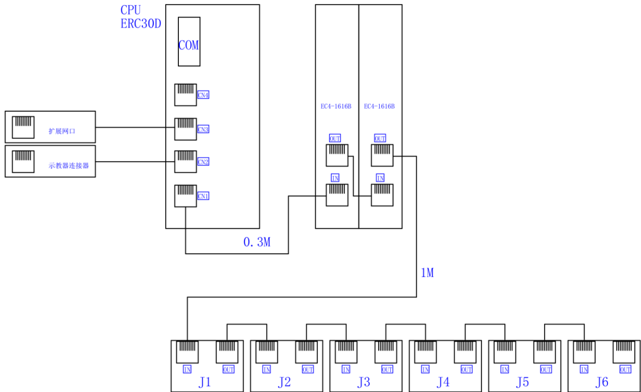
图 3.17 通讯连接图
