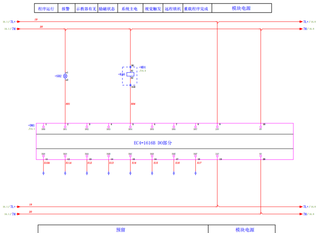
图 3.22 输出模块
