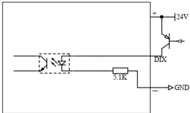
图 3.14 DI PNP 型接线图
