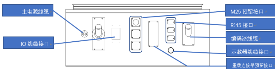
图 1.5 对外接口
