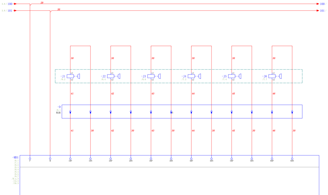
图 3.10 电机抱闸
