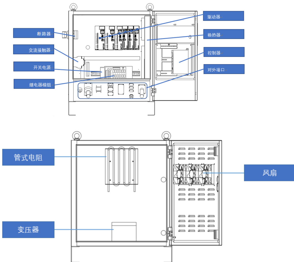
图 1.4 内部结构
