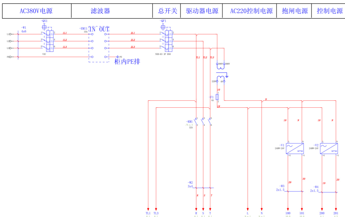
图 3.5 三相电源分配
