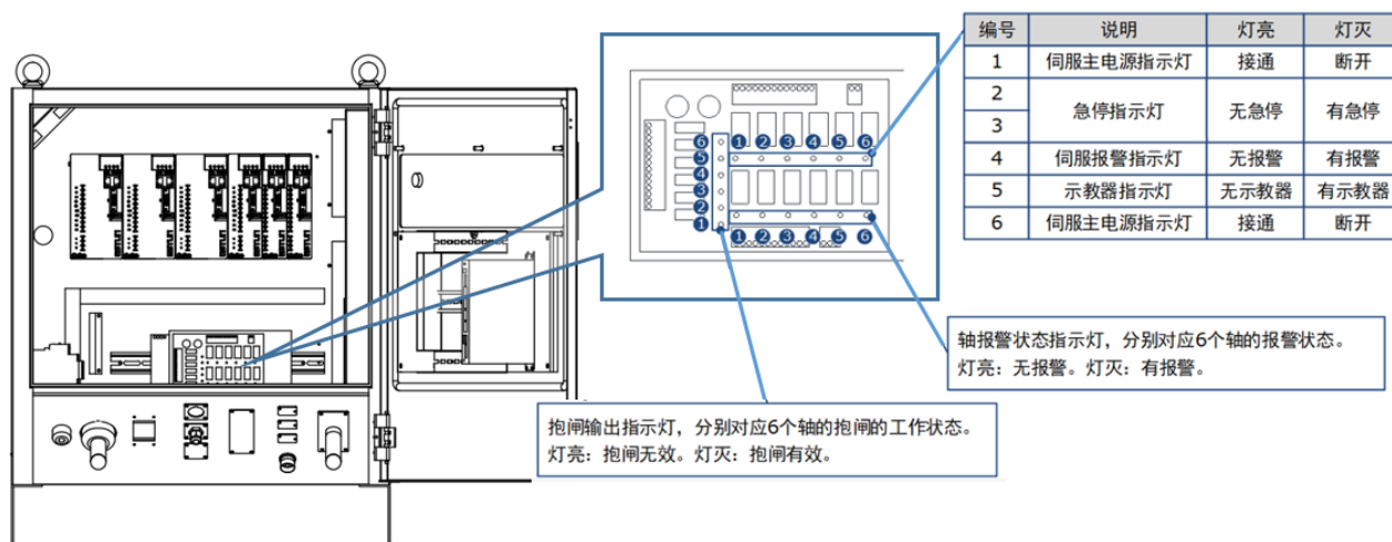
图 3.23 继电器模组指示灯
