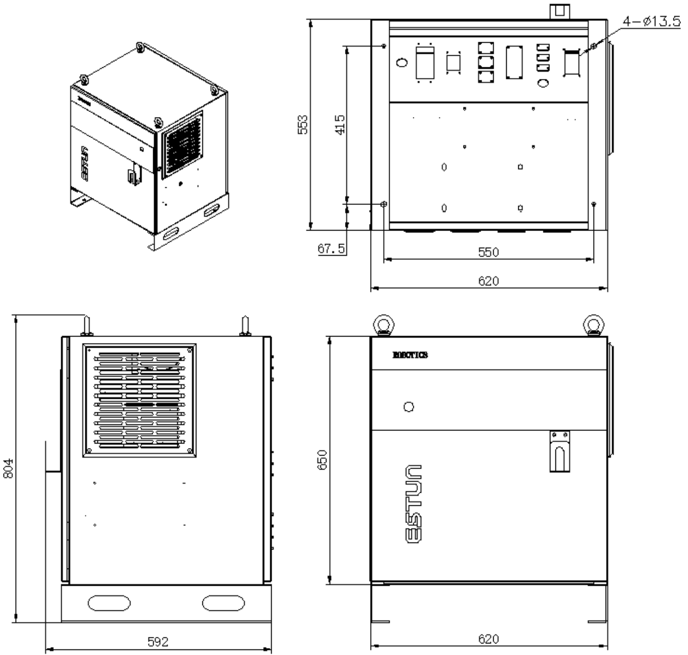
图 2.1 装配尺寸图
