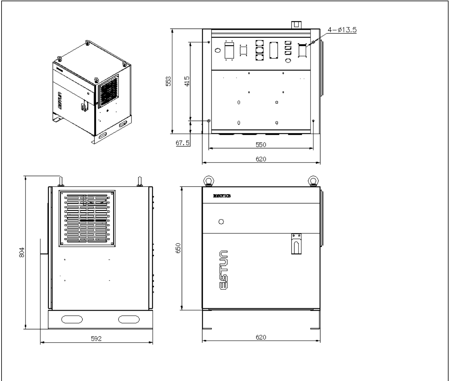
图 1.6 外形尺寸图
