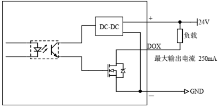
图 3.13 DO NPN 型接线图
