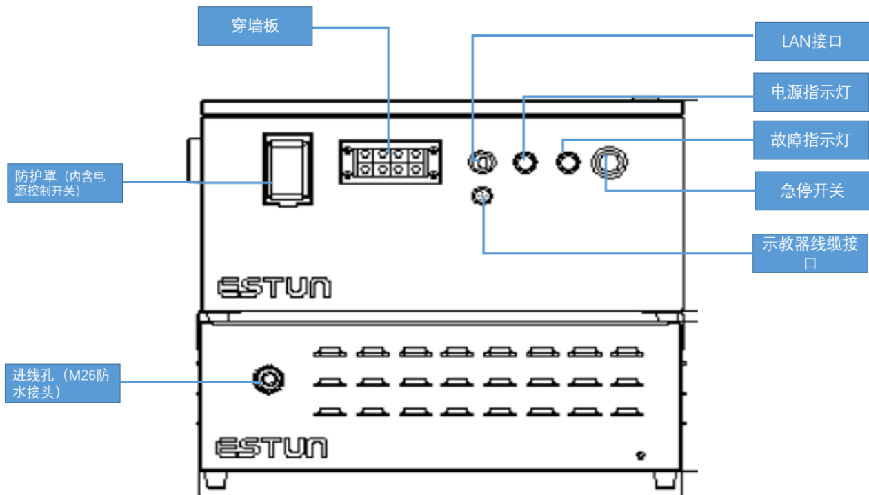
图1-5 对外接口
