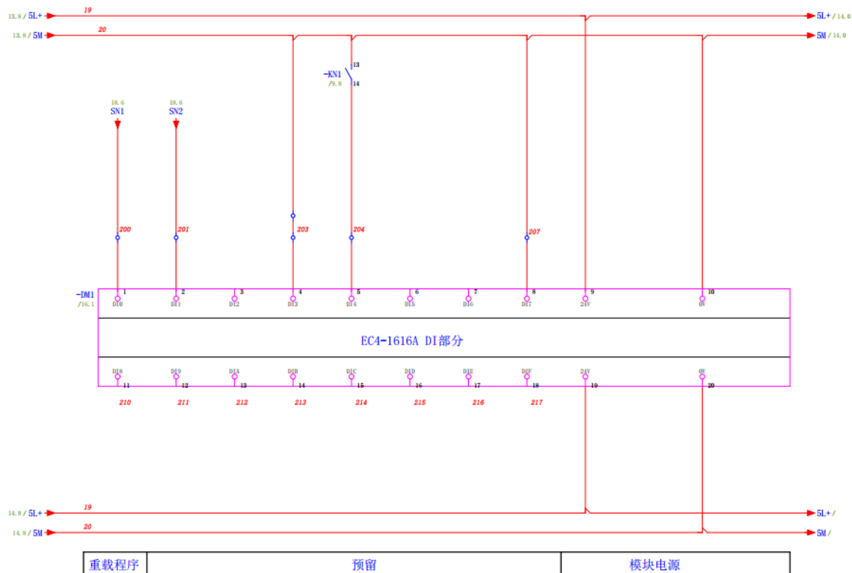
图3-19 输入模块
