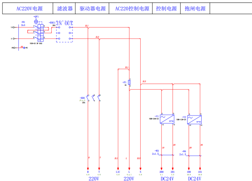
图3-2 单相电源分配 (ED3L-A)
