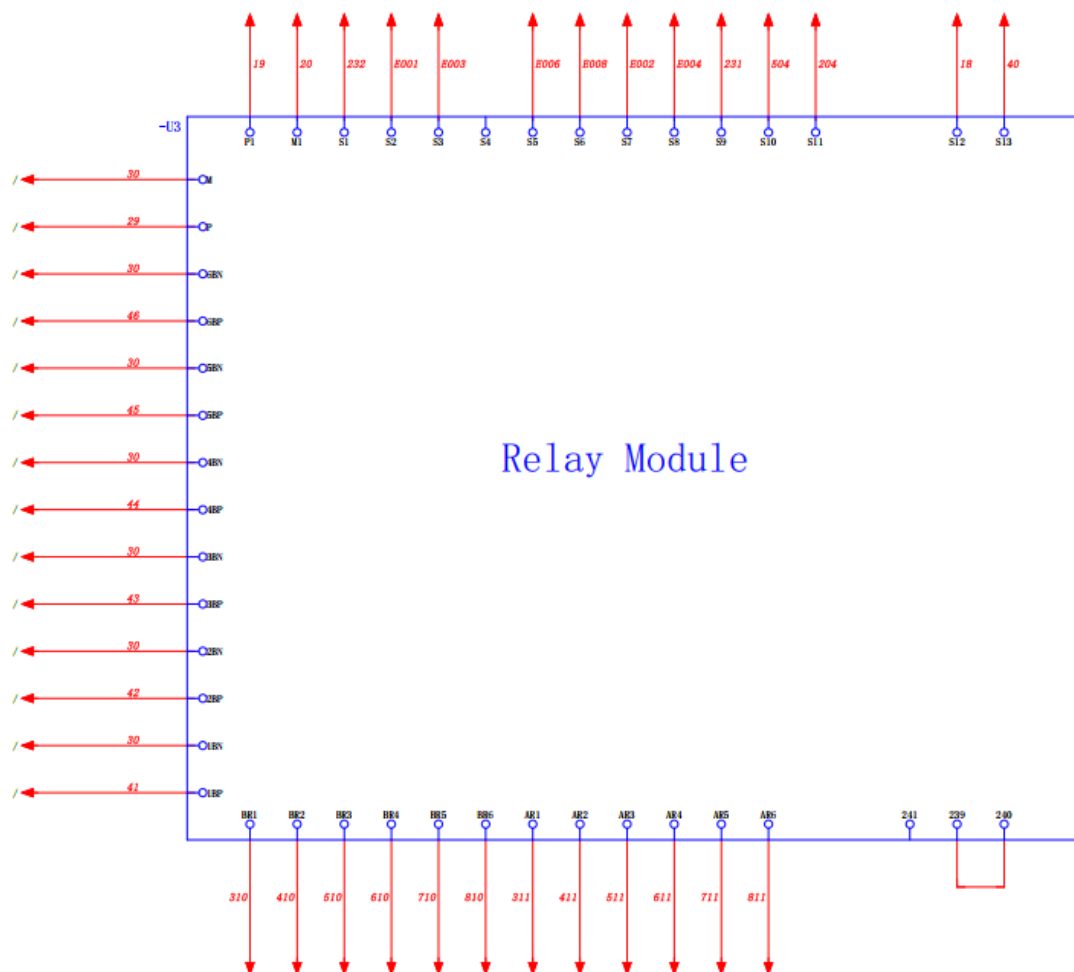
图3-22 继电器模组
