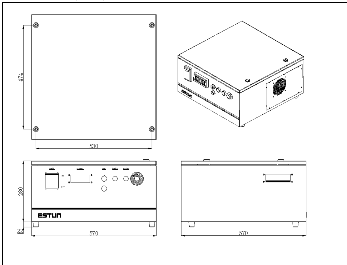
图1-7 ERC-C2-E4SA (ED3L-A) 产品尺寸图
