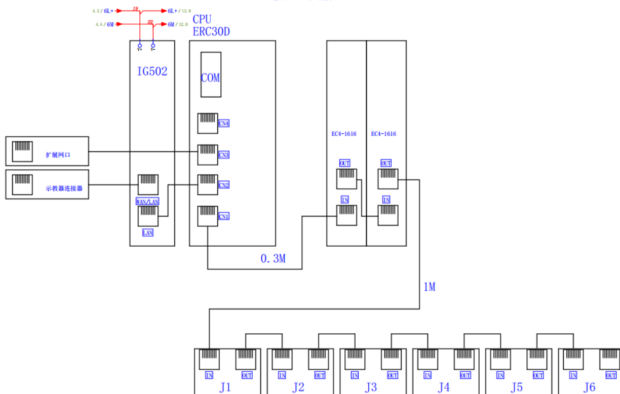
图3-15 通讯连接图（选配运维精灵）
