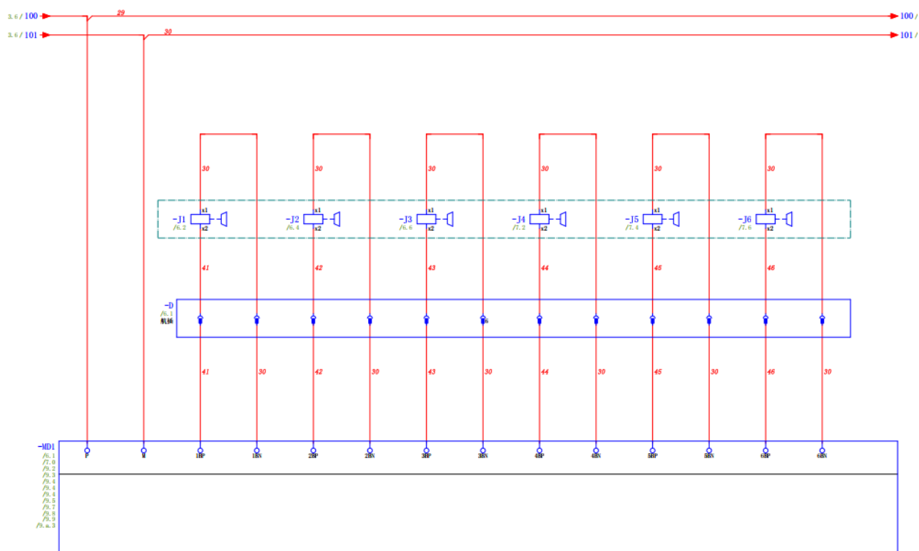
图3-8 电机抱闸
