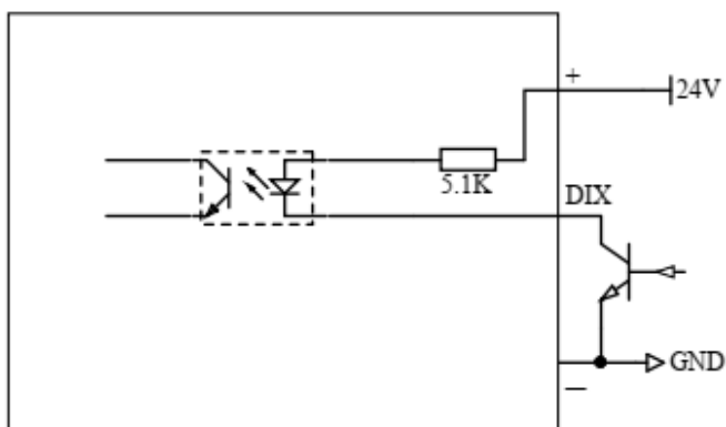
图3-13 DI NPN 型接线图
