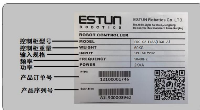
图1-1 ED3L-A 电柜铭牌信息
