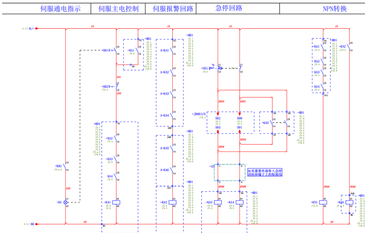
图3-6 DC 24V 控制回路
