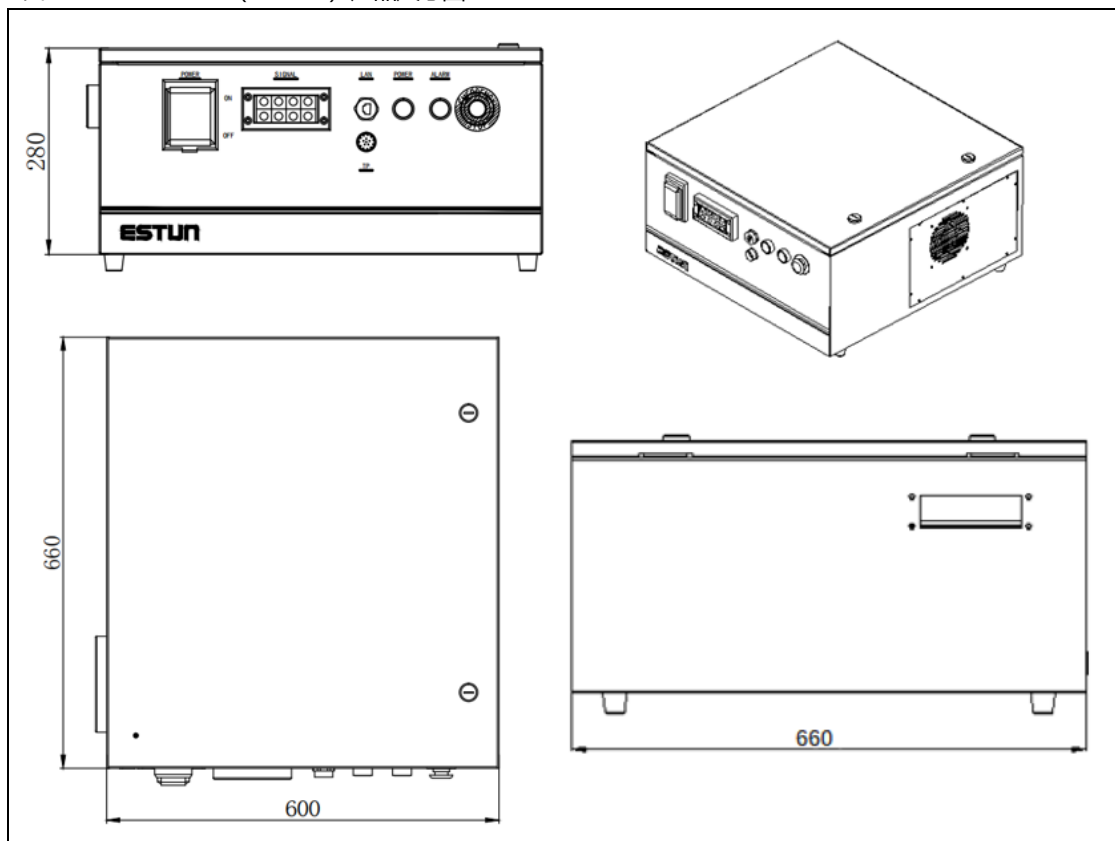
图1-8 ERC-C2-E4SA (ED3L-B) 产品尺寸图
