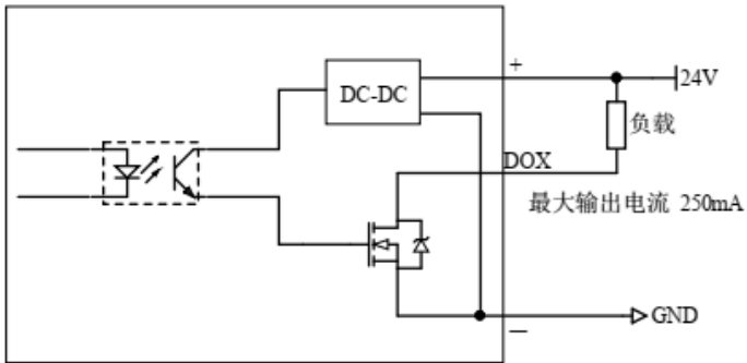
图3-10 DO NPN 型接线图
