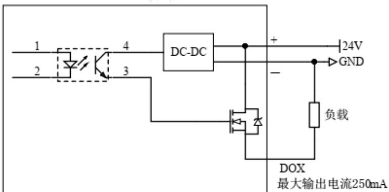
图3-12 DO PNP 型接线图
