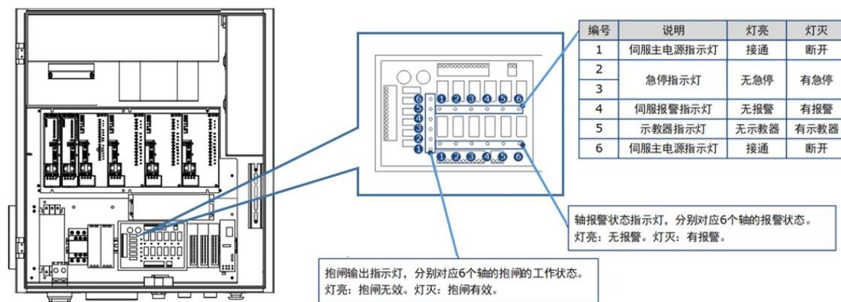
图3-21 继电器模组指示灯
