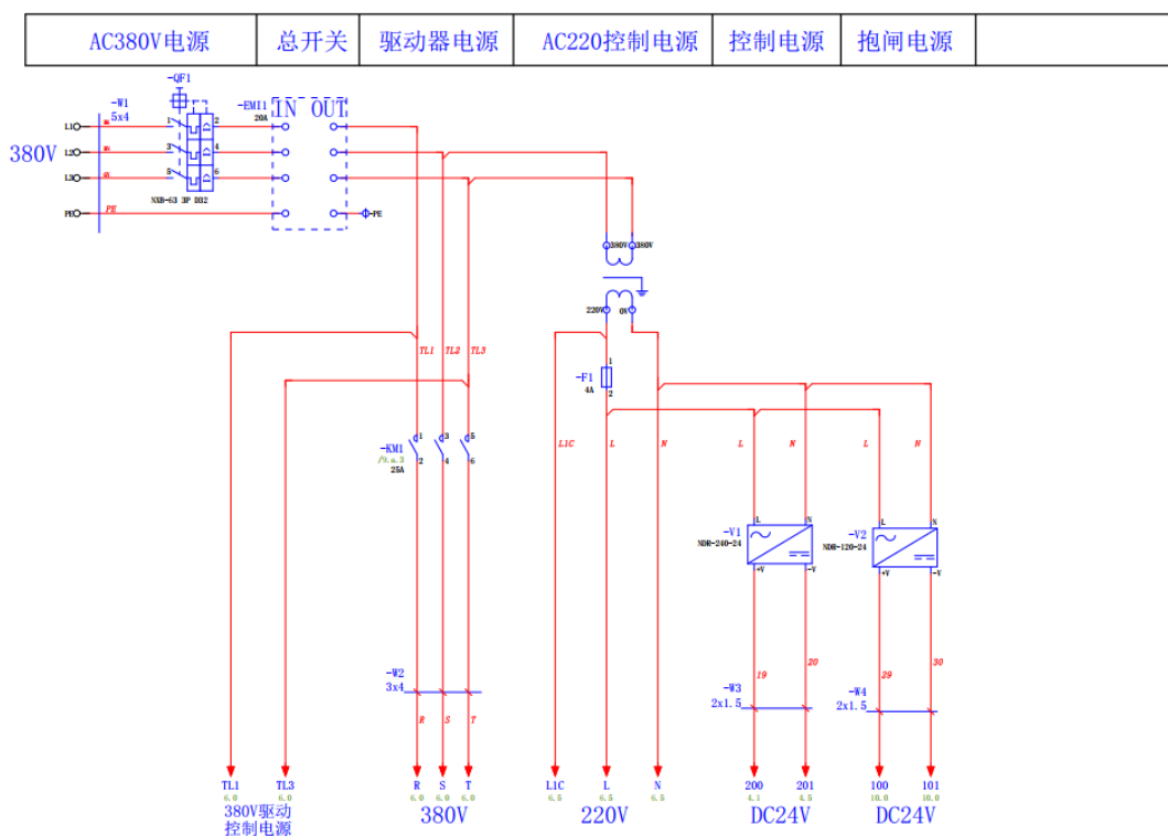
图3-3 三相电源分配 (ED3L-B)
