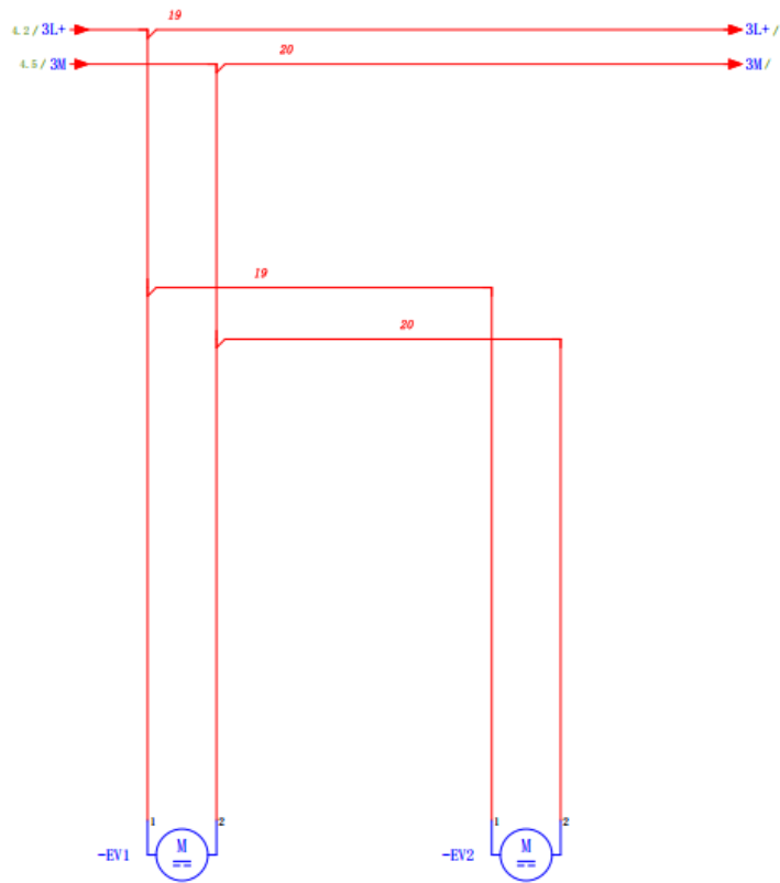
图3-5 散热风机
