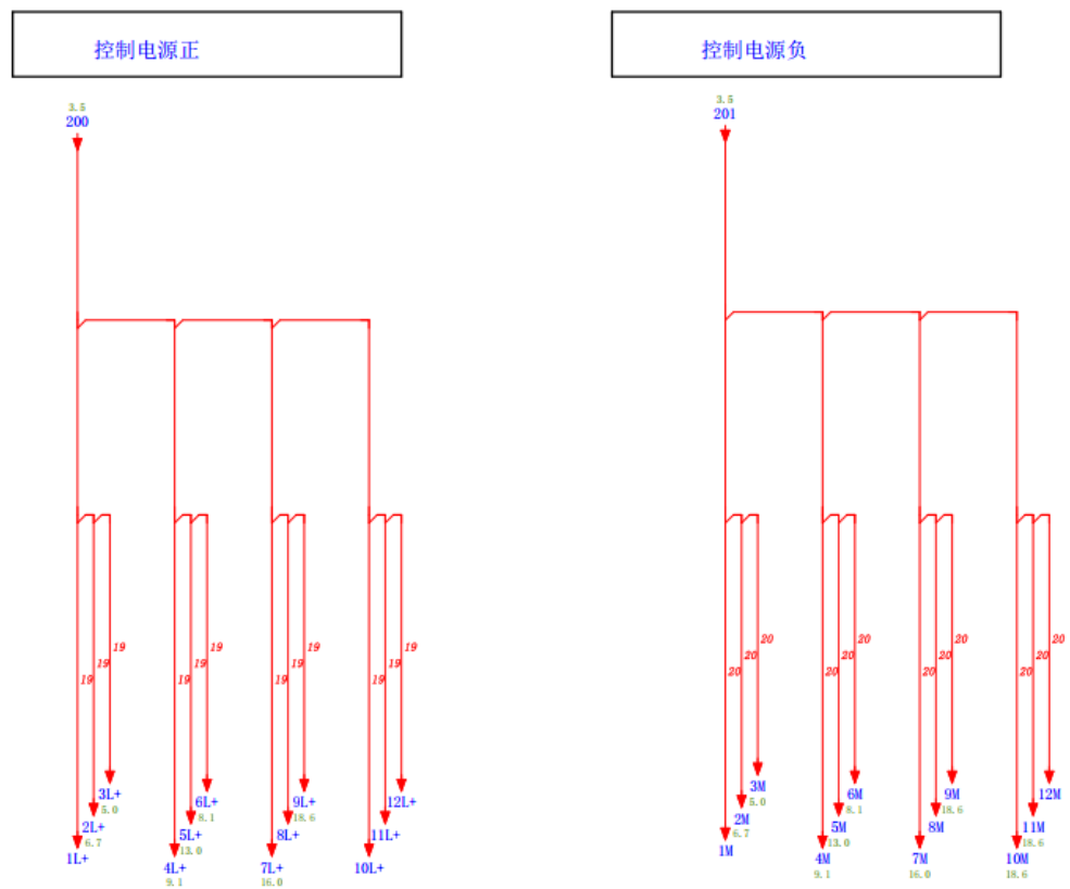
图3-4 控制电源 24V
