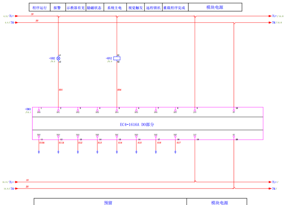
图3-20 输出模块
