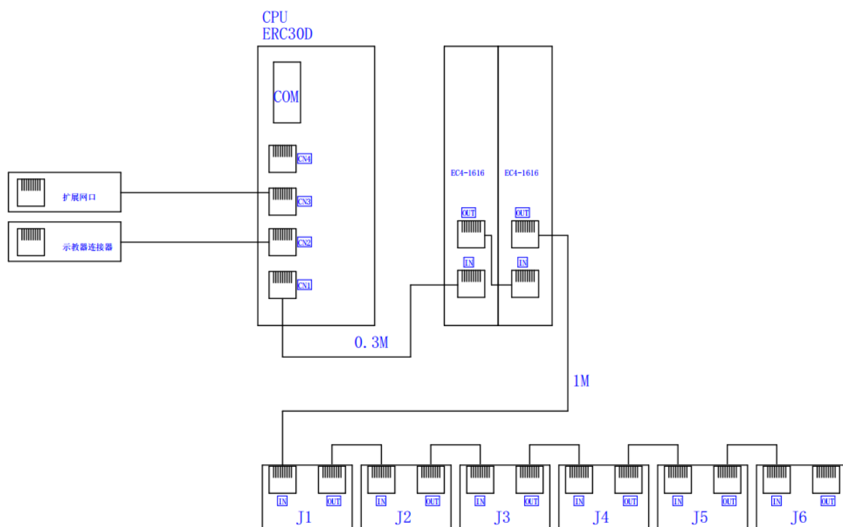
图3-14 通讯连接图
